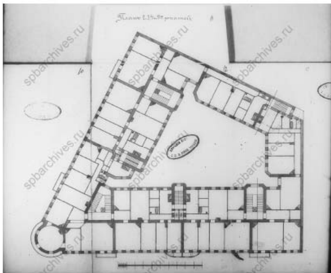
9. План 2, 3, 4 и 5-го этажей. 1908 г. // Источник: ЦНИИ СПб Ф. 513 Оп. 102 Д. 9551 Л. 10-13.
