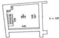
План антресоли
