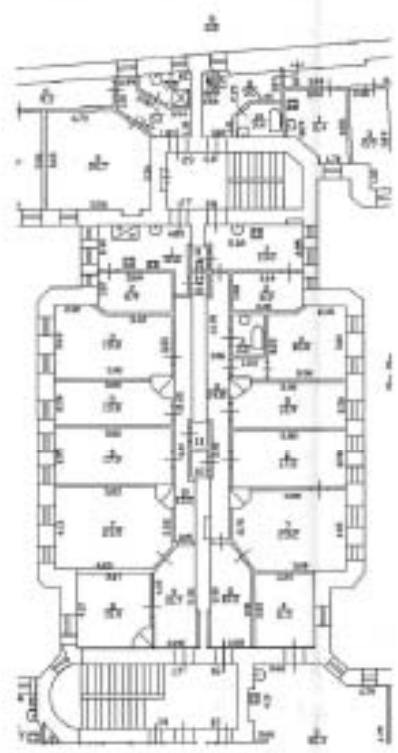
План части 4-го этажа
