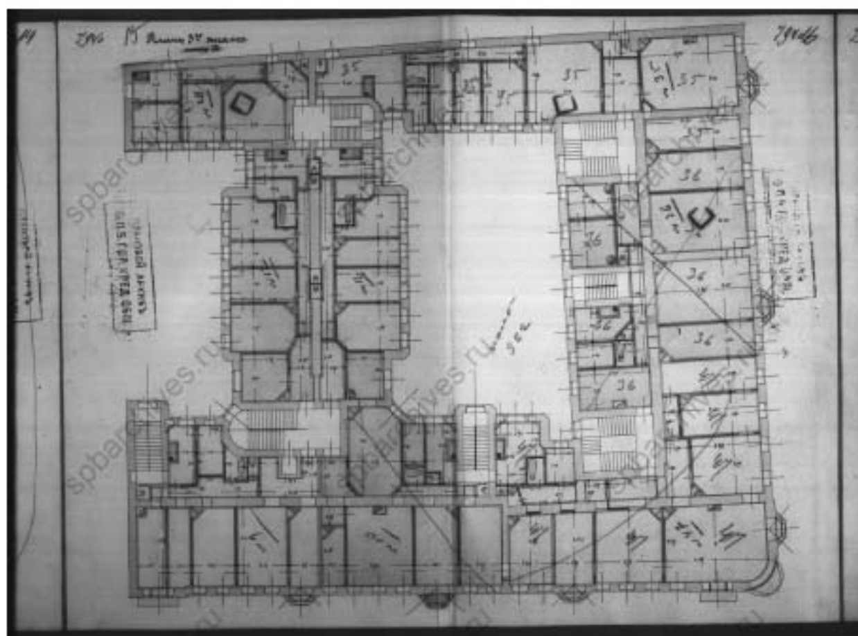
12. План третьего этажа. Чертежи дома В.В.Змеёва, И.И.Круглова по Невскому пр.,147. ЦГИА СПб. Фонд 515. Опись 4. Дело 3953. 15.11.1896–18.07.1915;
