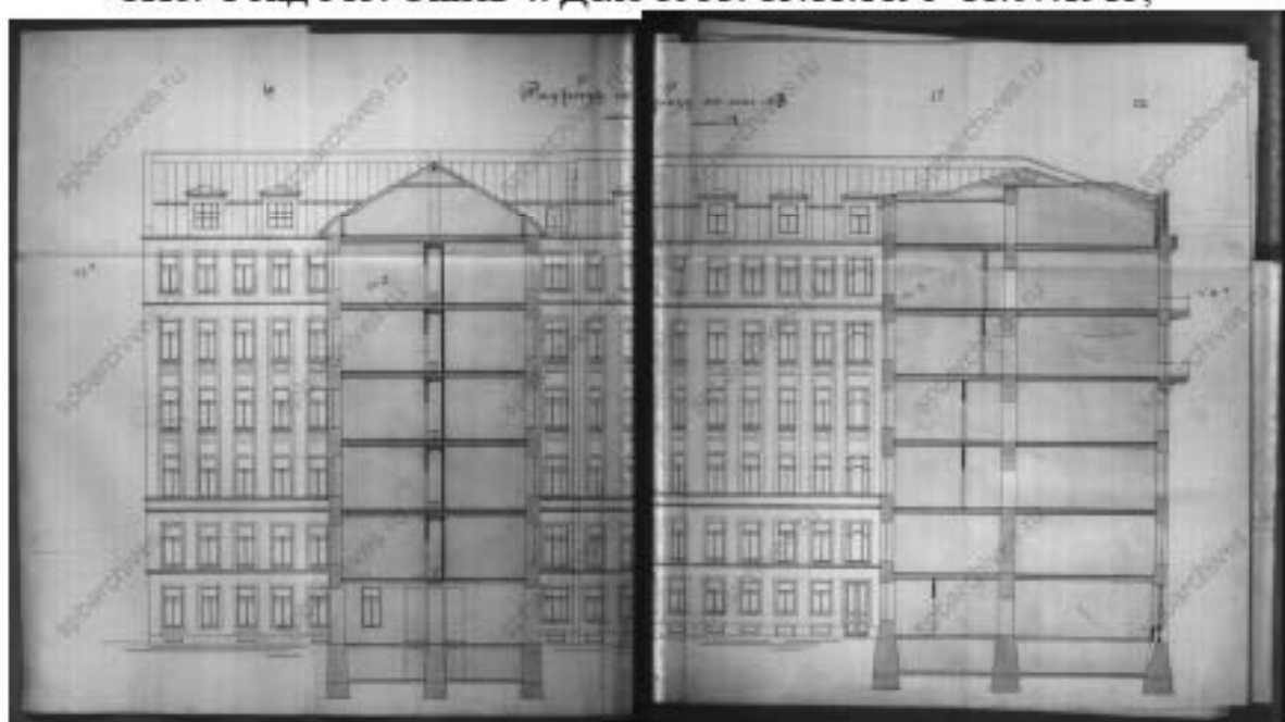
23. Разрез по линии № 8. Дворовой фасад. Чертежи дома В.В.Змеева, И.И.Круглова по Невскому пр., 147. ЦГИА СПб. Фонд 515. Описание 4. Дело 3953. 15.11.1896–18.07.1915;
