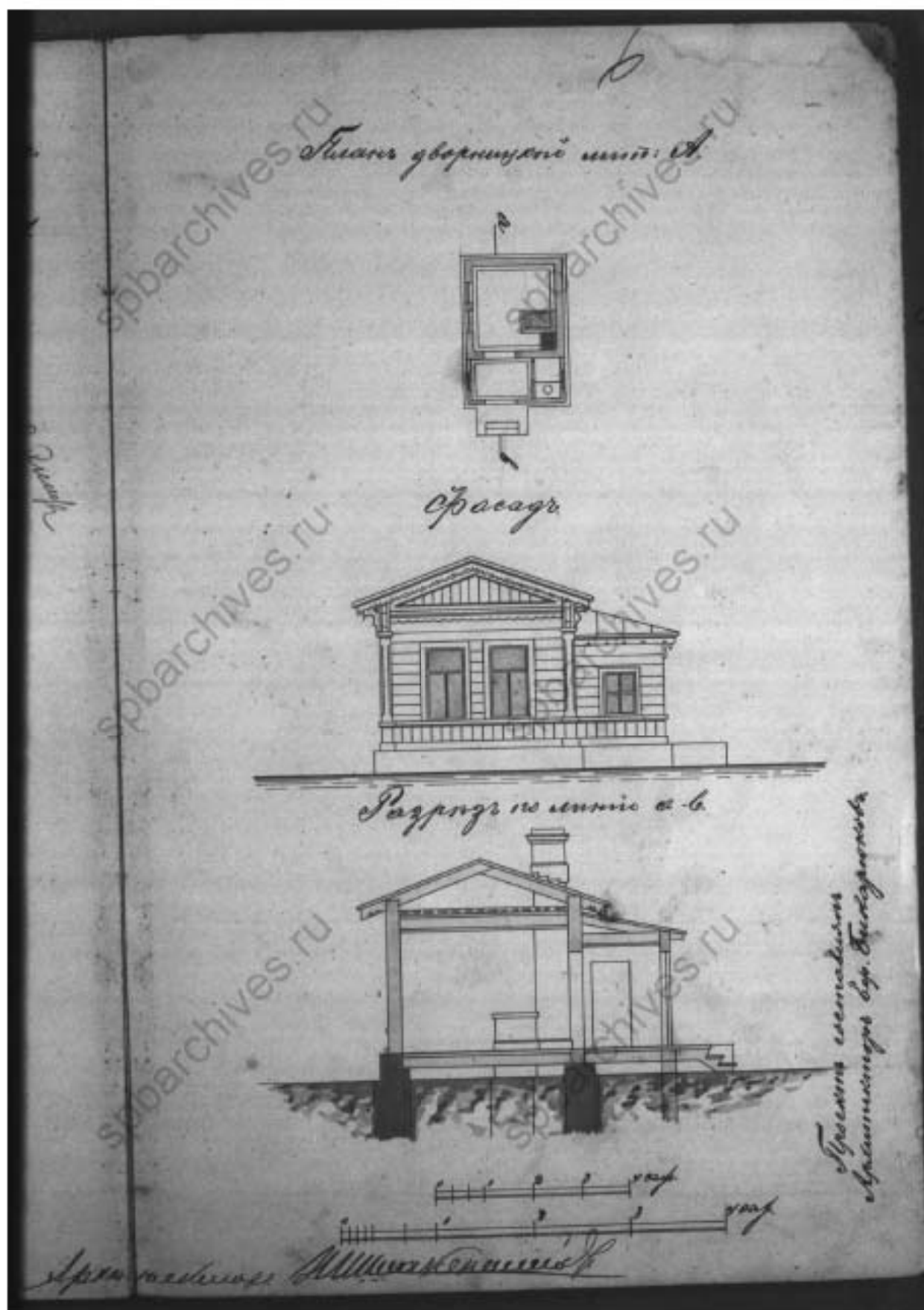
7. Фасад. Чертежи дома В.В.Змеева, И.И.Крутлова по Невскому пр.,147. ЦГИА СПб. Фонд 515. Описание 4. Дело 3953. 15.11.1896–18.07.1915;
