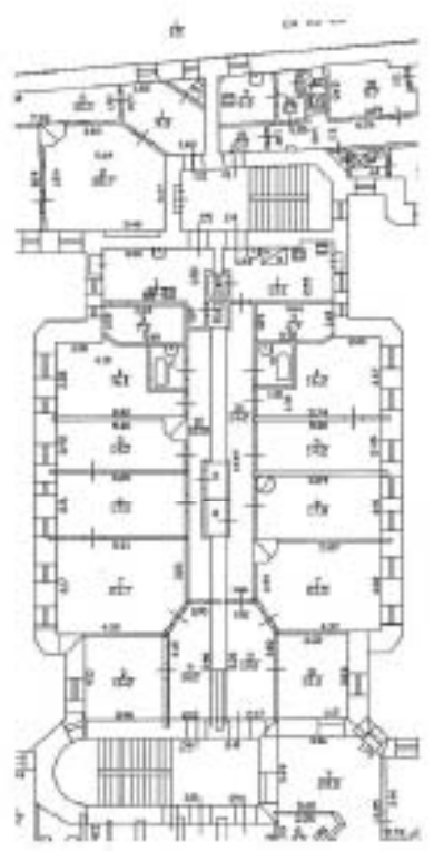
План части 6-го этажа
