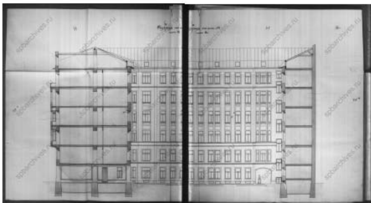
22. Разрез по линии № 4. Дворовой фасад. Чертежи дома В.В.Змеева, И.И.Круглова по Невскому пр., 147. ЦГИА СПб. Фонд 515. Описание 4. Дело 3953. 15.11.1896–18.07.1915;
