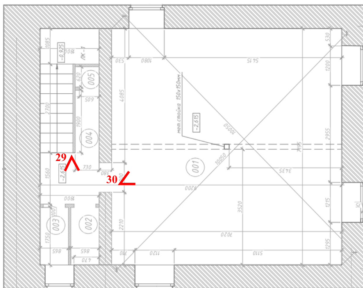
Подвал
