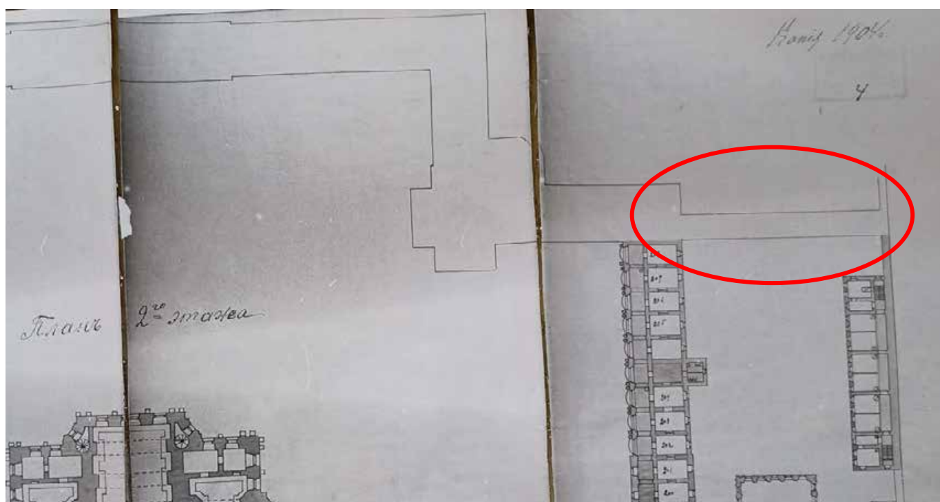
13. План 2-го этажа СПб Вдовьего дома (фрагмент). Архив КГИОП, коллекция фотографий.
