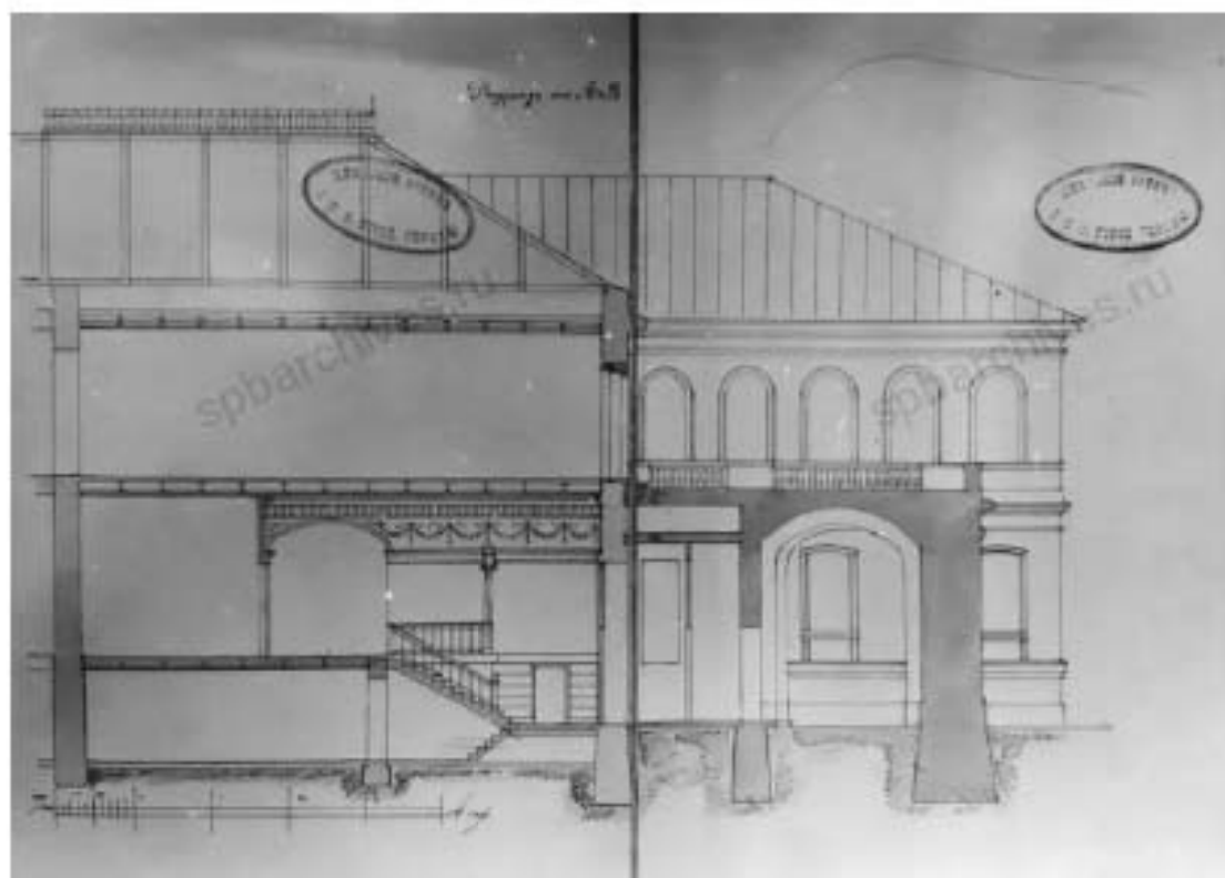
7. «Корпус служебный», входящий в состав объекта культурного наследия федерального значения «Дом Горчакова К.А.» (Большая Монетная ул., д. 17-19, лит. Г). Дом А.С.Слепшовой. Фасад на Большую Монетную ул. Проект 1893 г. Инженер Н.А.Архангельский. ЦГАНТД СПб Ф.488. Оп. 3-13. Д. 56. Историческая справка 1991 г.
