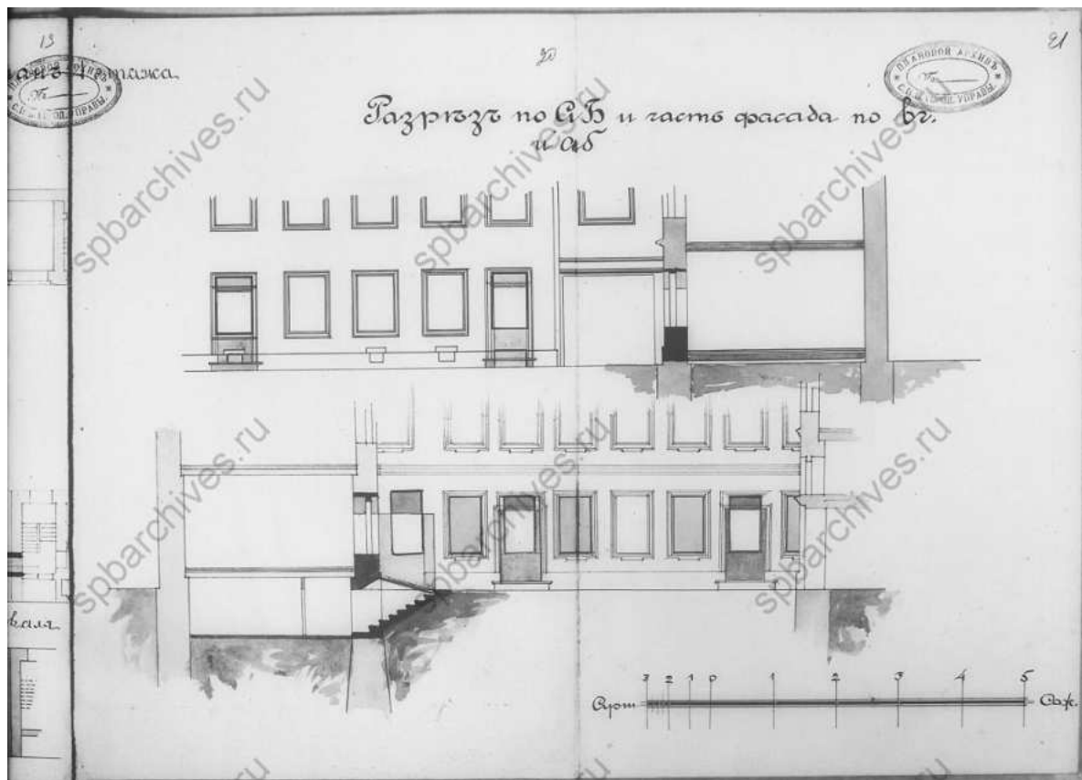
39. Разрез по линии АБ и часть фасада по динии вг. ЦГИА СПб. Фонд 513. Опись 102. Дело 9947
