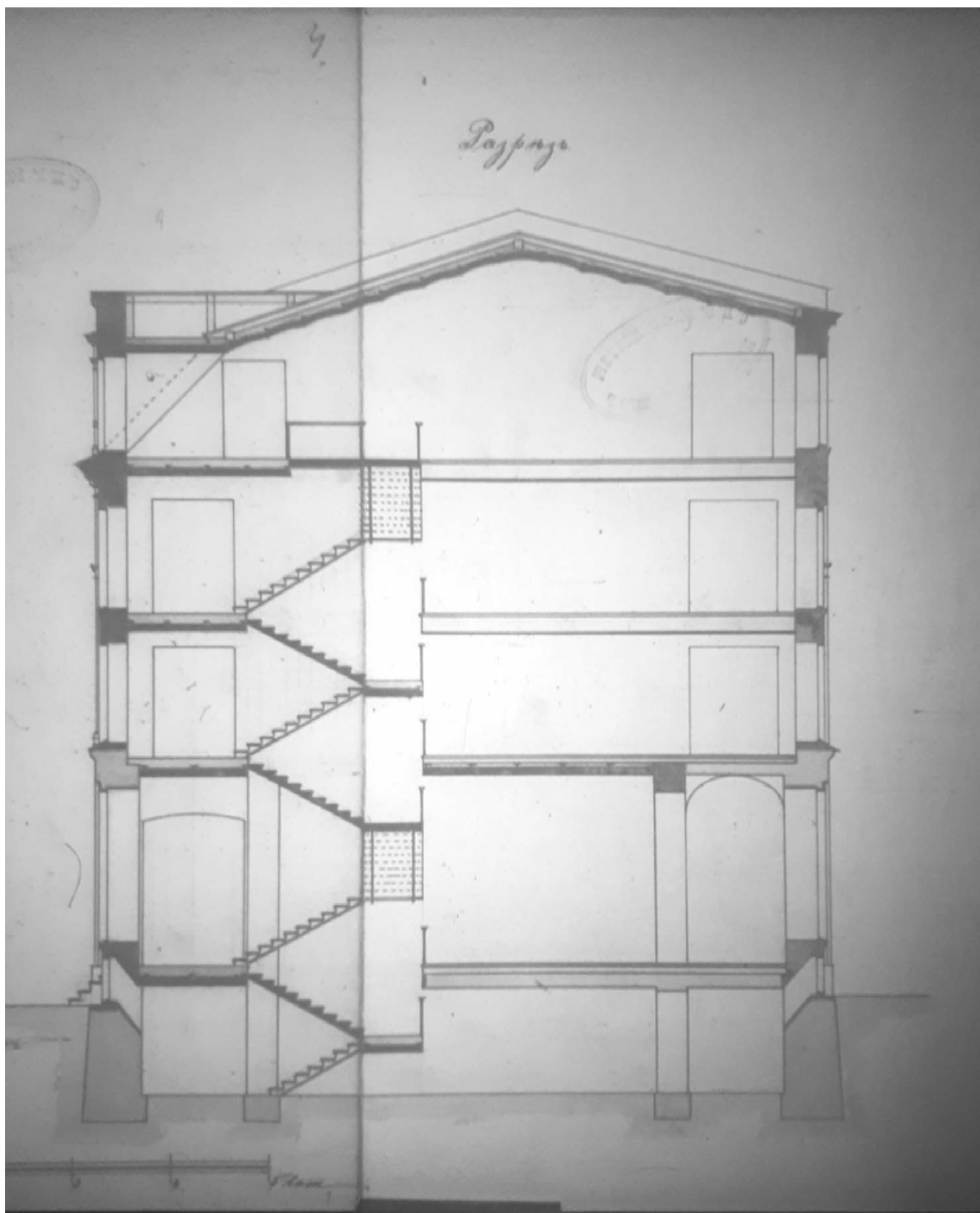
13. Разрез. Лавка купца Михаила Александровича Александрова. 1897 г. // Источник: ЦГИА СПб Ф.513 Оп.115 Д.697 Л.4-5.
