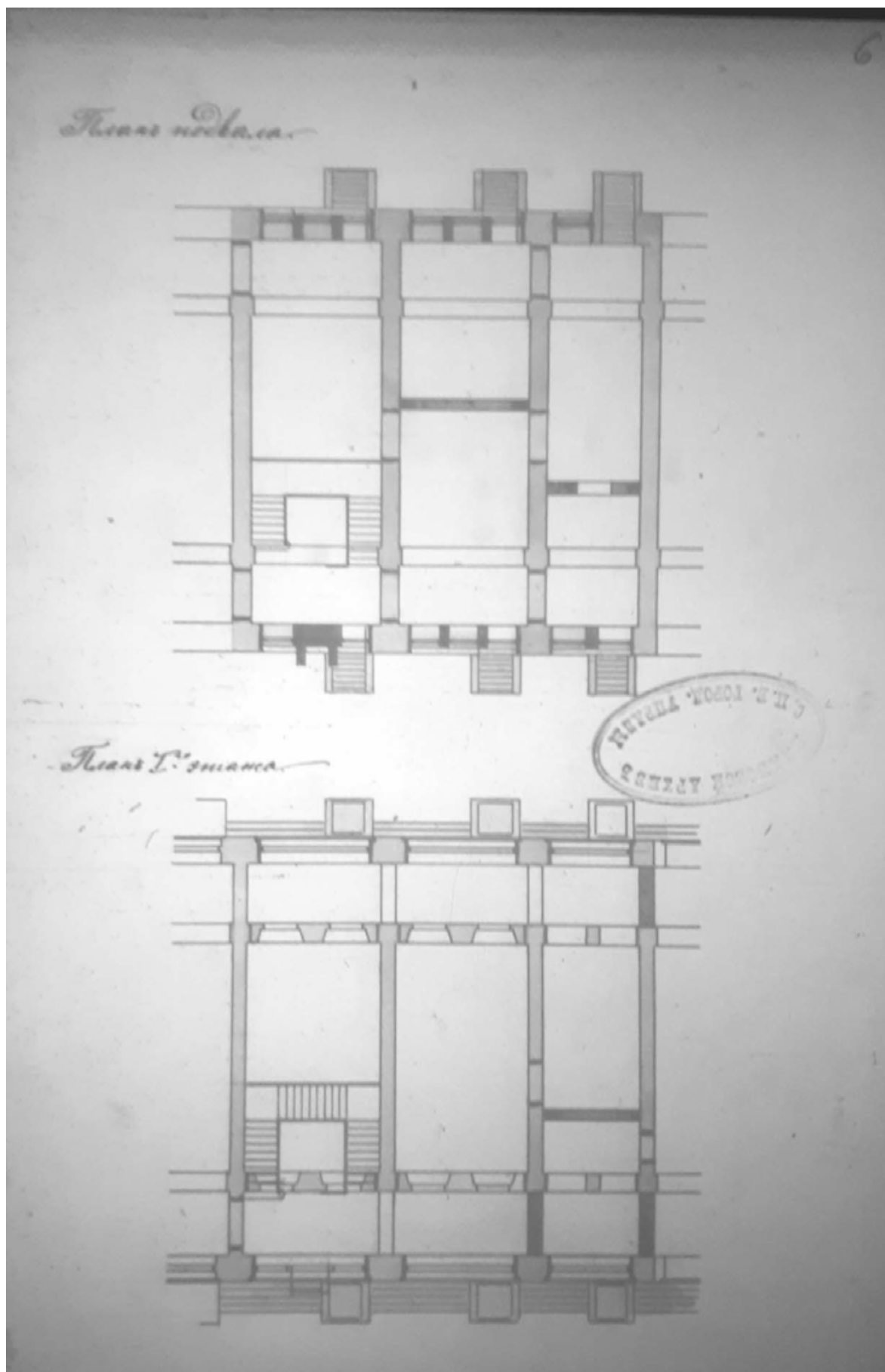
14. Планы подвала и 1-го этажа лавок купца Михаила Александровича Александра. 1897 г. // Источник: ЦГИА СПб Ф.513 Оп.115 Д.697 Л.6.
