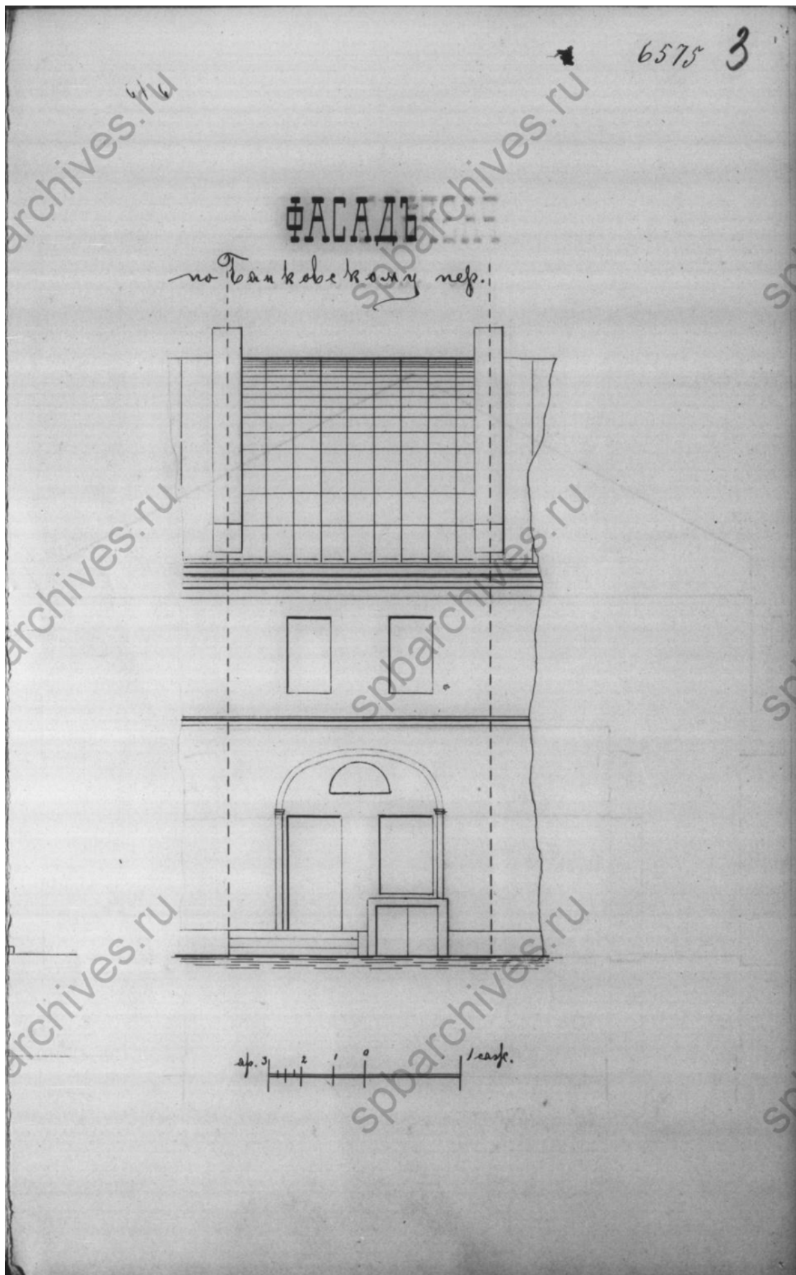
7. Чертежи лавки совладельцев Оприц по Банковскому пер.,3. Фасад по Банковскому переулку. 1844 г. // Источник: ЦГИА СПб Ф.515 Оп.4 Д.119. Л.3.
