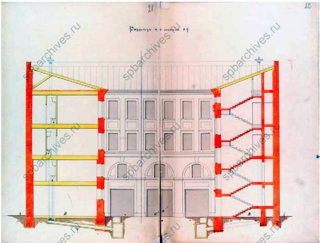
Илл. 23. Разрез по линии EF. 1873 г. ЦГИА СПб. Ф. 513. Оп. 102. Д. 171. Л. 21-22.
