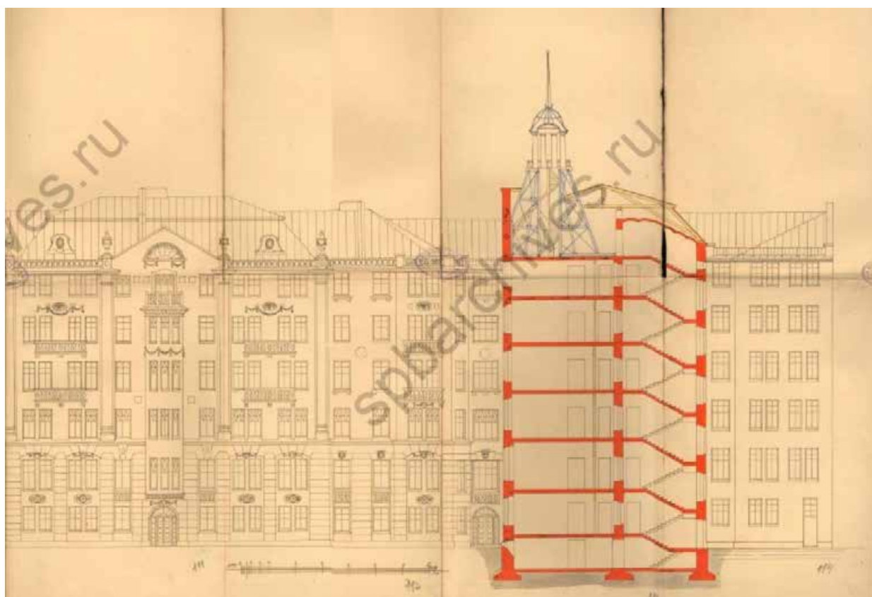
Илл. 21. Разрез по линии А-Б. 1911 г. ЦГИА СПб. Ф. 513. Оп. 102. Д. 5300. Л. 111-114.
