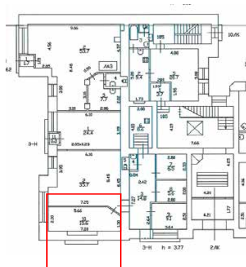
Рис. 3 – План части первого этажа (по состоянию на 14.08.2023 г.). Оконный проем в осях «А/2-3».
