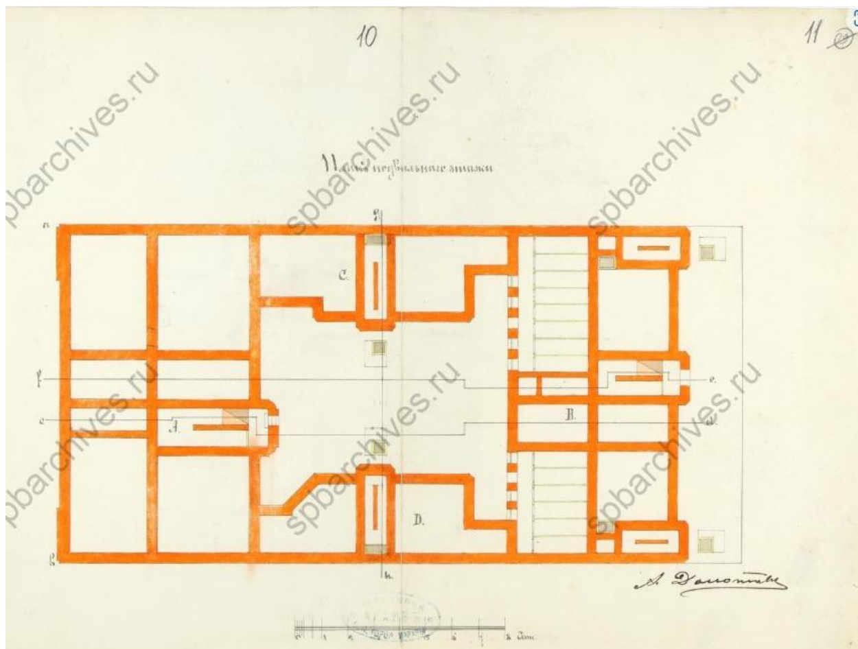
Илл. 13. Фасад дома по Эргелеву переулку под № 11. План подвального этажа. А. Долотов. 1876. ЦГИА СПб. Ф. 513. Оп. 102. Д. 4587. Л. 10-11.
