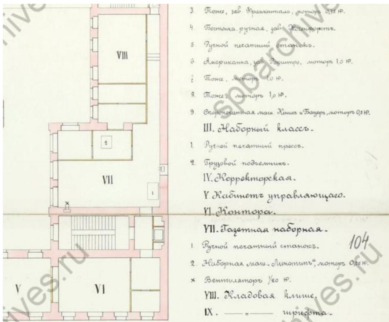
Илл. 44. План двора г-ва А.С. Суворина «Новое время», по Эртелеву пер. № 13. Экспликация помещений типографии. 2-й этаж. Фрагмент. 1915 г. ЦГИА СПб. Ф. 513. Оп. 102. Д. 4589. Л. 103-104.
