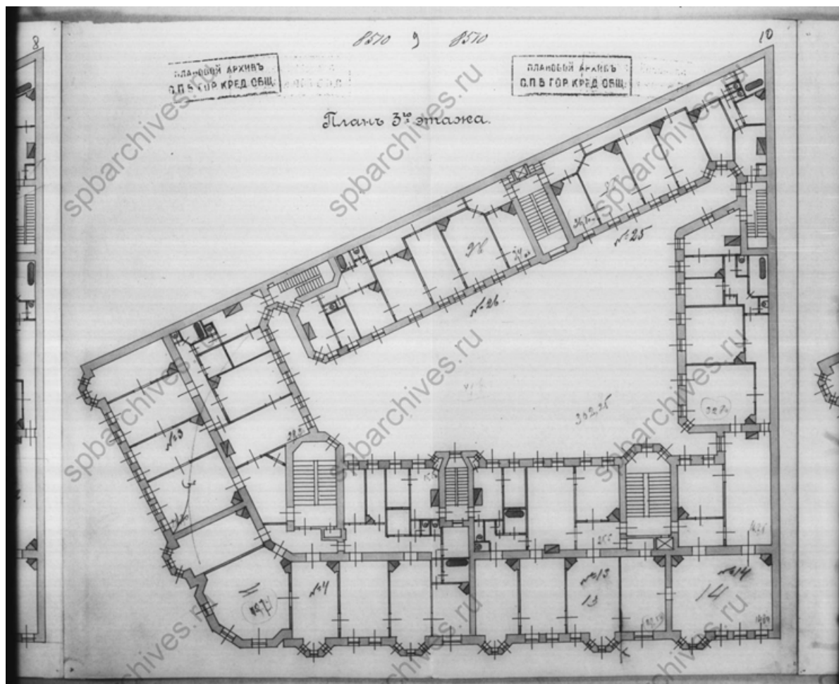
10. План 3-го этажа. Чертежи дома В.Г. и О.М.Чубаковых по Большому пр.П.С., 96 и Каменноостровскому пр., 38. ЦГИА СПб. Фонд 515. Опись 4. Дело 2484. 08.02.1912 г.
