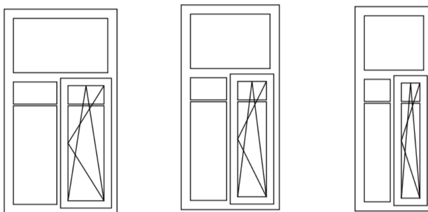
Рис. 2. Проектируемые оконные заполнения дворового фасада.
