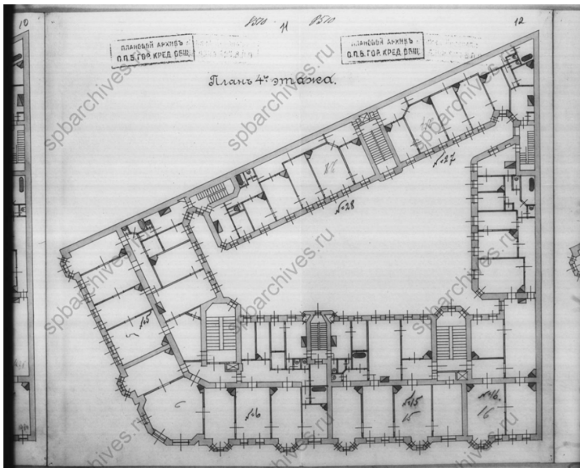
11. План 4-го этажа. Чертежи дома В.Г. и О.М.Чубаковых по Большому пр.П.С., 96 и Каменноостровскому пр., 38. ЦГИА СПб. Фонд 515. Опись 4. Дело 2484. 08.02.1912 г.
