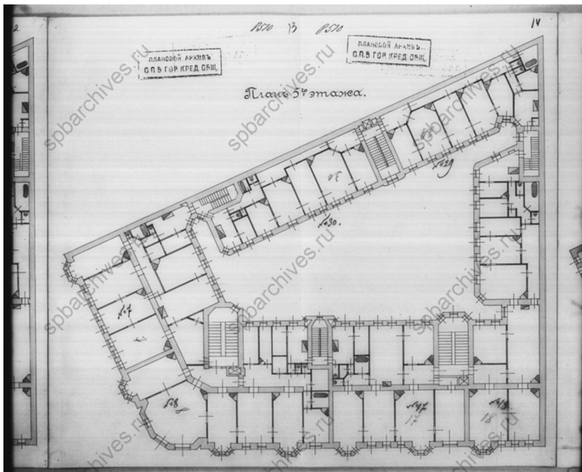
12. План 5-го этажа. Чертежи дома В.Г. и О.М.Чубаковых по Большому пр.П.С., 96 и Каменноостровскому пр., 38. ЦГИА СПб. Фонд 515. Опись 4. Дело 2484. 08.02.1912 г.
