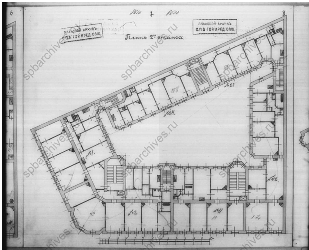
9. План 2-го этажа. Чертежи дома В.Г. и О.М.Чубаковых по Большому пр.П.С., 96 и Каменноостровскому пр., 38. ЦГИА СПб. Фонд 515. Опись 4. Дело 2484. 08.02.1912 г.
