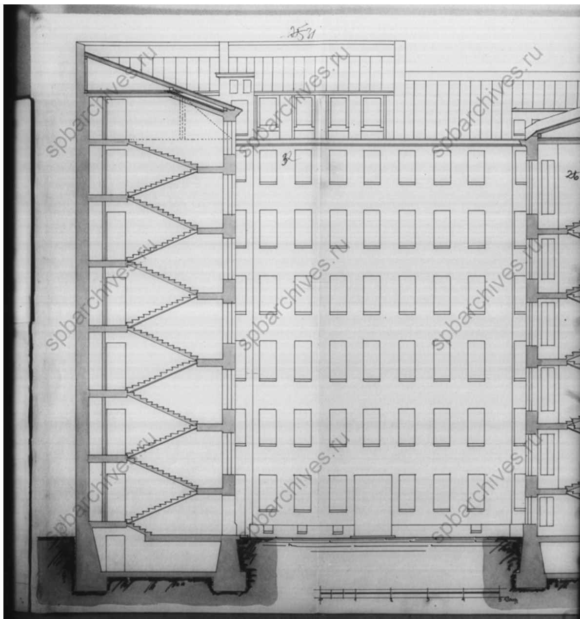
18. Разрез. Чертежи дома В.Г. и О.М.Чубаковых по Большому пр.П.С., 96 и Каменноостровскому пр., 38. ЦГИА СПб. Фонд 515. Опись 4. Дело 2484. 08.02.1912 г.
