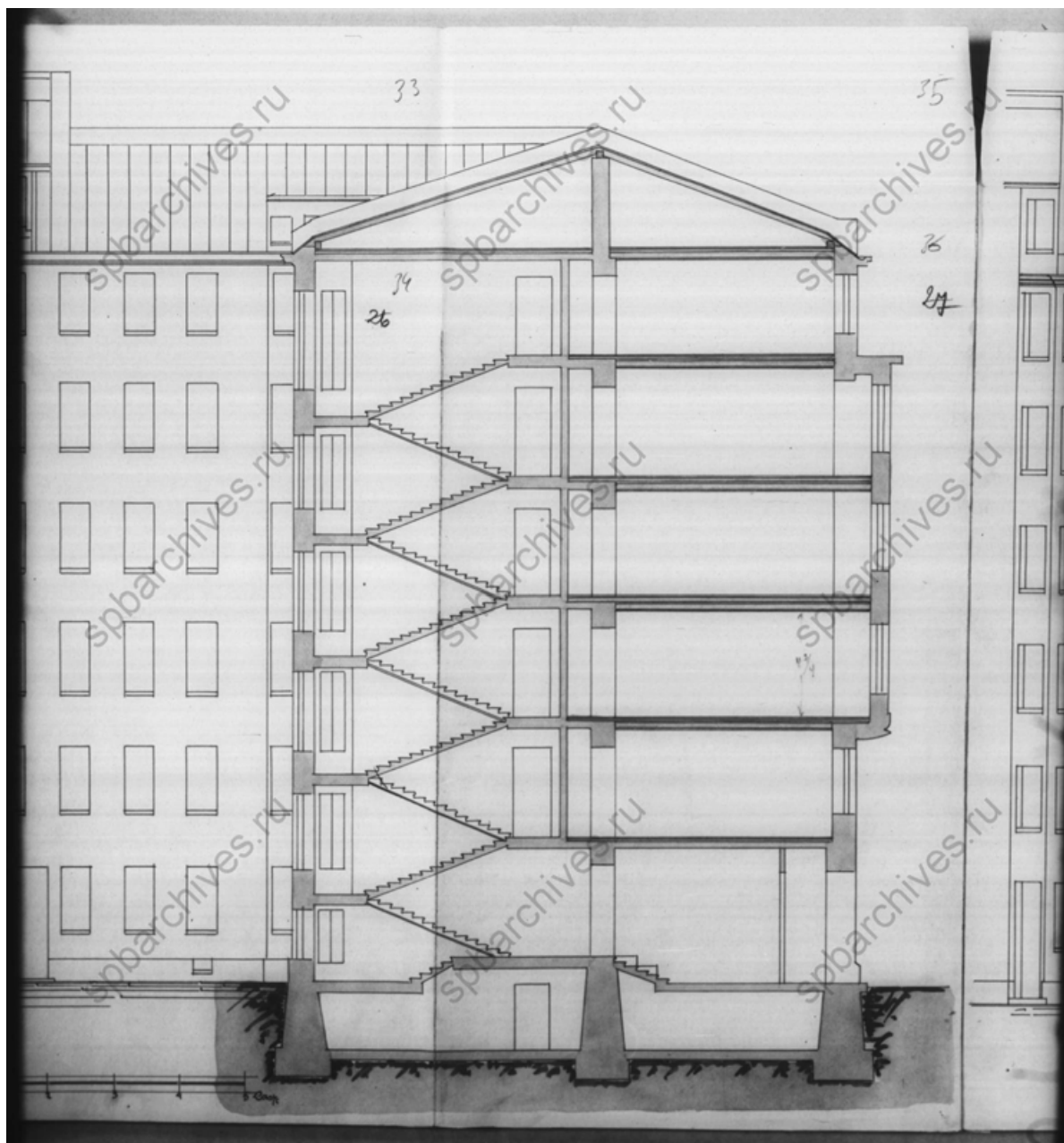
19. Разрез. Чертежи дома В.Г. и О.М.Чубаковых по Большому пр.П.С., 96 и Каменноостровскому пр., 38. ЦГИА СПб. Фонд 515. Опись 4. Дело 2484. 08.02.1912 г.
