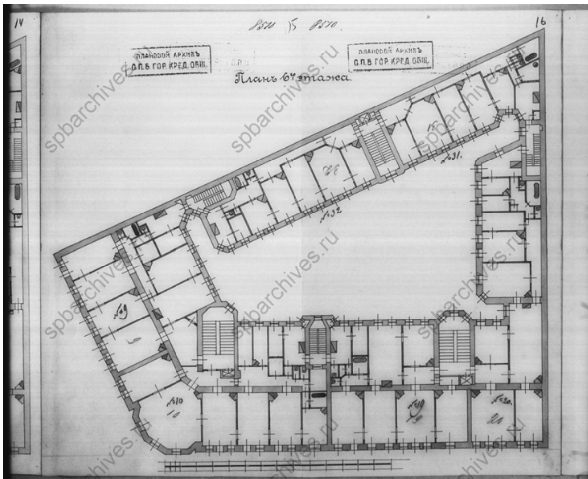
13. План 6-го этажа. Чертежи дома В.Г. и О.М.Чубаковых по Большому пр.П.С., 96 и Каменноостровскому пр., 38. ЦГИА СПб. Фонд 515. Опись 4. Дело 2484. 08.02.1912 г.
