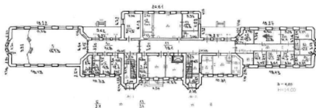
План 1 этажа
