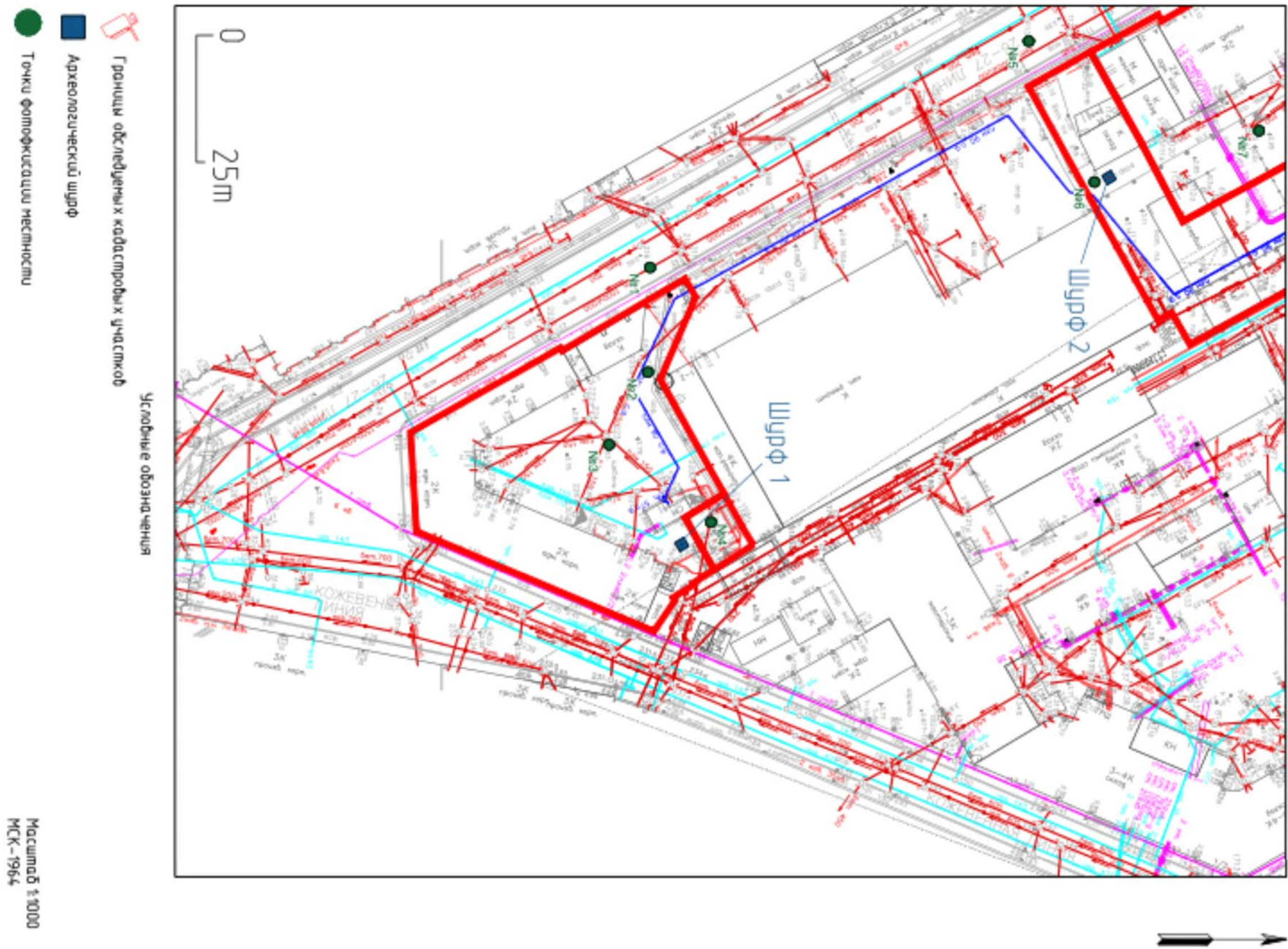
Рис. 12. СПб-2025. Василеостровский р-н. 26-я линия, д. 1-3. Топографический план обследуемой территории. Масштаб 1:500
