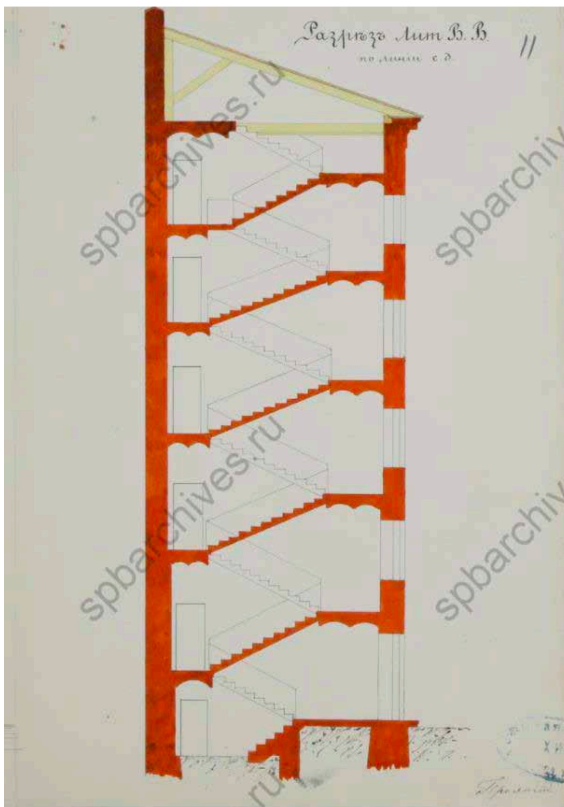
9. Разрез Лит. ВВ по линии сд. ЦГИА СПб. Ф. 513. Оп. 102. Д. 4580. Л. 11.
