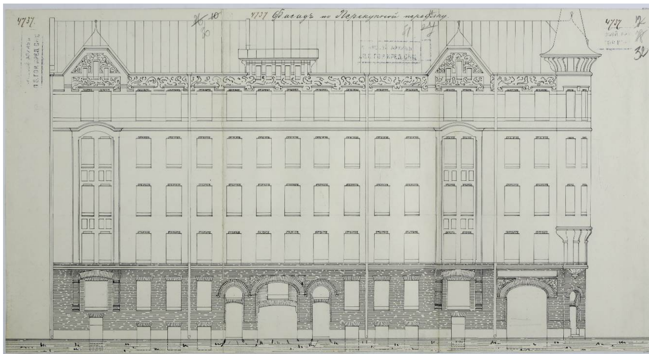
13. Фасад по Перекупному переулку. Л.30-32. ЦГИА СПб. Фонд 515. Опись 4. Дело 5724. Чертежи дома А.П.Шерстобитова, П.В. Клименко, К.К. Шмидта по Херсонской ул.,13 и Перекупному пер.,12. (1862–1916)
