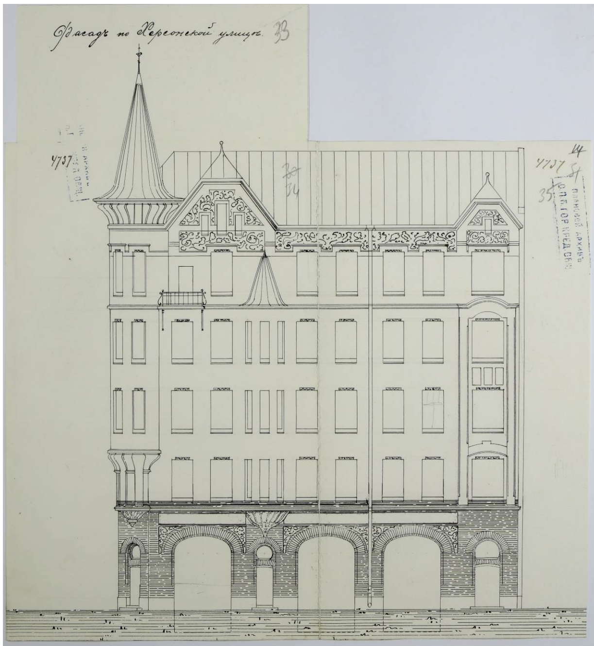
14. Фасад по Херсонской улице. Л.33-35. ЦГИА СПб. Фонд 515. Опись 4. Дело 5724. Чертежи дома А.П.Шерстобитова, П.В. Клименко, К.К. Шмидта по Херсонской ул.,13 и Перекупному пер.,12. (1862–1916)
