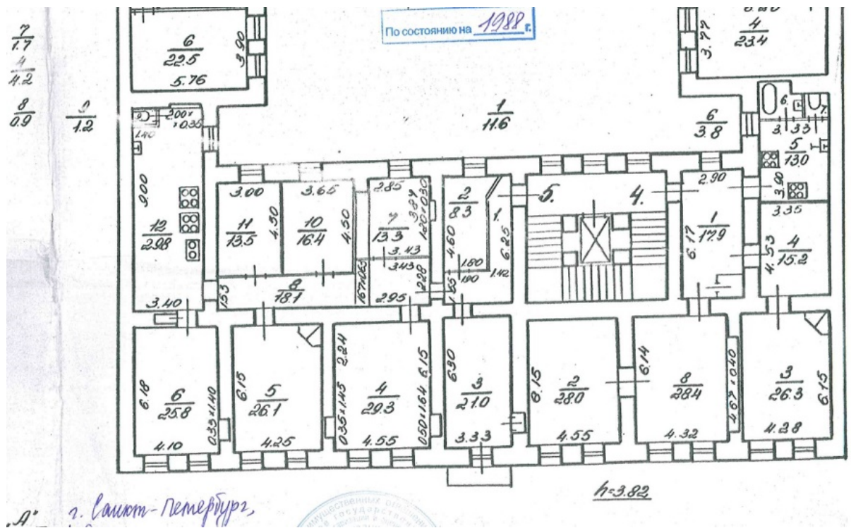
76. План 2 этажа дома № 6 по Невскому проспекту. 1988 г. Филиал ГУП ГУИОН ПИБ Центрального района.
