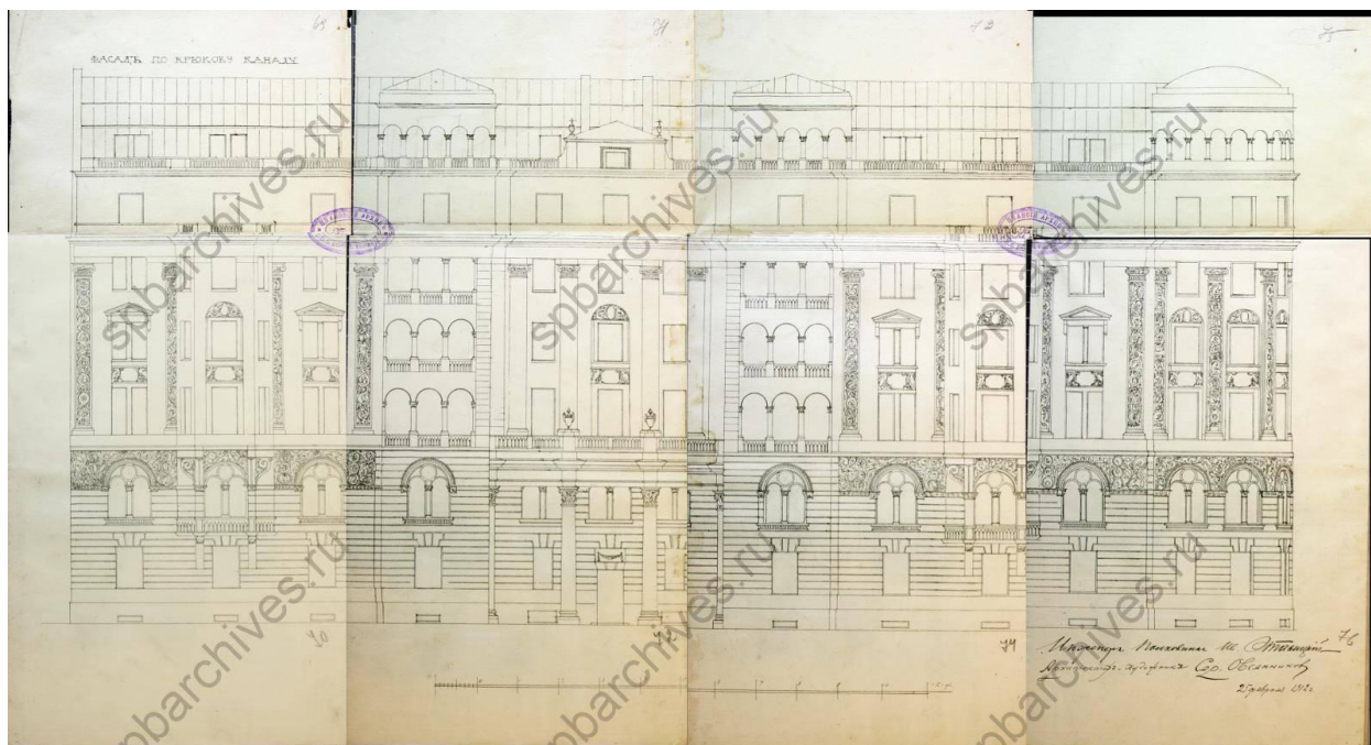
16. Фасад по Крюкову каналу. 1912 г. // ЦГИА СПб. Фонд 513. Опись 102. Дело 3354.
