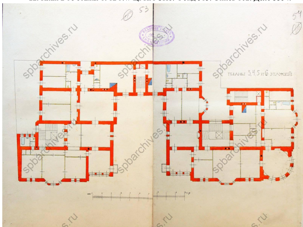
13. План 3, 4, 5, и 6-го этажей. 1912 г. // ЦГИА СПб. Фонд 513. Описание 102. Дело 3354.
