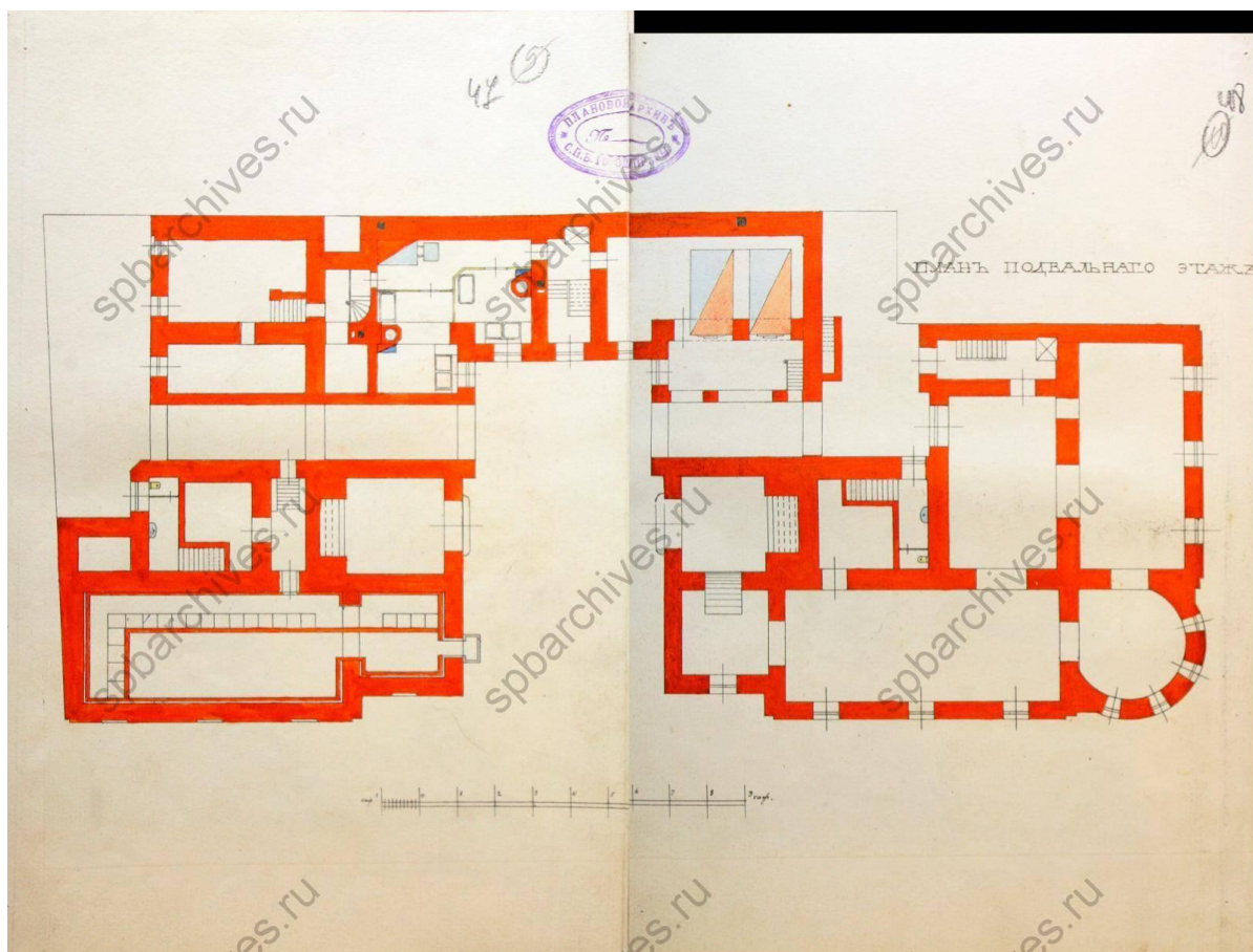
10. План подвального этажа. 1912 г. // ЦГИА СПб. Фонд 513. Опись 102. Дело 3354.
