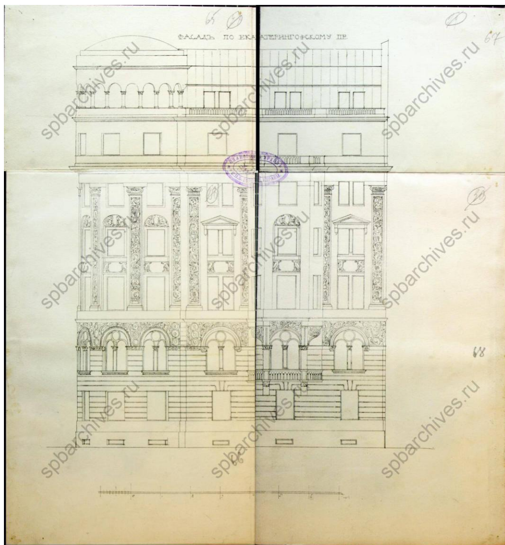
15. Фасад по Екатерингофскому пв. 1912 г. // ЦГИА СПб. Фонд 513. Опись 102. Дело 3354.
