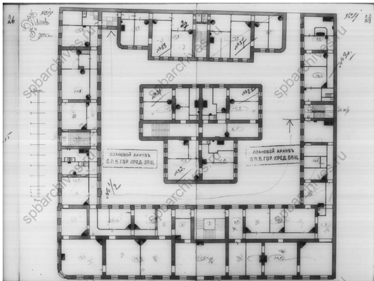
Илл. 32. План двора дома, принадлежащего графине Марии Дмитриевны Нирод. План 3-го этажа. Архитектор А. Каценко. 1908. ЦГИА СПб. Ф. 515. Оп. 4. Д. 4289. Л. 27-28.
