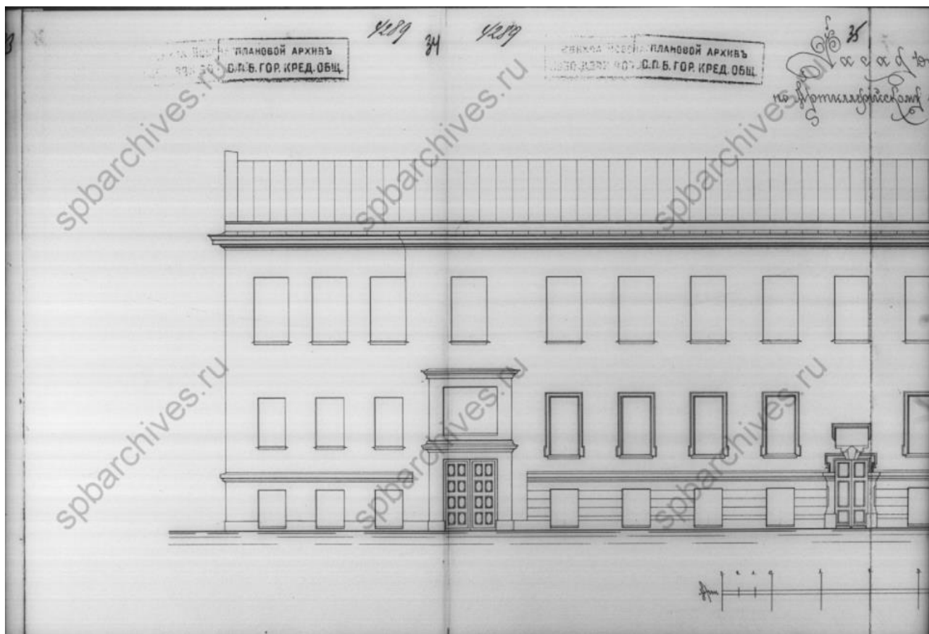
Илл. 35. План двора дома, принадлежащего графине Марии Дмитриевны Нирод. Фасад по Артиллерийскому переулку. Архитектор А. Кащенко. 1908. ЦГИА СПб. Ф. 515. Оп. 4. Д. 4289. Л. 34-35.
