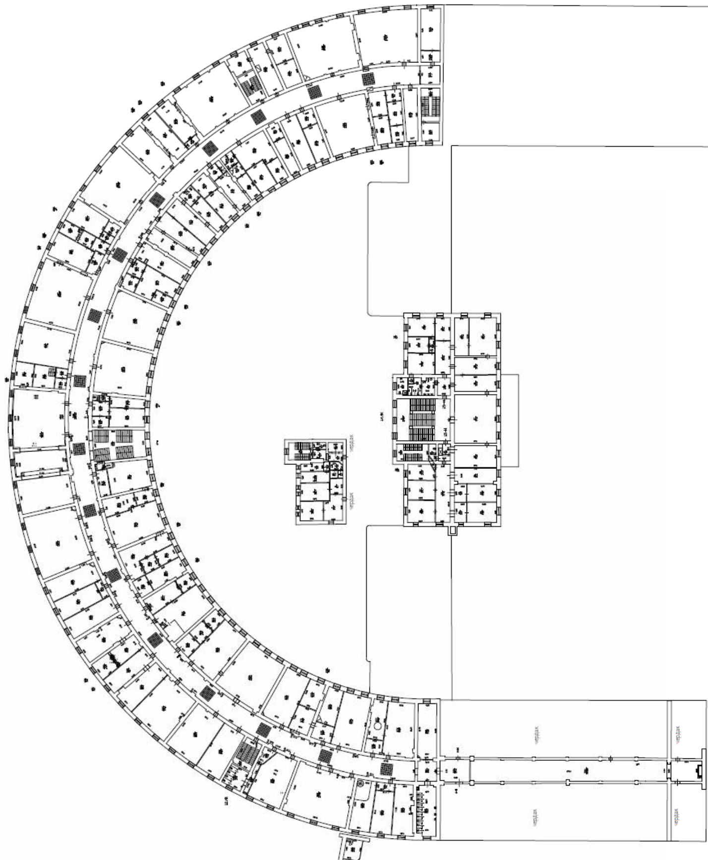
План 3 этажа
