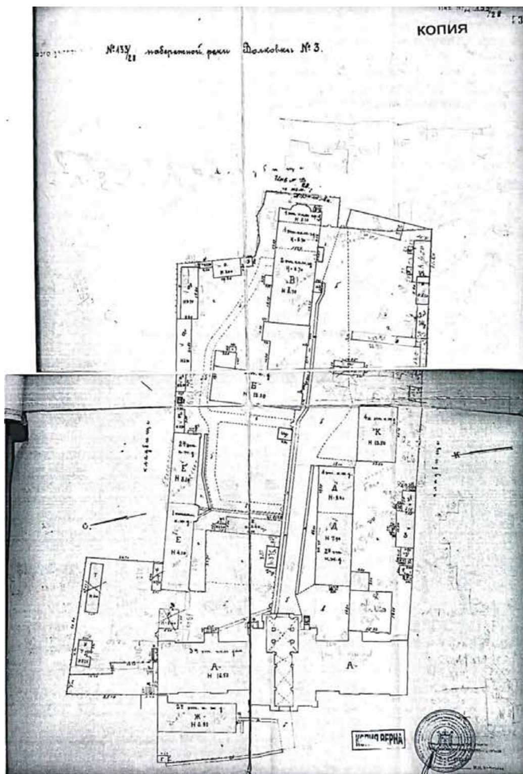
Илл. 16. План участка по наб. р. Волковки №3.
