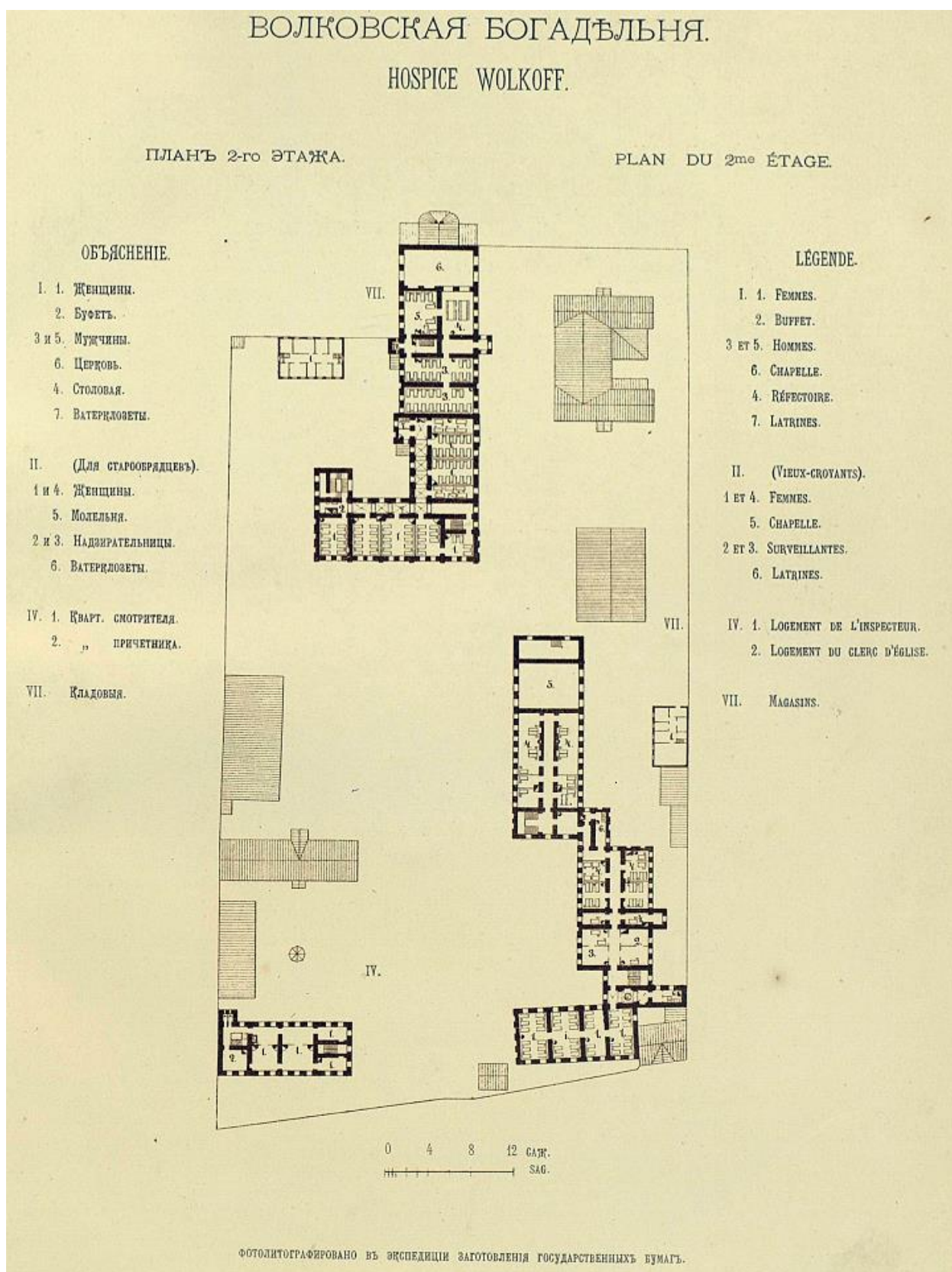
Илл. 15. План 2 этажа. 1878 // Попечительный совет заведений общественного призрения в С.-Петербурге. Очерк деятельности за пятьдесят лет 1828–1878. По поручению попечительного совета. Составил и издал К. Ордин, член совета. СПб., 1878.
