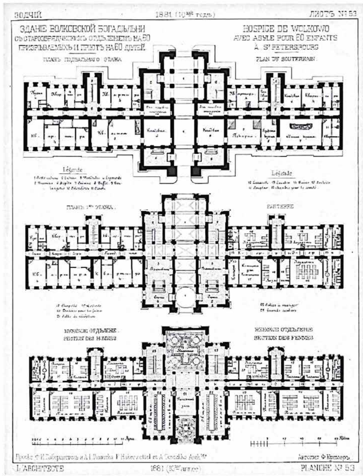
Илл. 18. План подвального, 1 и 2 этажей. Архитекторы Ф.И. Габерцетль, А.И. Томишко // Зодчий. 1881 г.
