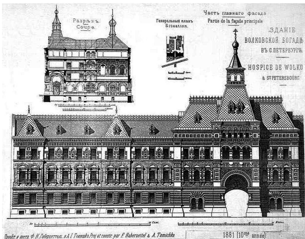
Илл. 19. Часть главного фасада // Зодчий. 1881 г.
