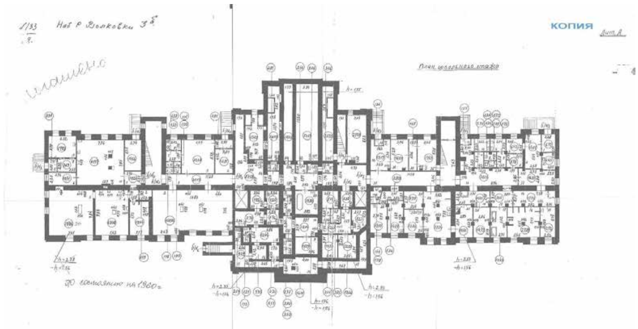
Илл. 27. План цокольного этажа. 1960 г. // ПИБ
