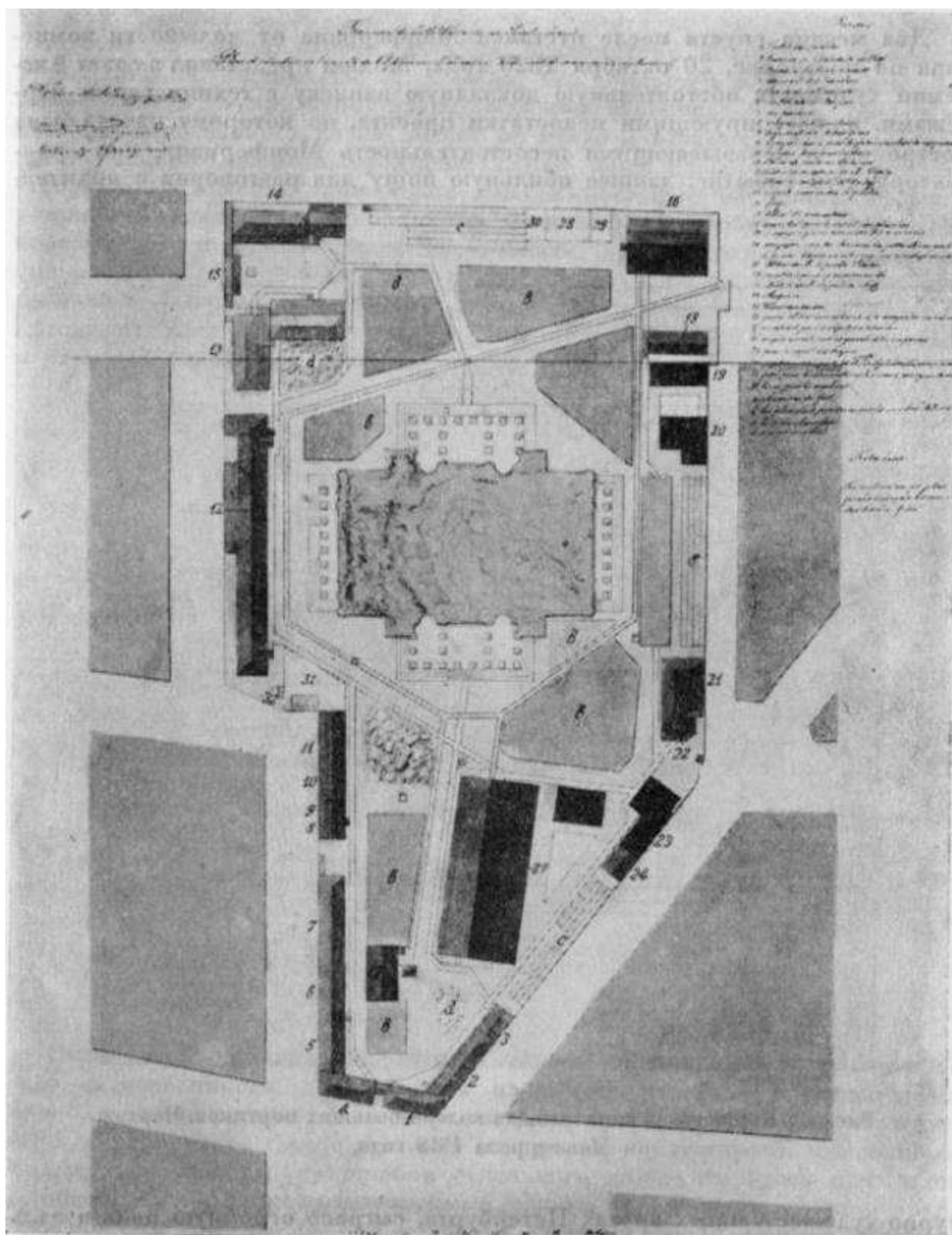
Илл. 10. Генеральный план строительной площадки Исаакиевского собора, 1847.
