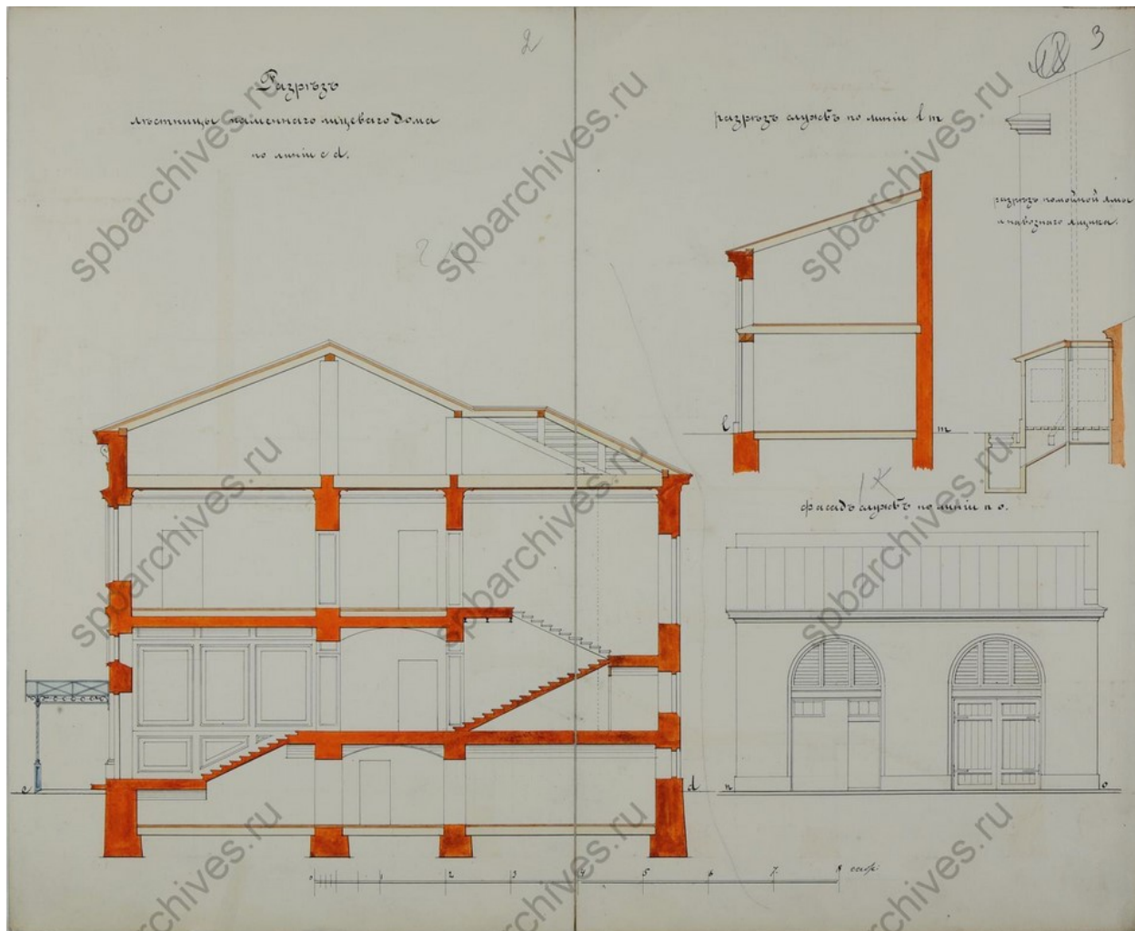
Илл. 14. Разрез лестницы каменного лицевого дома по линии CD, разрез служб по линии LM, фасад служб по линии NO. 1873 г. ЦГИА СПб. Ф. 513. Оп. 102. Д. 5310. Л. 2-3.
