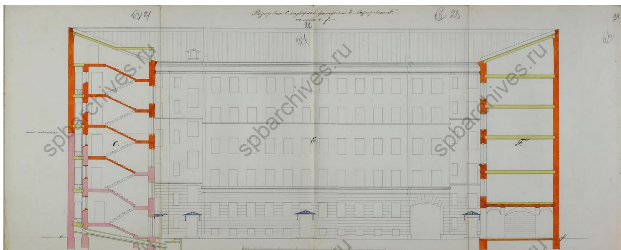
Илл. 24. Разрез лит. С, надворный фасад лит. Е и разрез лит. Е по линии ЕЕ. 1877 г. ЦГИА СПб. Ф. 513. Оп. 102. Д. 5310. Л. 21-24.
