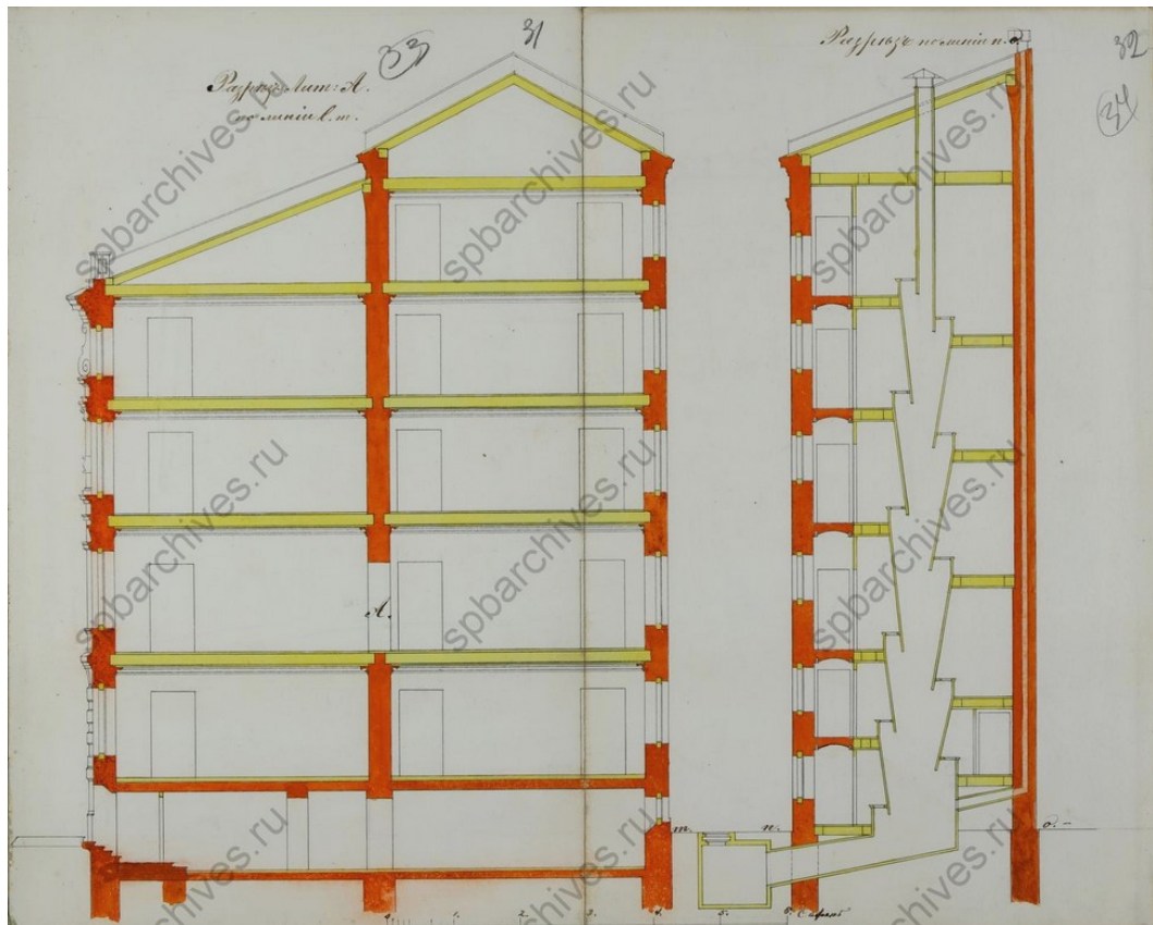
Илл. 27. Разрез лит. А по линии LM. 1877 г. ЦГИА СПб. Ф. 513. Оп. 102. Д. 5310. Л. 31-32.
