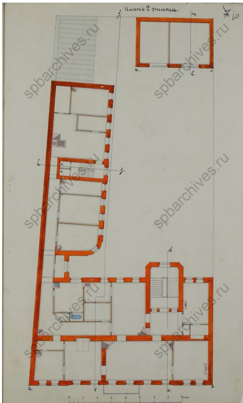
Илл. 19. План 2-го этажа. 1873 г. ЦГИА СПб. Ф. 513. Оп. 102. Д. 5310. Л. 10.
