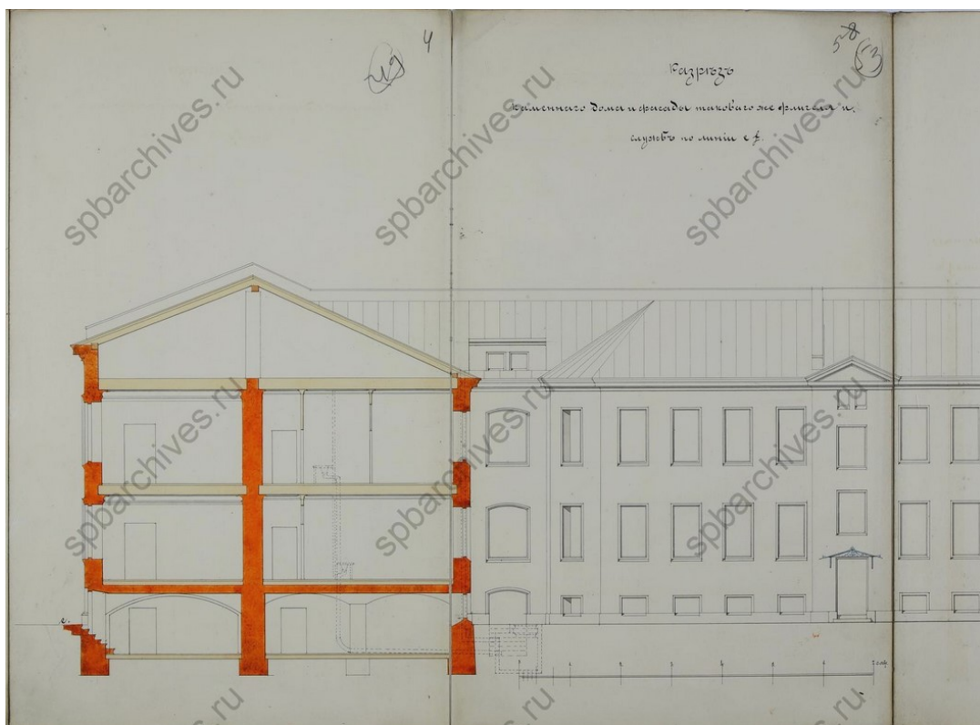
Илл. 15. Разрез каменного дома и фасады такового флигеля и служб по линии ЕФ. 1873 г. ЦГИА СПб. Ф. 513. Оп. 102. Д. 5310. Л. 4-5.
