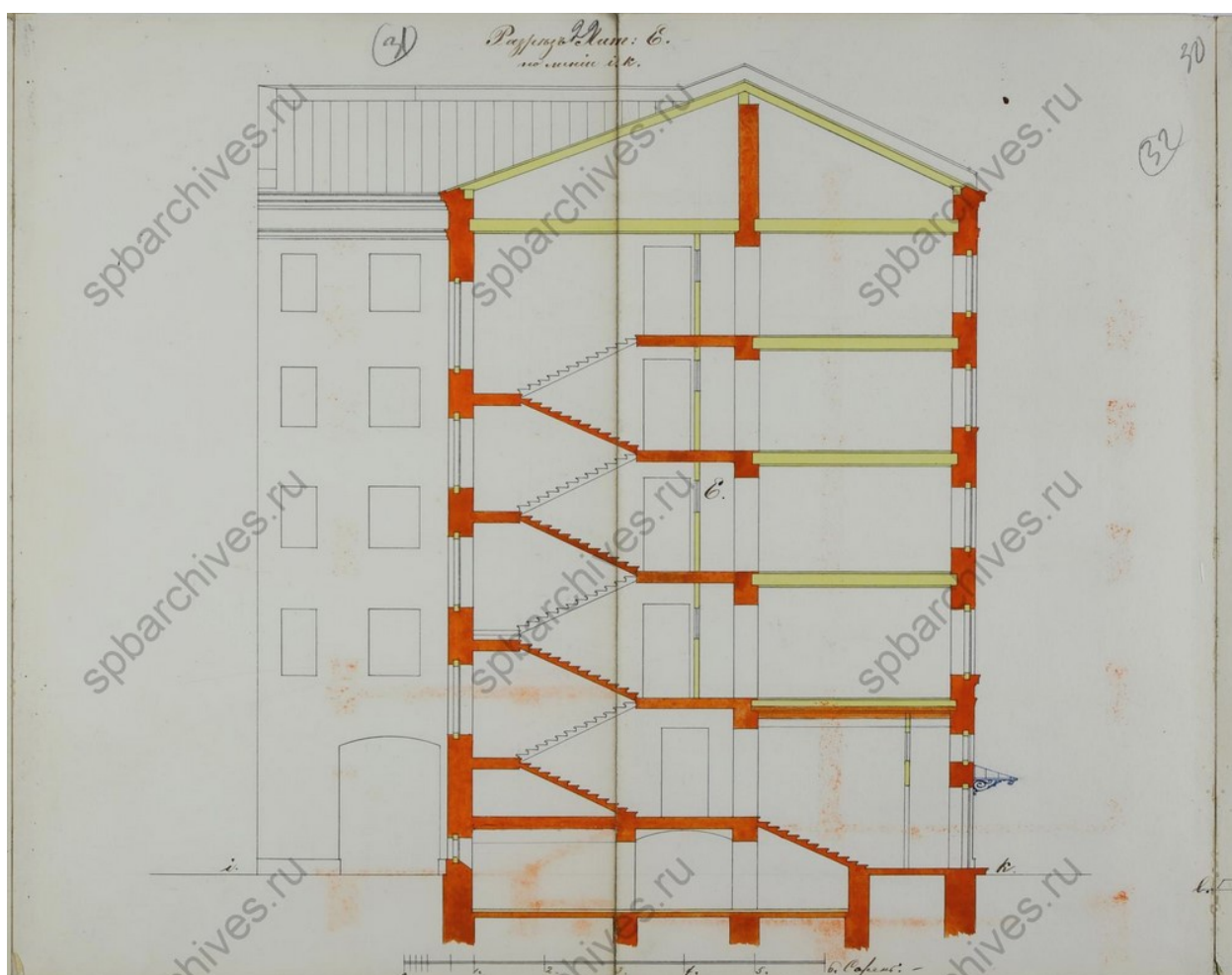
Илл. 26. Разрез лит. Е по линии IK. 1877 г. ЦГИА СПб. Ф. 513. Оп. 102. Д. 5310. Л. 29-30.
