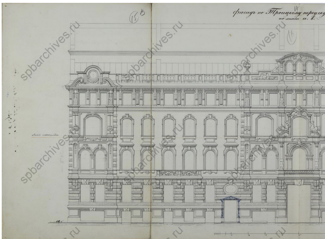
Илл. 21. Фасад по Троицкому переулку по линии АВ. 1877 г. ЦГИА СПб. Ф. 513. Оп. 102. Д. 5310. Л. 13-14.
