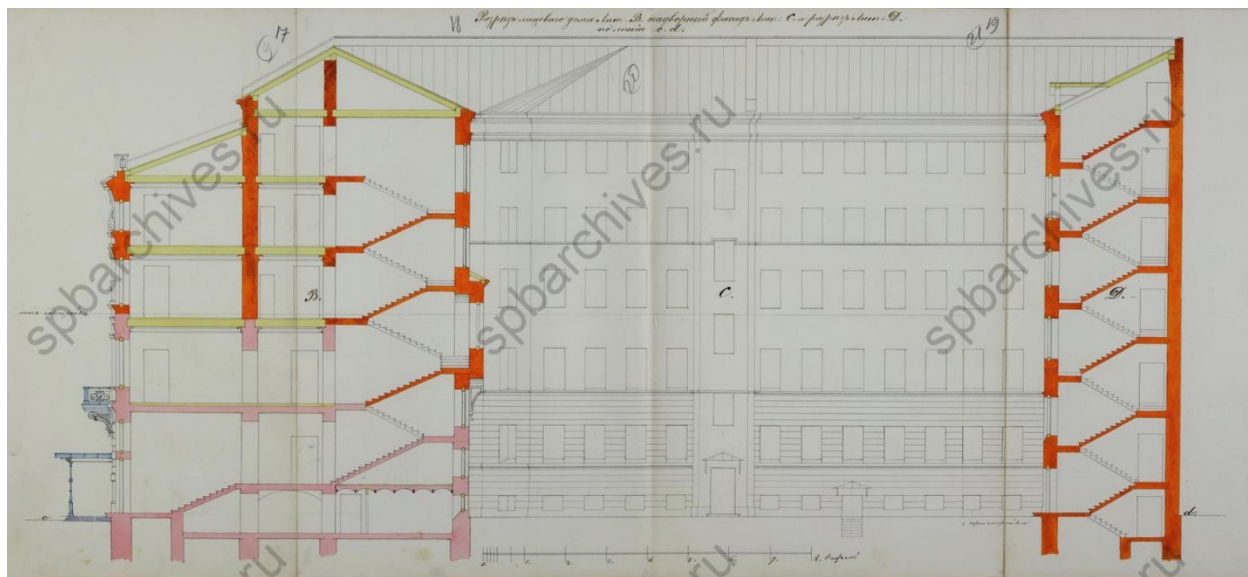
Илл. 23. Разрез лицевого дома лит. В, надворный фасад лит. С. и разрез лит. Д по линии СД. 1877 г. ЦГИА СПб. Ф. 513. Оп. 102. Д. 5310. Л. 17-20.
