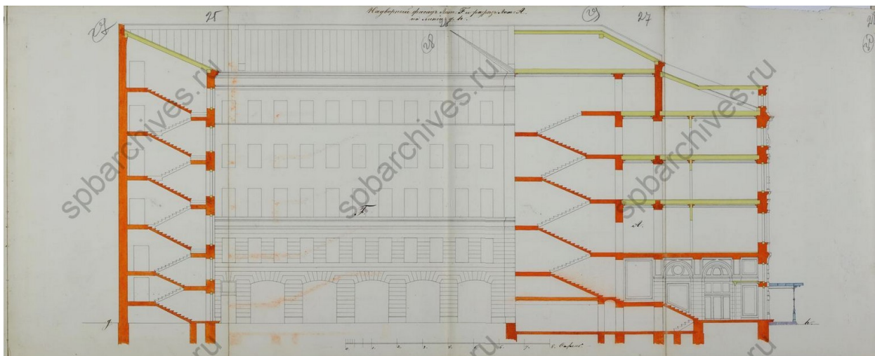
Илл. 25. Надворный фасад лит. F и разрез лит. А по линии GH. 1877 г. ЦГИА СПб. Ф. 513. Оп. 102. Д. 5310. Л. 25-28.
