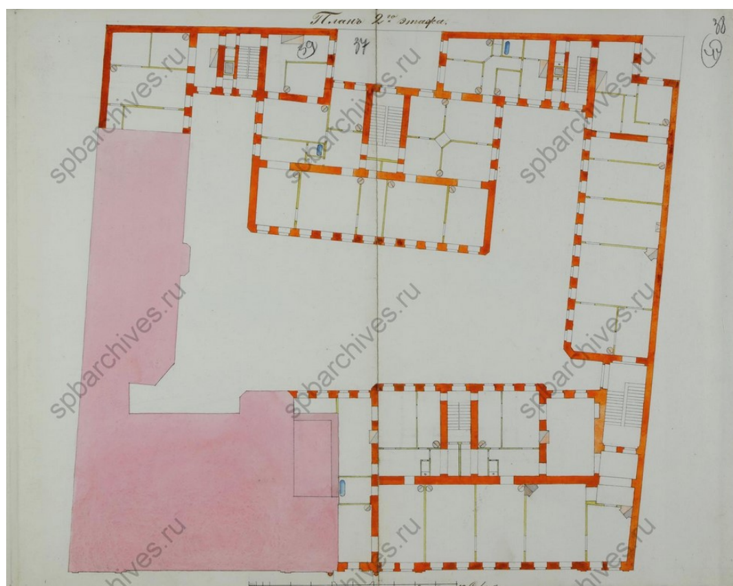
Илл. 30. План 2-го этажа. 1877 г. ЦГИА СПб. Ф. 513. Оп. 102. Д. 5310. Л. 37-38.
