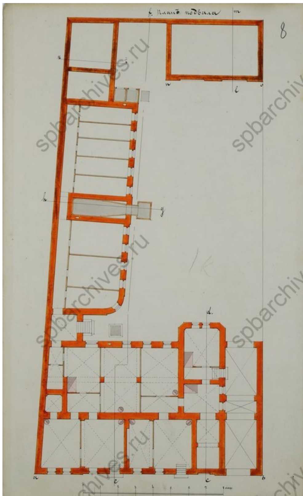
Илл. 17. План подвала. 1873 г. ЦГИА СПб. Ф. 513. Оп. 102. Д. 5310. Л. 8.
