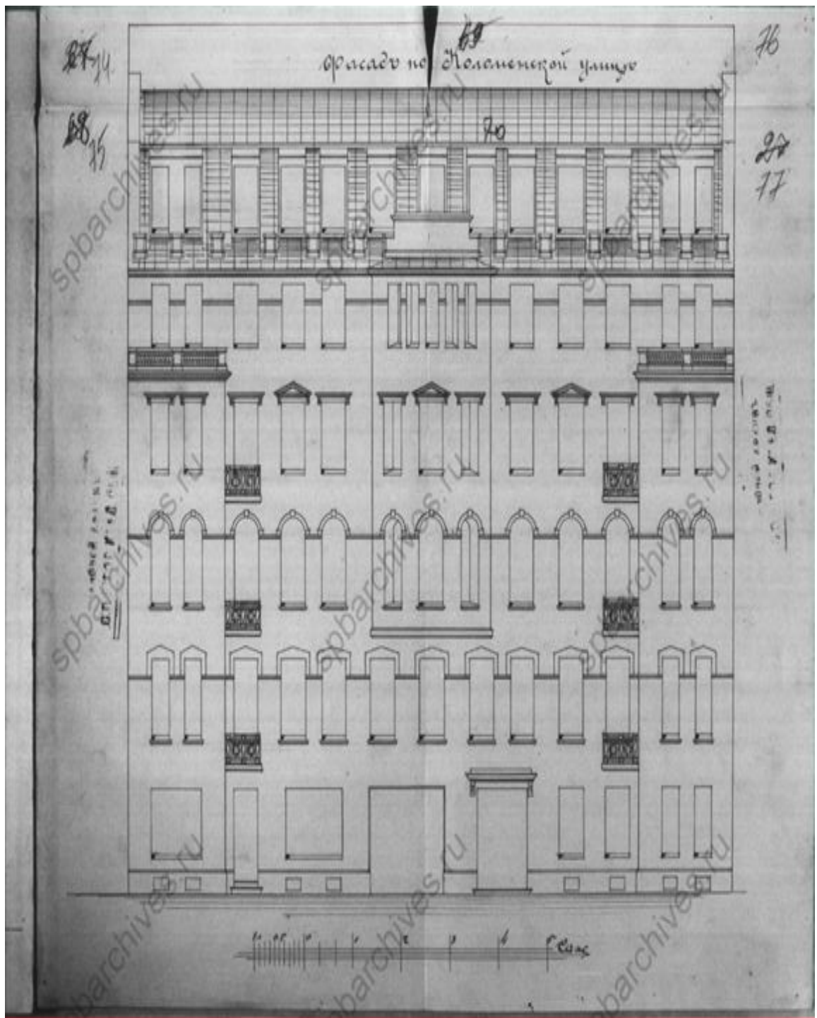
Илл. 10. Выписки из Плана 1; Московской части; улица Коломенская, участок 2, фасад по Коломенской улице, 1913г.// ЦГИА СПб. Фонд 515. Опись 4. Дело 1793. Чертежи дома А.И. Каличицкой, И.Ф. и Н.И. Дыренковых по Коломенской ул., 13
