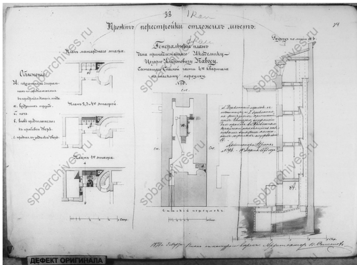
19. План перестройки отхожих мест дома, принадлежащего Титулярному Советнику Ц. А. Кавосу. 1858 г. Чертежи дома на участке, принадлежавшем И.И.Иванову, Ц.А.Кавосу, Е.Ц.Кавос, А.И.Суслову по Спасскому пер., 10. ЦГИА СПб ф.513 оп.102 д.9902. Л.33-34;
