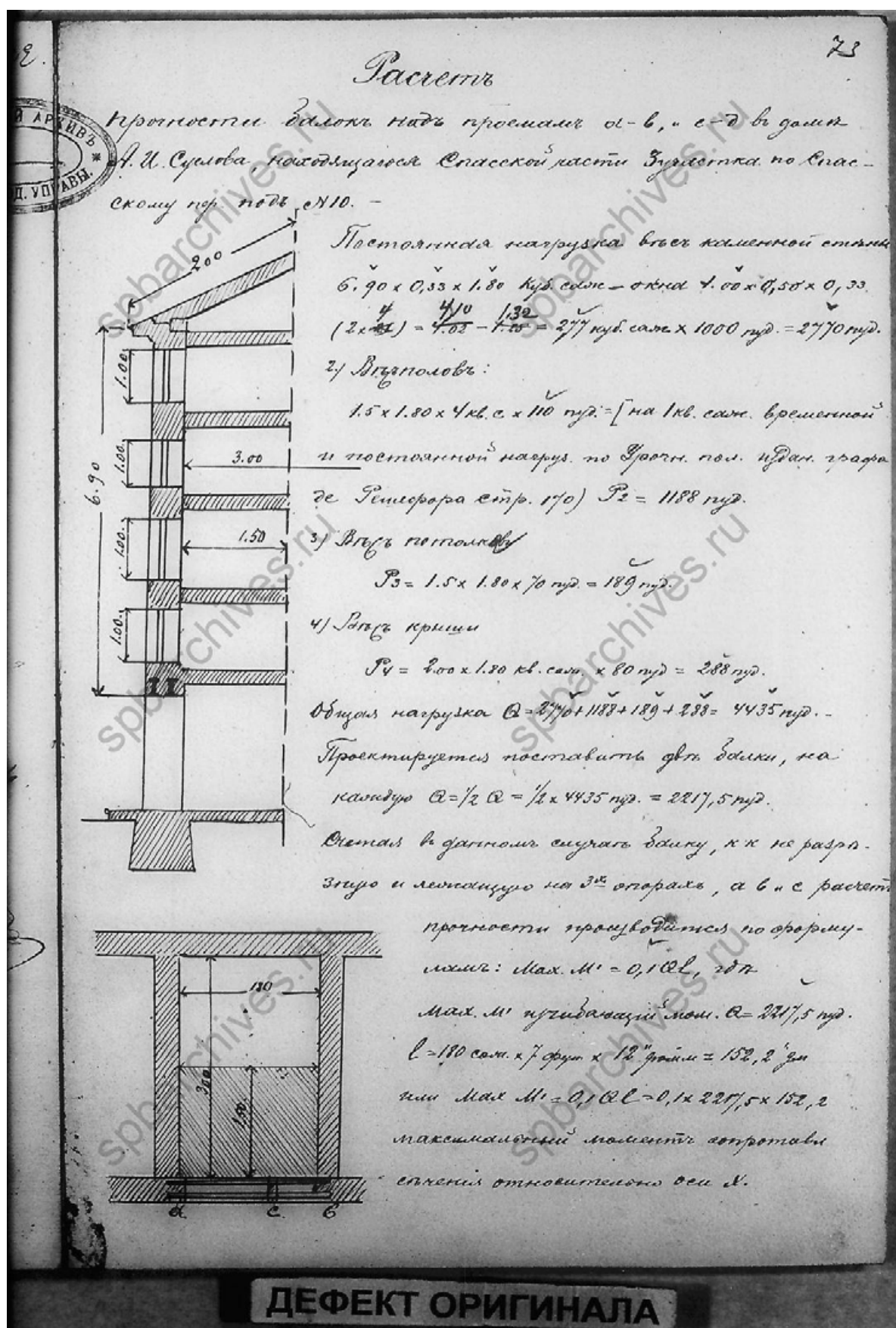
52. Расчеты прочности балок дома, принадлежащего Титулярному Советнику Ц. А. Кавосу. 1858 г. Чертежи дома на участке, принадлежавшем И.И.Иванову, Ц.А.Кавосу, Е.Ц.Кавос, А.И.Суслову по Спасскому пер., 10. ЦГИА СПб ф.513 оп.102 д.9902. Л.73;
