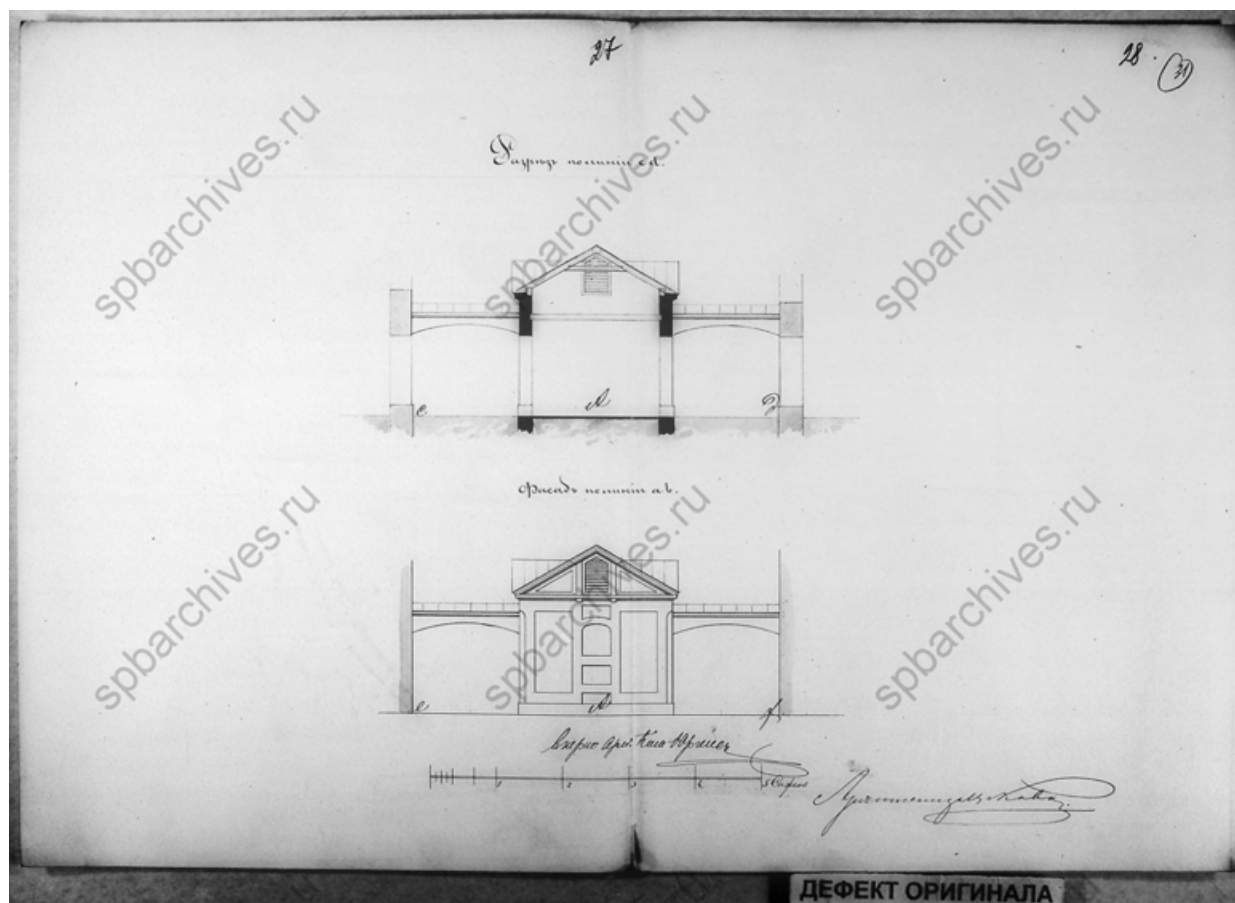
16. Разрез по линии CD дома, принадлежащего Титулярному Советнику Ц. А. Кавосу. 1858 г. Чертежи дома на участке, принадлежавшем И.И.Иванову, Ц.А.Кавосу, Е.Ц.Кавос, А.И.Суслову по Спасскому пер., 10. ЦГИА СПб ф.513 оп.102 д.9902. Л.27-28;
