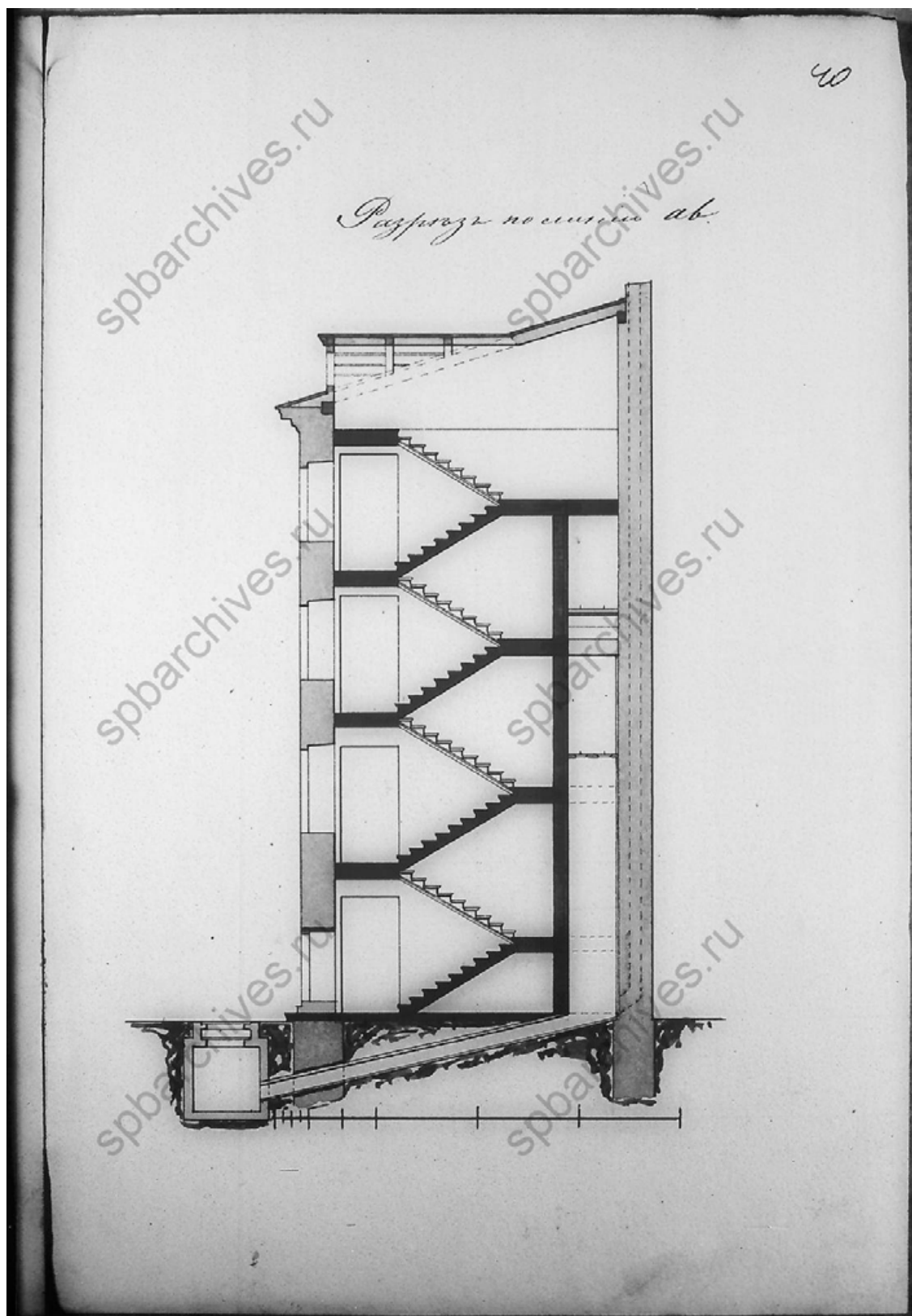
24. Разрез по линии а в дома, принадлежащего Титулярному Советнику Ц. А. Кавосу. 1858 г. Чертежи дома на участке, принадлежавшем И.И.Иванову, Ц.А.Кавосу, Е.Ц.Кавос, А.И.Сулову по Спасскому пер., 10. ЦГИА СПб ф.513 оп.102 д.9902. Л.40;
