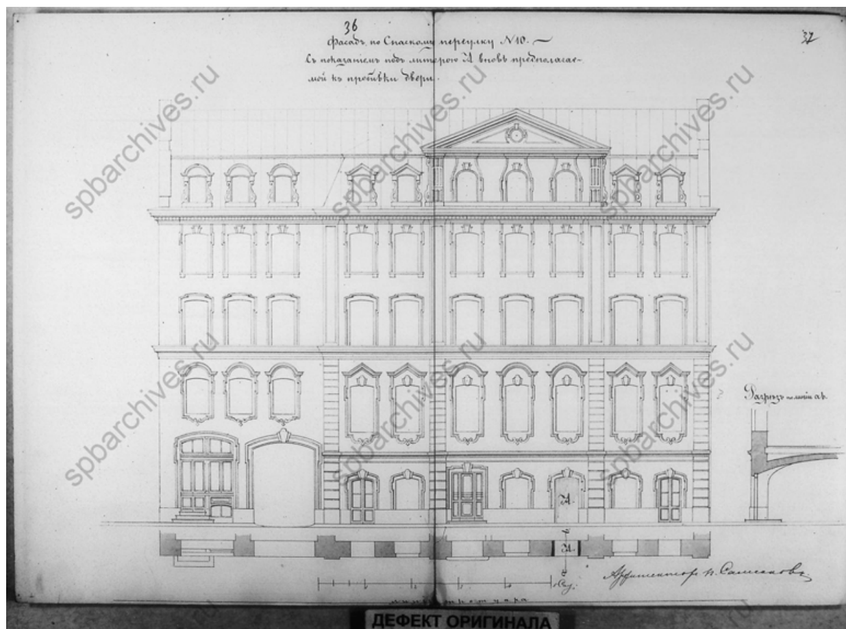
21. Фасад дома, принадлежащего Титулярному Советнику Ц. А. Кавосу. 1858 г. Чертежи дома на участке, принадлежавшем И.И.Иванову, Ц.А.Кавосу, Е.Ц.Кавос, А.И.Суслову по Спасскому пер., 10. ЦГИА СПб ф.513 оп.102 д.9902. Л.36-37;
