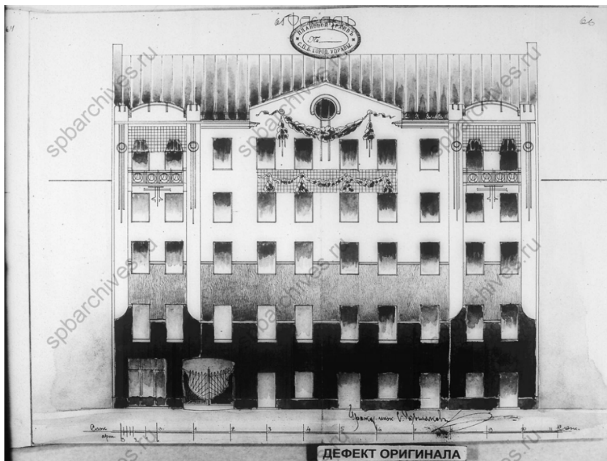
46. Фасад дома, принадлежащего Титулярному Советнику Ц. А. Кавосу. 1858 г. Чертежи дома на участке, принадлежавшем И.И.Иванову, Ц.А.Кавосу, Е.Ц.Кавос, А.И.Суслову по Спасскому пер., 10. ЦГИА СПб ф.513 оп.102 д.9902. Л.65-66;
