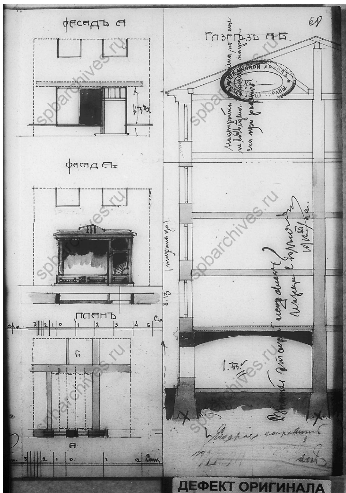
48. Фасад и разрезы дома, принадлежащего Титулярному Советнику Ц. А. Кавосу. 1858 г. Чертежи дома на участке, принадлежавшем И.И.Иванову, Ц.А.Кавосу, Е.Ц.Кавос, А.И.Суслову по Спасскому пер., 10. ЦГИА СПб ф.513 оп.102 д.9902. Л.68;
