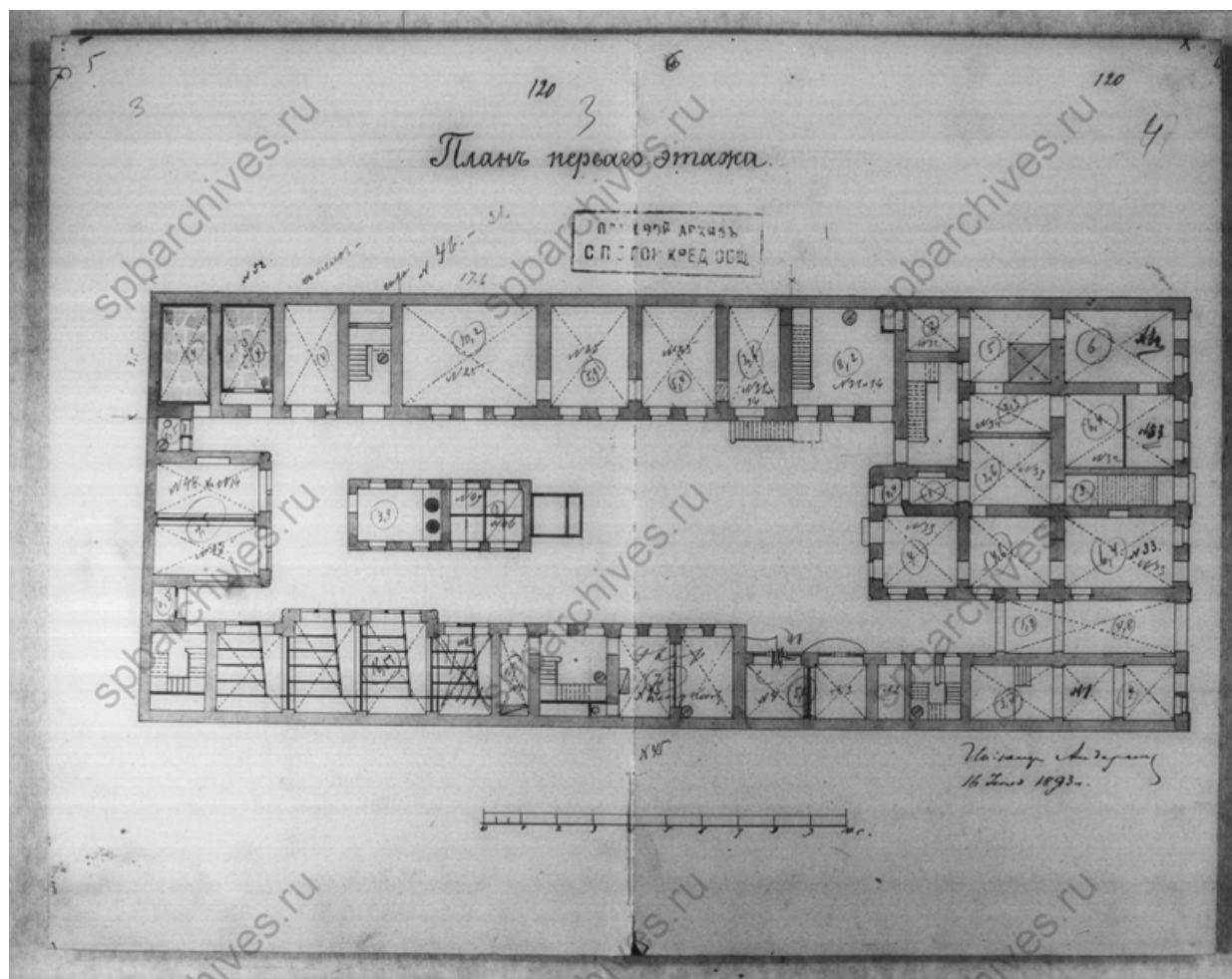
58. План первого этажа. Чертежи дома Е.Ц.Кавоса по Спасскому пер.,10. ЦГИА СПб. Фонд 515. Опись 4. Дело 33. 10.08.1892–08.02.1900. ЛЗ-4;
