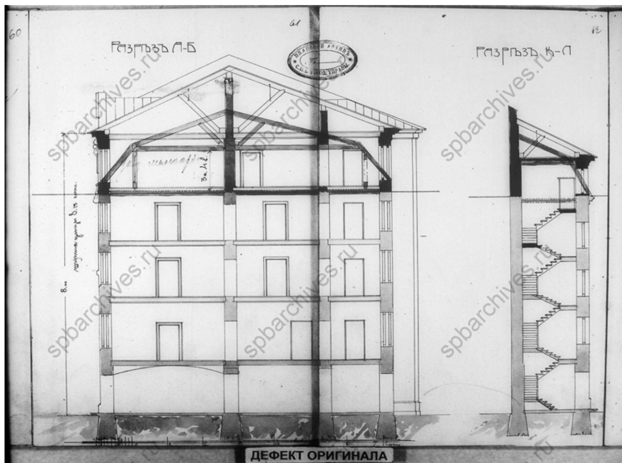
44. Разрезы дома, принадлежащего Титулярному Советнику Ц. А. Кавосу. 1858 г. Чертежи дома на участке, принадлежавшем И.И.Иванову, Ц.А.Кавосу, Е.Ц.Кавос, А.И.Суслову по Спасскому пер., 10. ЦГИА СПб ф.513 оп.102 д.9902. Л.61-62;
