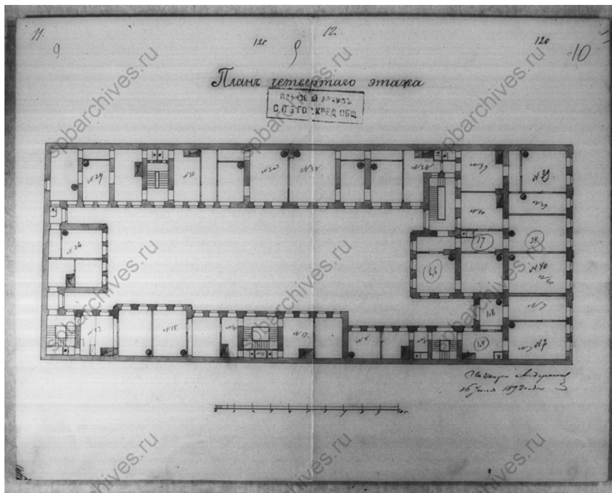
61. План четвертого этажа. Чертежи дома Е.Ц.Кавоса по Спасскому пер.,10. ЦГИА СПб. Фонд 515. Опись 4. Дело 33. 10.08.1892–08.02.1900. Л9-10;
