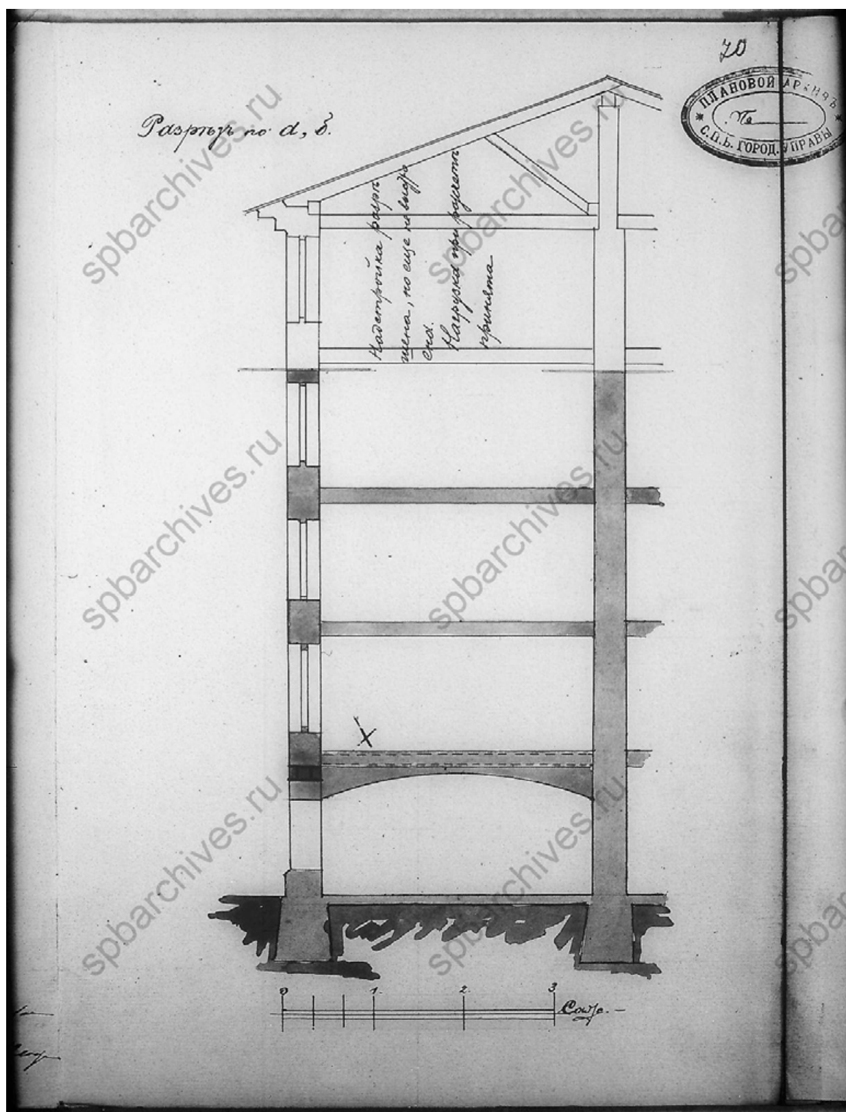
50. Разрез по а,б дома, принадлежащего Титулярному Советнику Ц. А. Кавосу. 1858 г. Чертежи дома на участке, принадлежавшем И.И.Иванову, Ц.А.Кавосу, Е.Ц.Кавос, А.И.Суслову по Спасскому пер., 10. ЦГИА СПб ф.513 оп.102 д.9902. Л.70;
