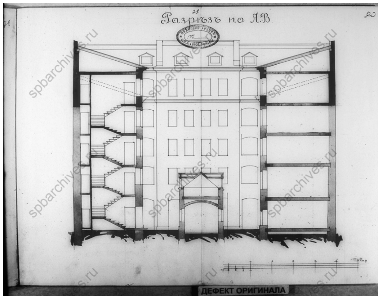
56. Разрез по АВ дома, принадлежащего Титулярному Советнику Ц. А. Кавосу. 1858 г. Чертежи дома на участке, принадлежавшем И.И.Иванову, Ц.А.Кавосу, Е.Ц.Кавос, А.И.Суслову по Спасскому пер., 10. ЦГИА СПб ф.513 оп.102 д.9902. Л.79-80;
