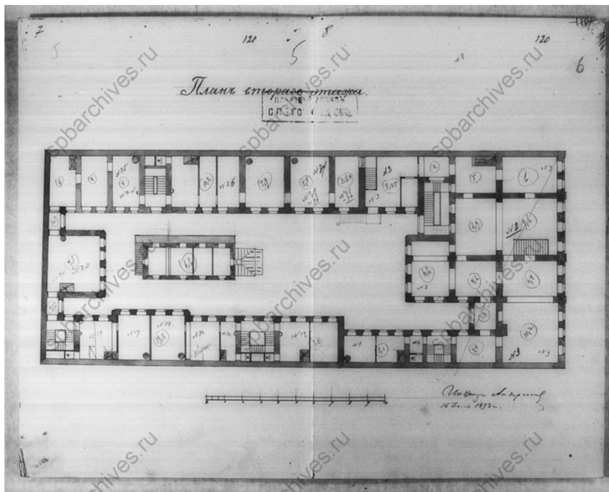
59. План второго этажа. Чертежи дома Е.Ц.Кавоса по Спасскому пер.,10. ЦГИА СПб. Фонд 515. Опись 4. Дело 33. 10.08.1892–08.02.1900. Л5-6;
