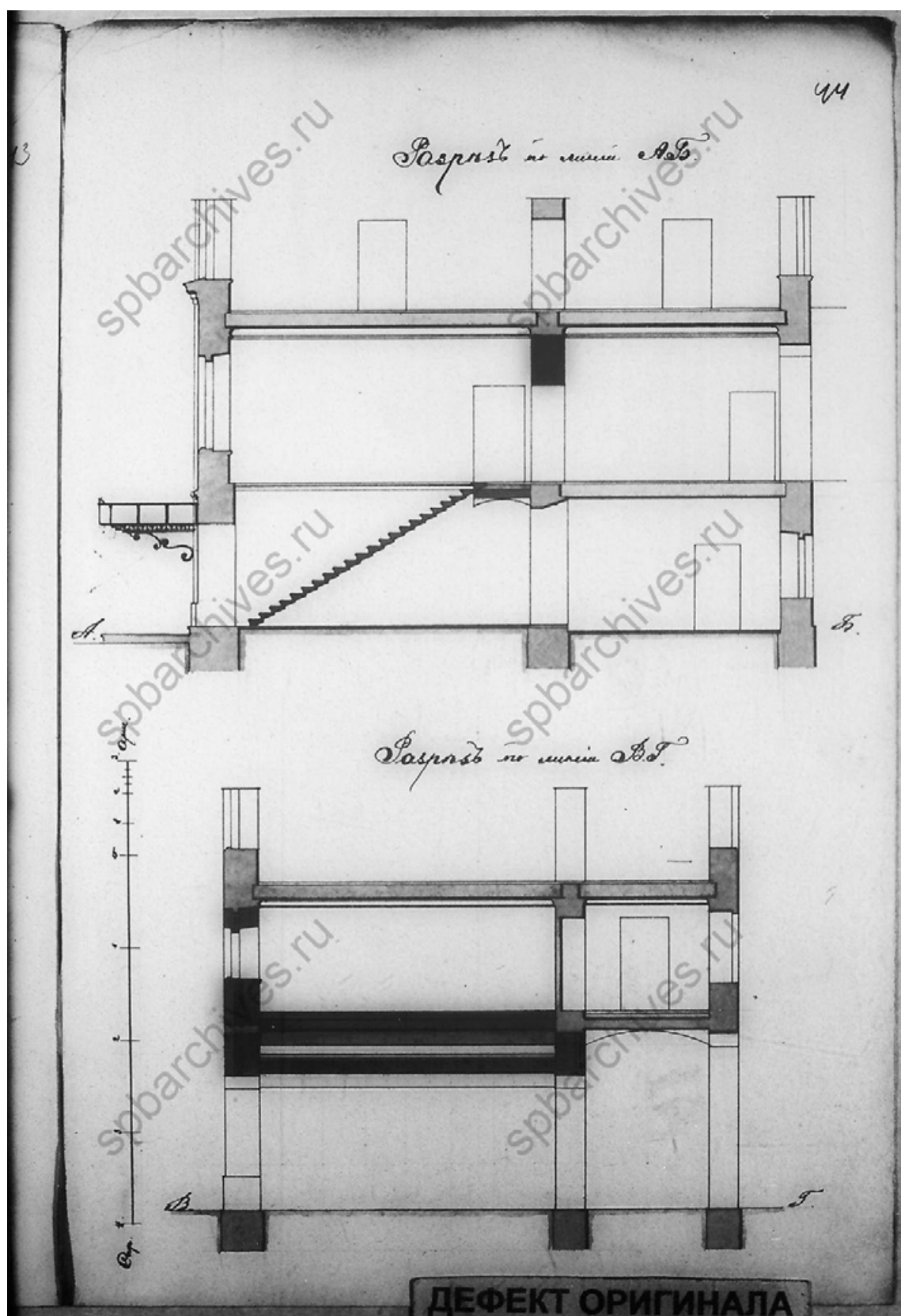
28. Разрез по линии АБ дома, принадлежащего Титулярному Советнику Ц. А. Кавосу. 1858 г. Чертежи дома на участке, принадлежавшем И.И.Иванову, Ц.А.Кавосу, Е.Ц.Кавос, А.И.Сулову по Спасскому пер., 10. ЦГИА СПб ф.513 оп.102 д.9902. Л.44;
