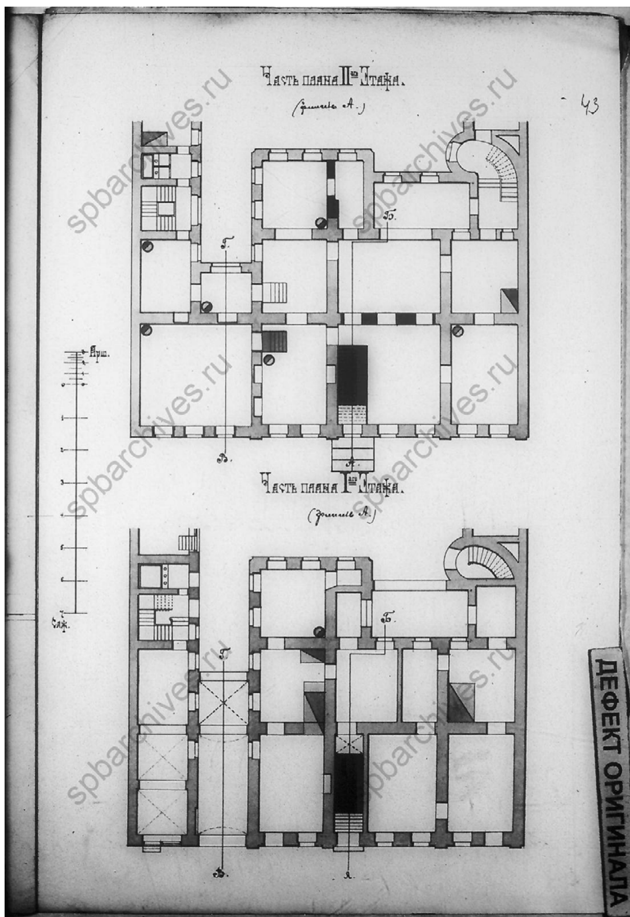
27. Поэтажный план дома, принадлежащего Титулярному Советнику Ц. А. Кавосу. 1858 г. Чертежи дома на участке, принадлежавшем И.И.Иванову, Ц.А.Кавосу, Е.Ц.Кавос, А.И.Суслову по Спасскому пер., 10. ЦГИА СПб ф.513 оп.102 д.9902. Л.43;
