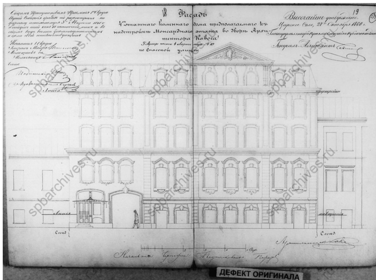
10. Фасад дома, принадлежащего Титулярному Советнику Ц. А. Кавосу. 1858 г. Чертежи дома на участке, принадлежавшем И.И.Иванову, Ц.А.Кавосу, Е.Ц.Кавос, А.И.Суслову по Спасскому пер., 10. ЦГИА СПб ф.513 оп.102 д.9902. Л.18-19;
