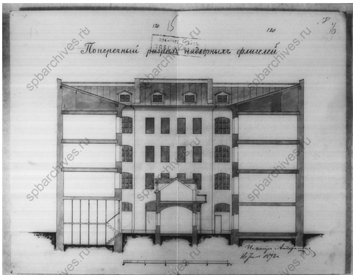
64. Разрез надворных флигелей. Чертежи дома Е.Ц.Кавоса по Спасскому пер.,10. ЦГИА СПб. Фонд 515. Опись 4. Дело 33. 10.08.1892–08.02.1900. 15-16;
