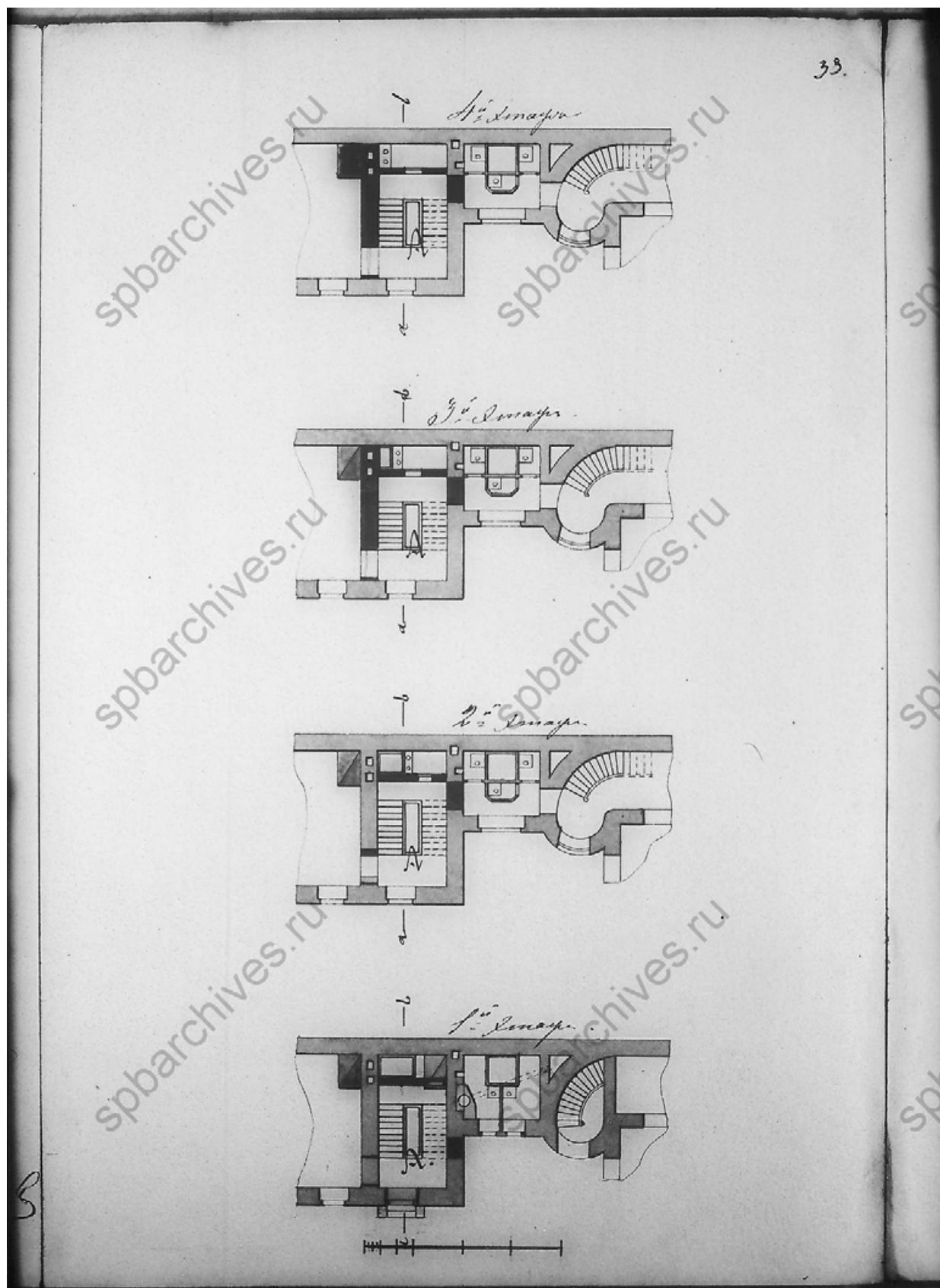
23. Поэтажный план дома, принадлежащего Титулярному Советнику Ц. А. Кавосу. 1858 г. Чертежи дома на участке, принадлежавшем И.И.Иванову, Ц.А.Кавосу, Е.Ц.Кавос, А.И.Сулову по Спасскому пер., 10. ЦГИА СПб ф.513 оп.102 д.9902. Л.39;
