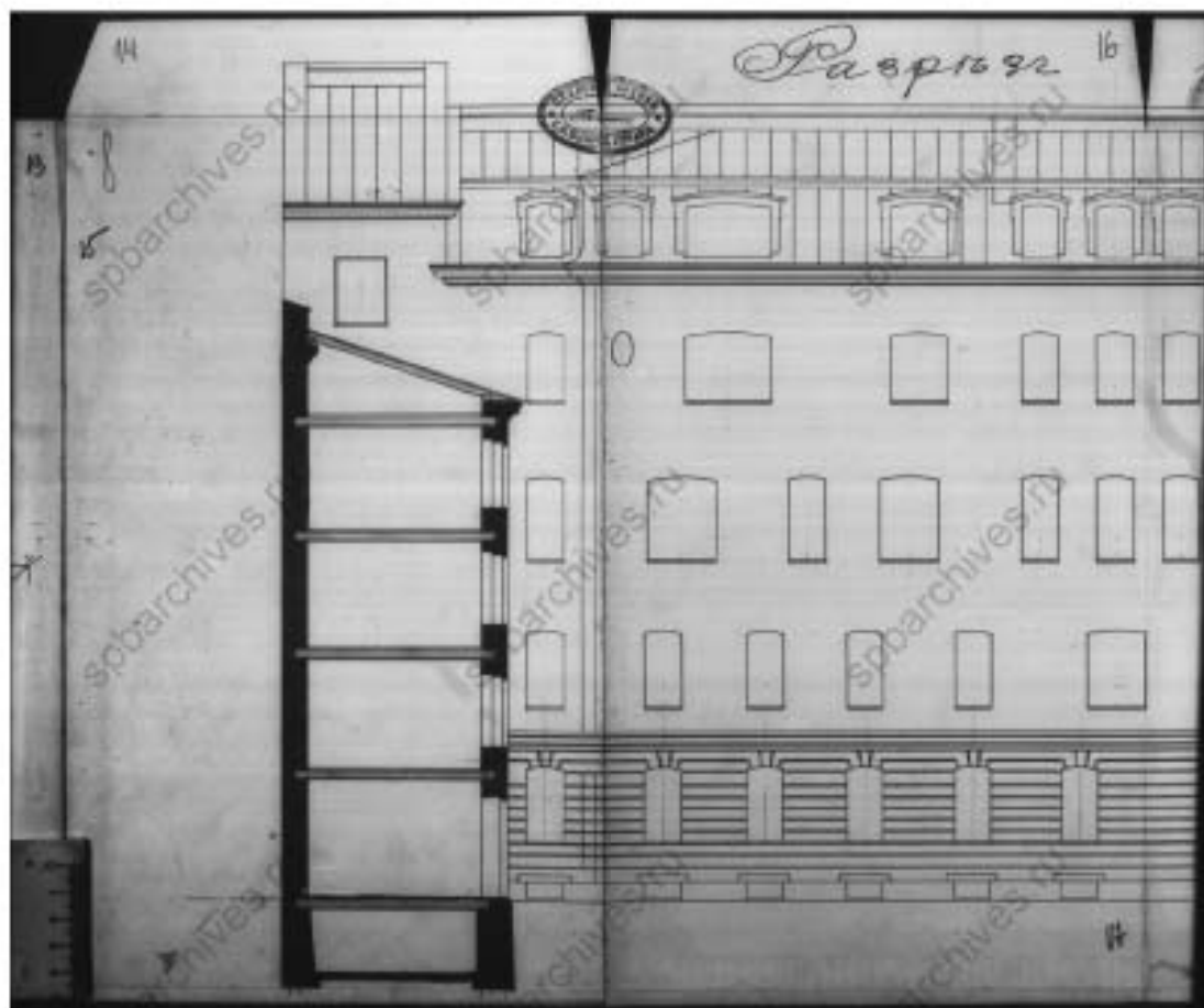
14. ЦГИА СПб. Фонд 515. Опись 4. Дело 3577. Чертежи дома В.С. Голенищева, М.Ф. Штифтер по Моховой ул., 15. 1861-1919 гг. Разрез.
