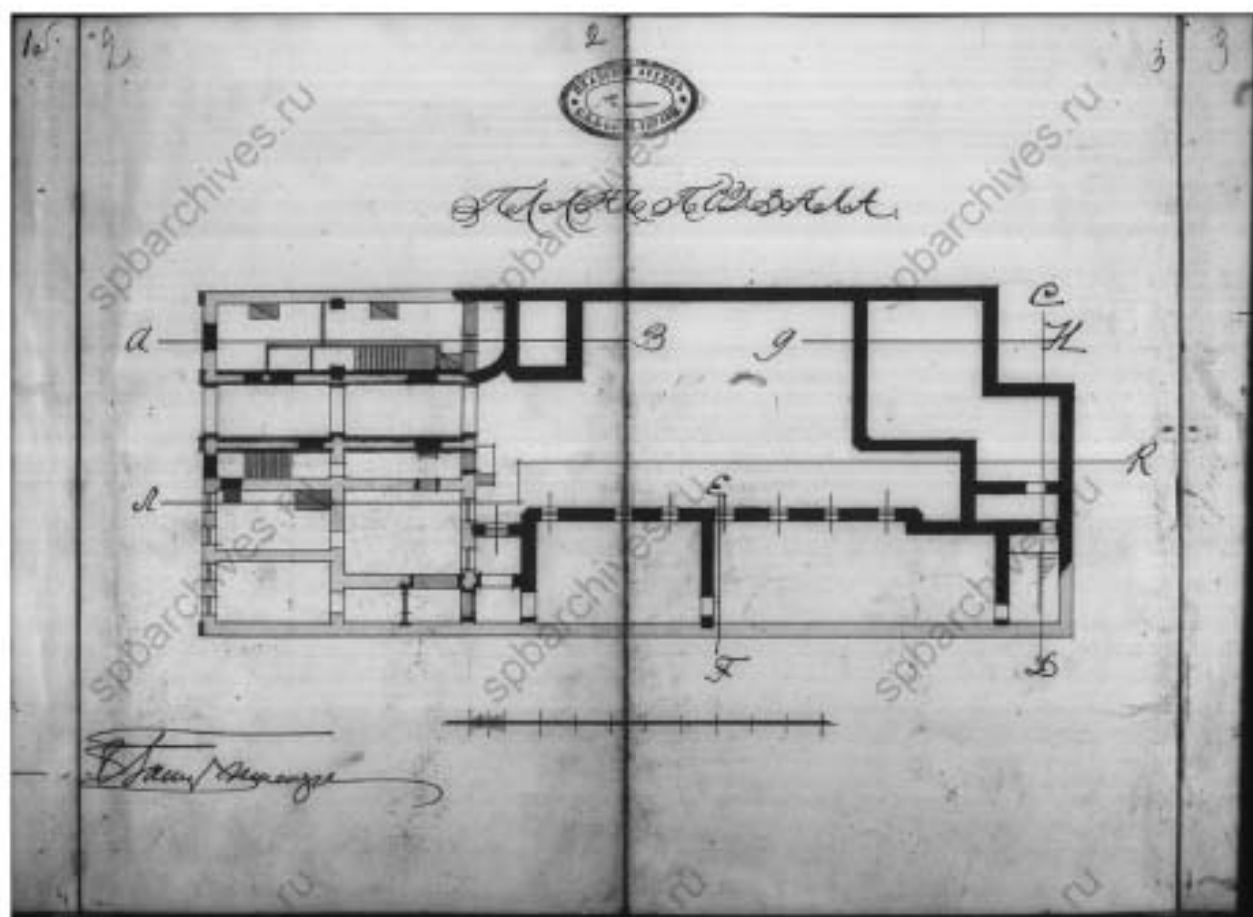
8. ЦГИА СПб. Фонд 515. Опись 4. Дело 3577. Чертежи дома В.С. Голенищева, М.Ф. Штифтер по Моховой ул., 15. 1861-1919 гг. План подвала.
