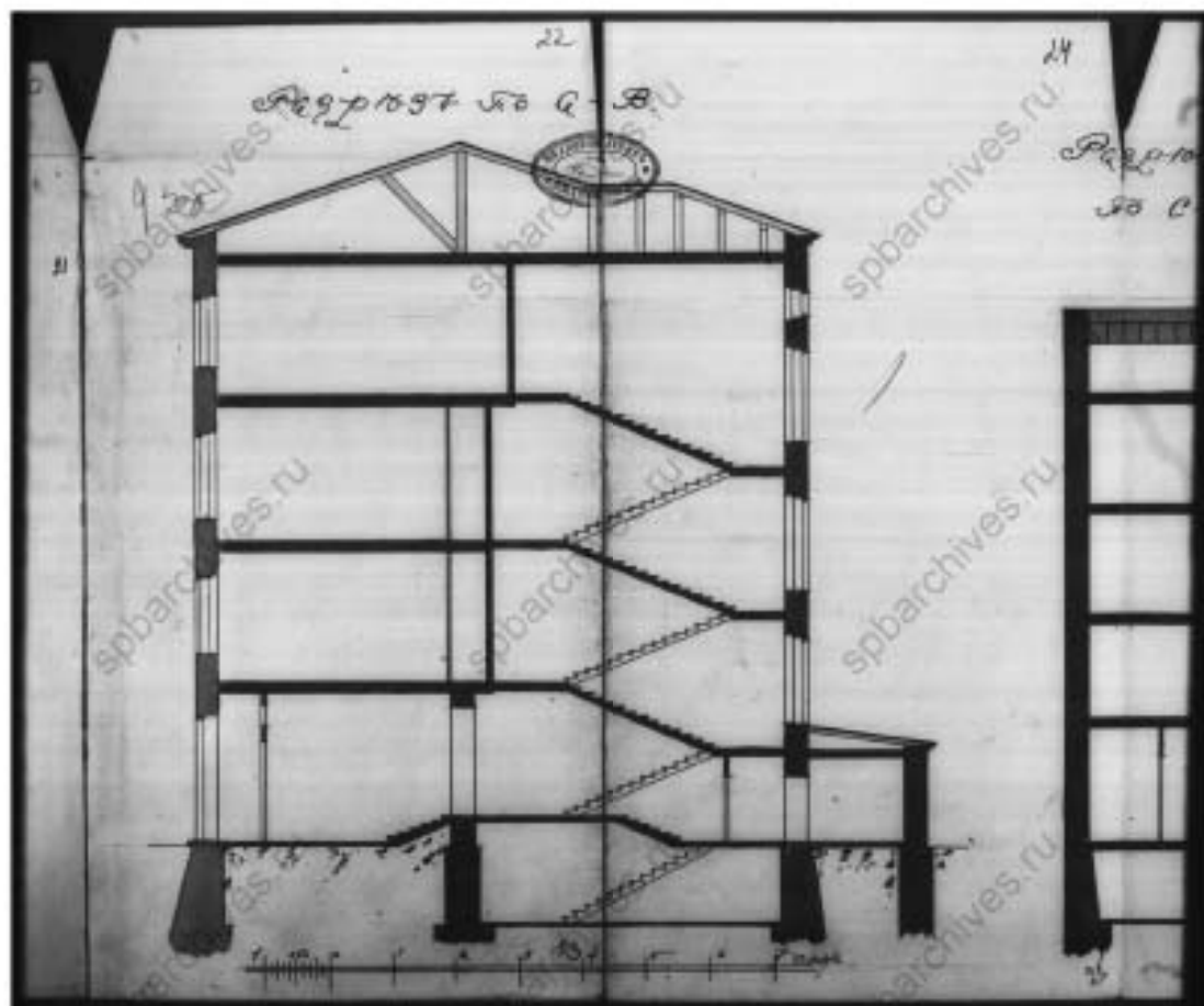
16. ЦГИА СПб. Фонд 515. Опись 4. Дело 3577. Чертежи дома В.С. Голенищева, М.Ф. Штифтер по Моховой ул., 15. 1861-1919 гг. Разрез.
