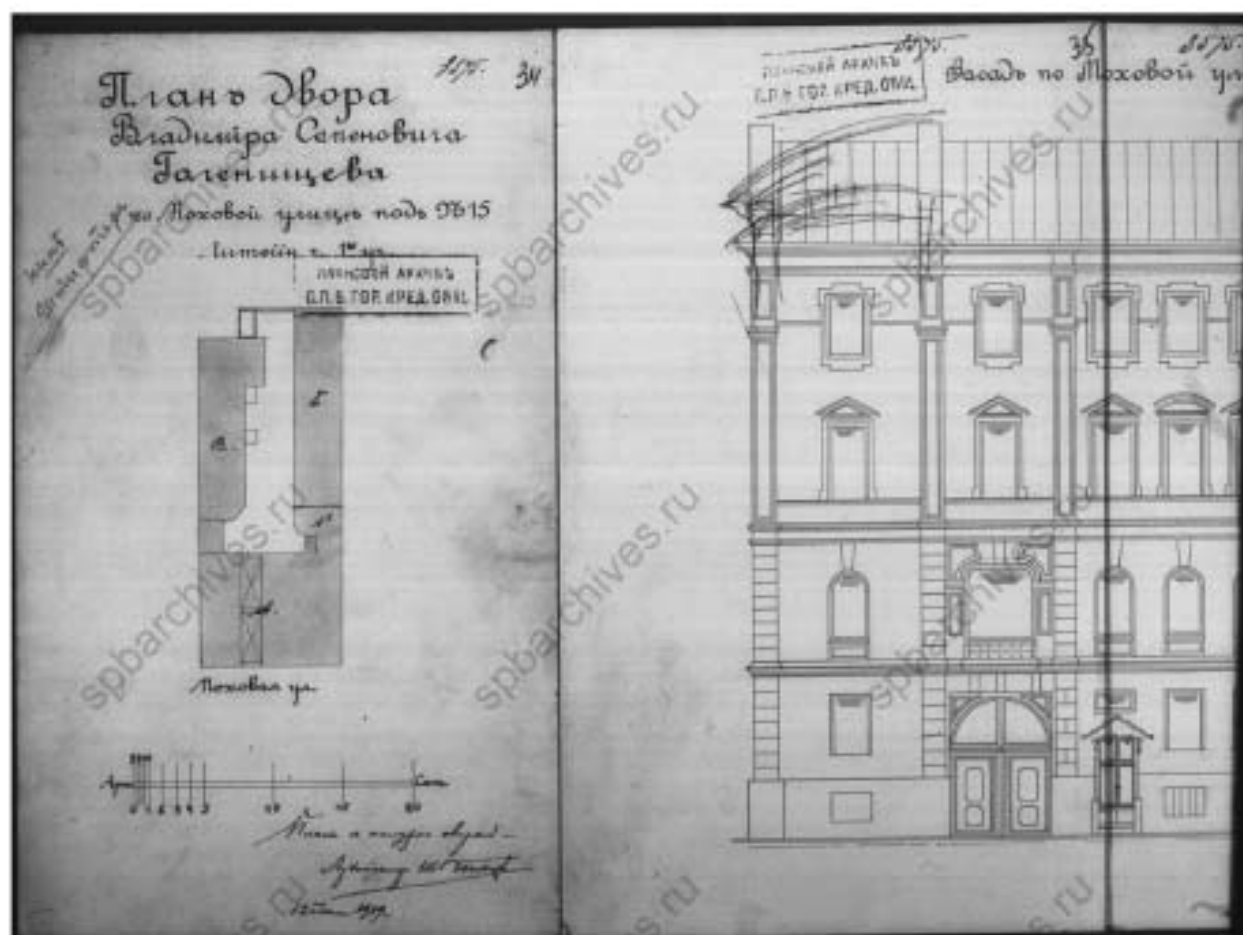
18. ЦГИА СПб. Фонд 515. Опись 4. Дело 3577. Чертежи дома В.С. Голенищева, М.Ф. Штифтер по Моховой ул., 15. 1861-1919 гг. План двора и часть фасада по Моховой.
