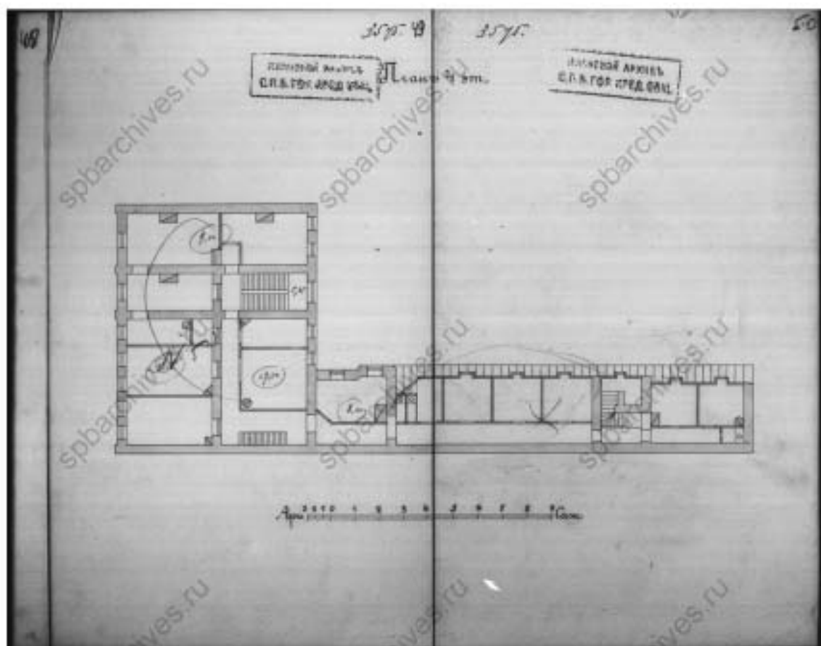
26. ЦГИА СПб. Фонд 515. Опись 4. Дело 3577. Чертежи дома В.С. Голенищева, М.Ф. Штифтер по Моховой ул., 15. 1861-1919 гг. План 4 этажа.
