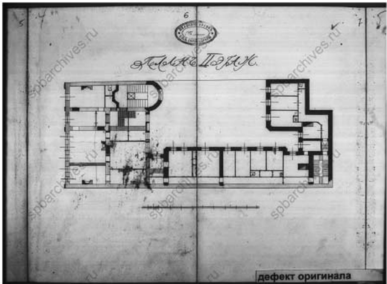
10. ЦГИА СПб. Фонд 515. Опись 4. Дело 3577. Чертежи дома В.С. Голенищева, М.Ф. Штифтер по Моховой ул., 15. 1861-1919 гг. План 2 этажа.
