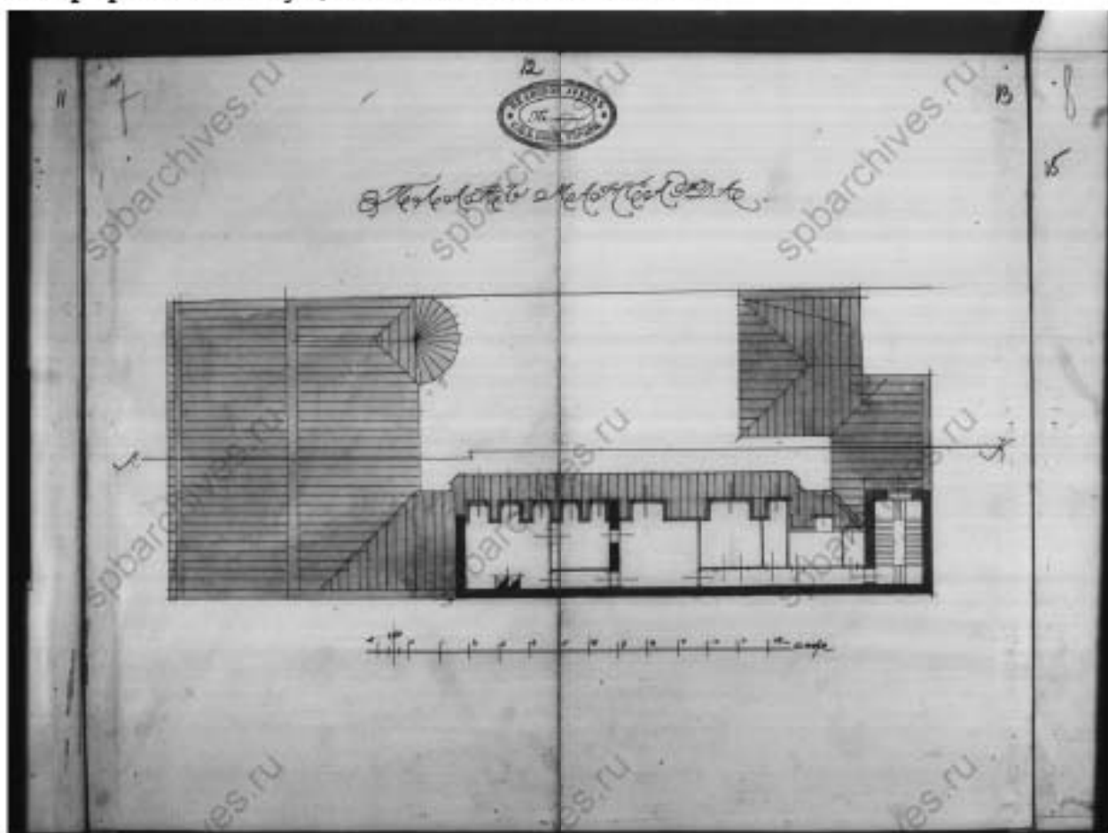
13. ЦГИА СПб. Фонд 515. Опись 4. Дело 3577. Чертежи дома В.С. Голенищева, М.Ф. Штифтер по Моховой ул., 15. 1861-1919 гг. План мансарды.
