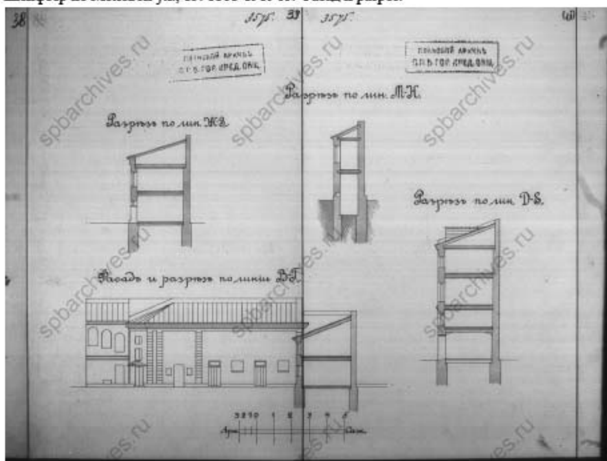
21. ЦГИА СПб. Фонд 515. Опись 4. Дело 3577. Чертежи дома В.С. Голенищева, М.Ф. Штифтер по Моховой ул., 15. 1861-1919 гг. Разрез.
