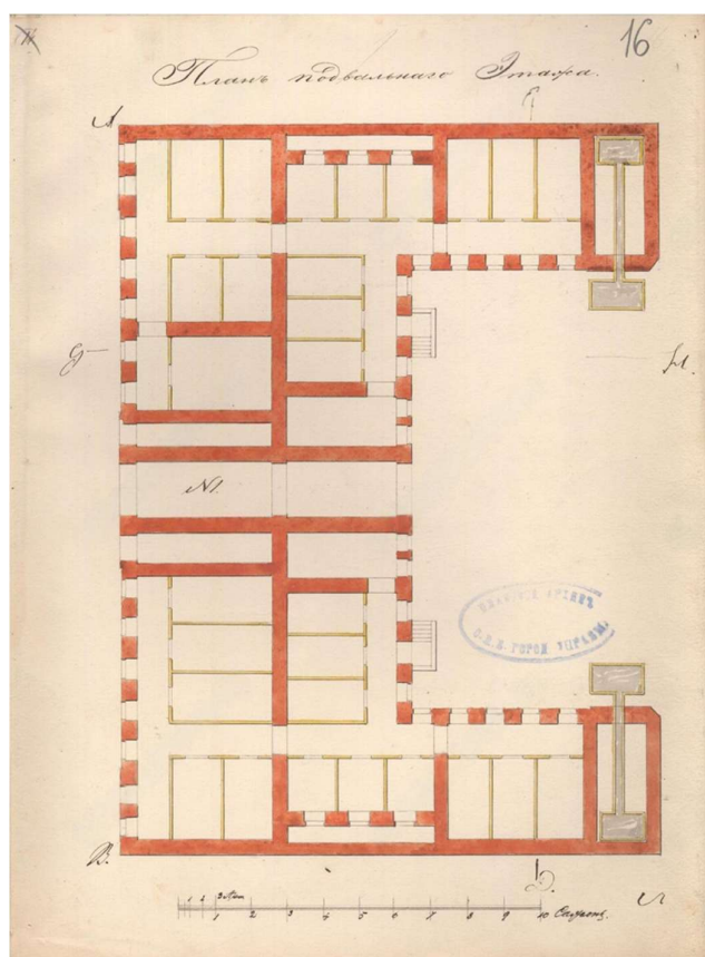
16. План подвального этажа. 1860 г. // Источник: ЦГИА СПб Ф.513 Оп.102 Д.1577 Л.16.
