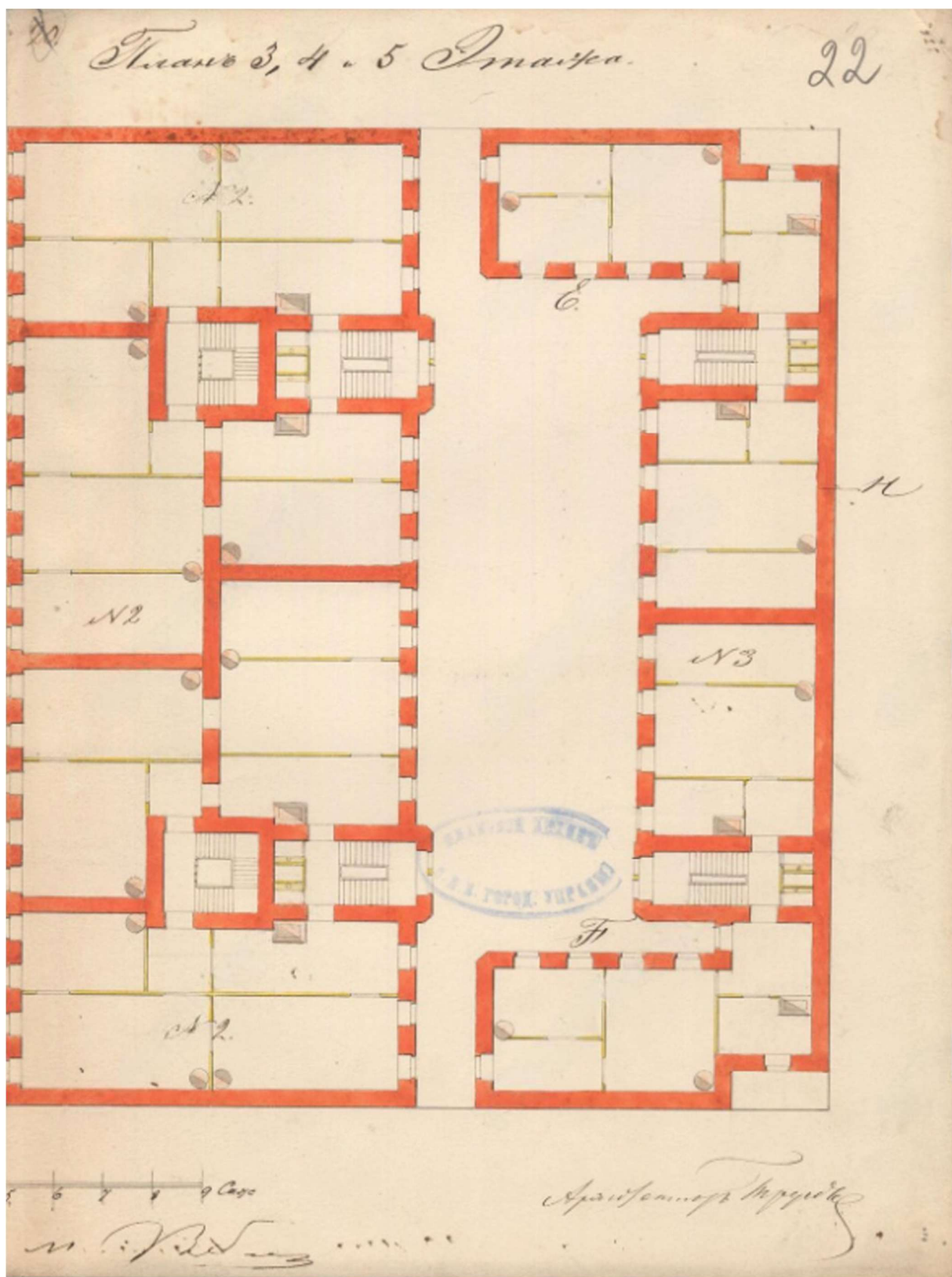
20. План 3, 4 и 5 этажей. 1860 г. // Источник: ЦГИА СПб Ф.513 Оп.102 Д.1577 Л.22.
