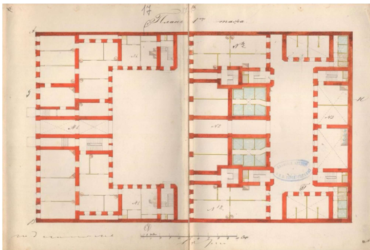
17. План 1-го этажа. 1860 г. // Источник: ЦГИА СПб Ф.513 Оп.102 Д.1577 Л.17-18.
