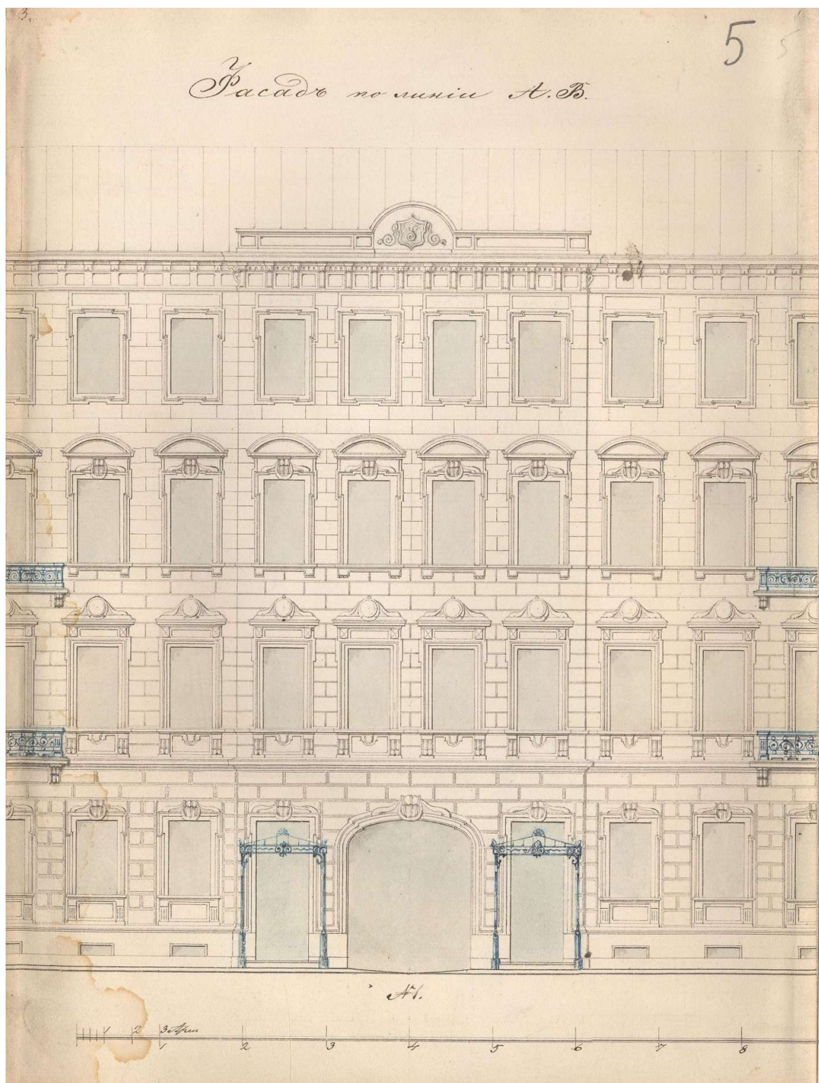
10.2. Фасад по линии АБ. 1860 г. // Источник: ЦГИА СПб Ф.513 Оп.102 Д.1577 Л.5.
