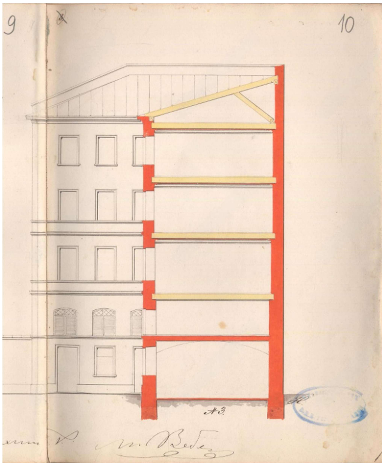
13. Разрез по ПН. 1860 г. // Источник: ЦГИА СПб Ф.513 Оп.102 Д.1577 Л.9-10.
