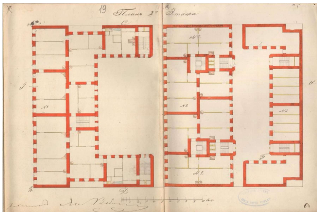
18. План 2-го этажа. 1860 г. // Источник: ЦГИА СПб Ф.513 Оп.102 Д.1577 Л.19-20.
