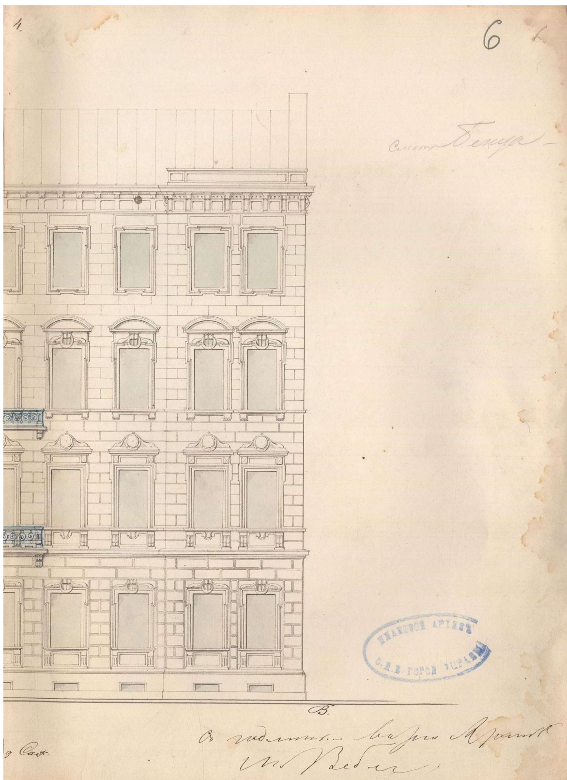
10.3. Фасад по линии АБ. 1860 г. // Источник: ЦГИА СПб Ф.513 Оп.102 Д.1577 Л.6.
