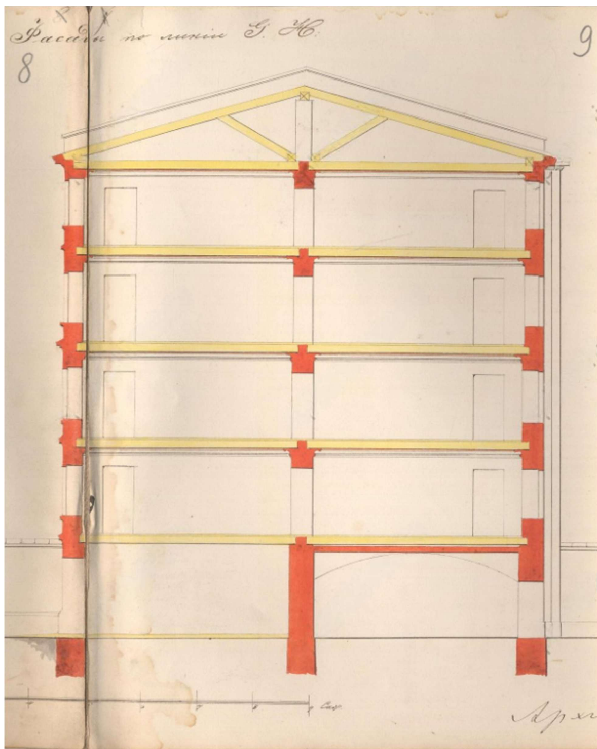
12. Разрез по линии ИИ. 1860 г. // Источник: ЦГИА СПб Ф.513 Оп.102 Д.1577 Л.8-9.
