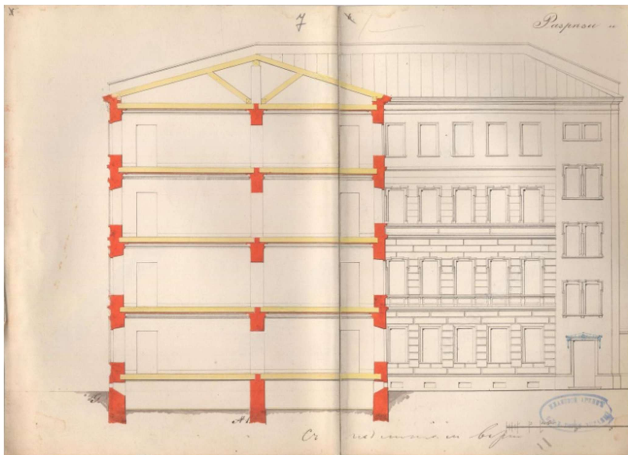
11.Разрез. 1860 г. // Источник: ЦГИА СПб Ф.513 Оп.102 Д.1577 Л.7-8.
