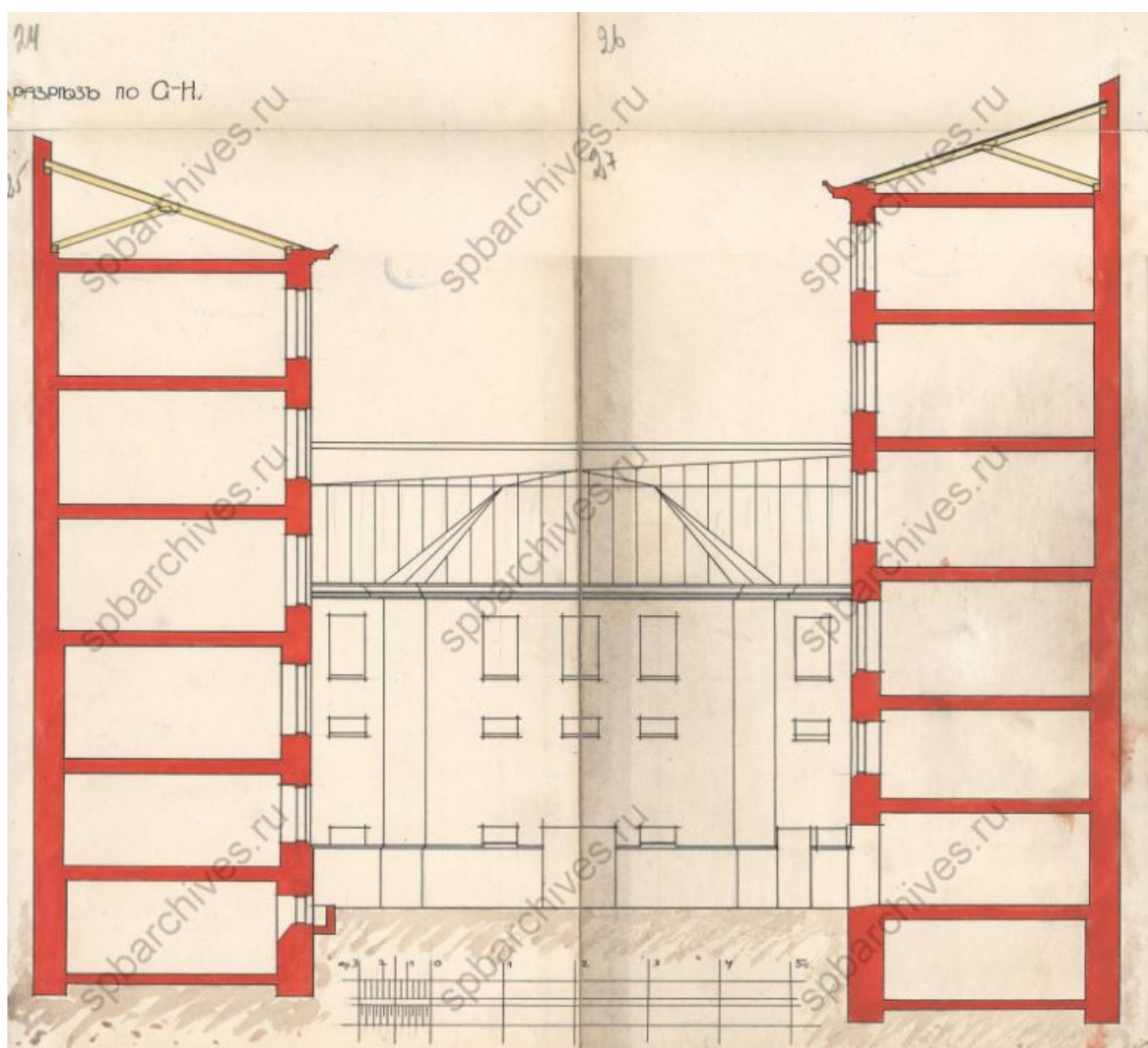
32. Разрез по линии G-H. ЦГИА СПб. Фонд 513. Опись 102. Дело 5093
