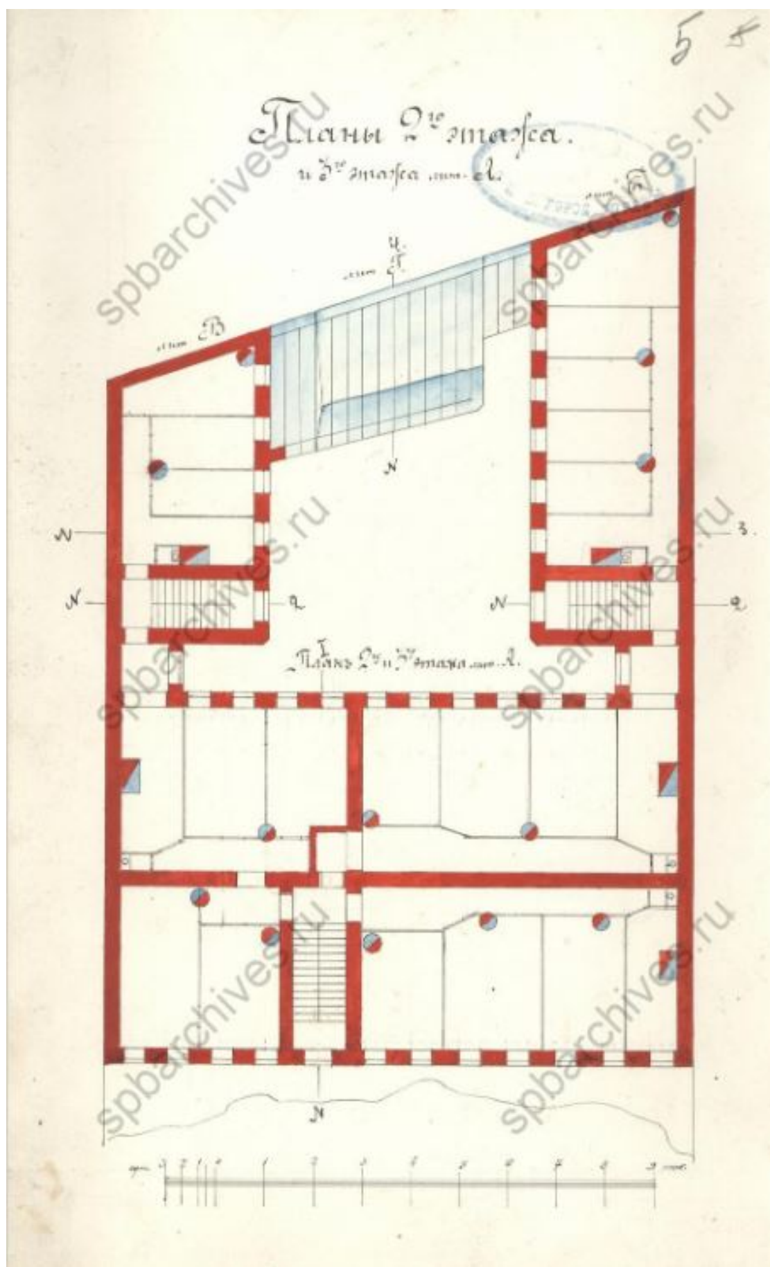
23. План 2-го этажа. ЦГИА СПб. Фонд 513. Опись 102. Дело 5093
