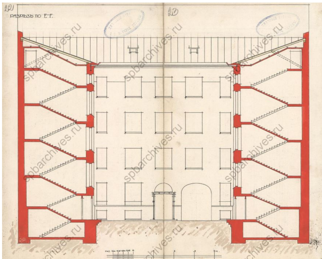
31. Разрез по линии ЕФ. ЦГИА СПб. Фонд 513. Опись 102. Дело 5093
