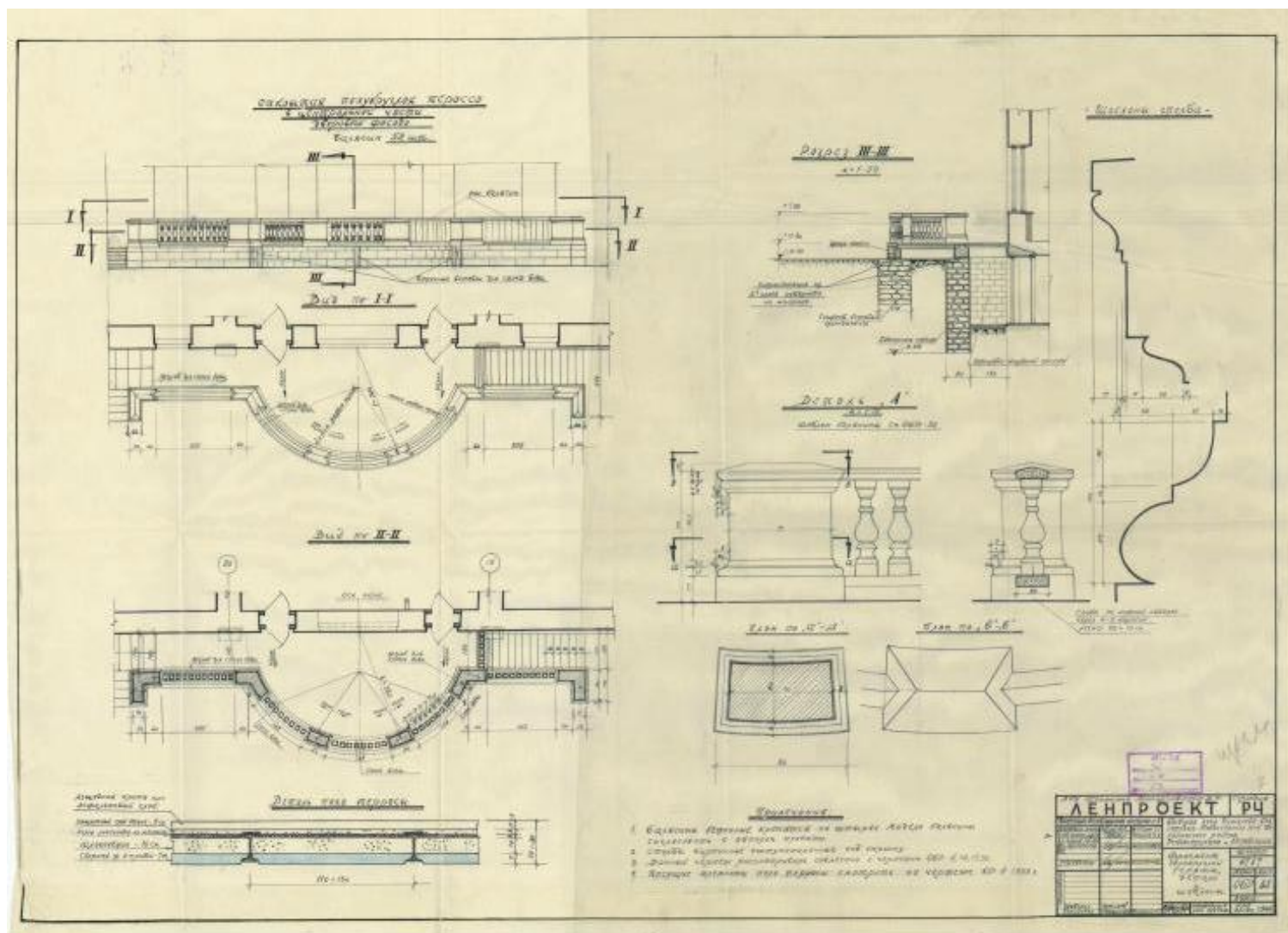
Илл. 27. Проект реставрации. Крыльцо центрального корпуса со стороны парка. 1965 г. Автор – архитектор Шерстнев. ЦГА НТД ф. 36 о. 3-4 д. 53 л. 7
