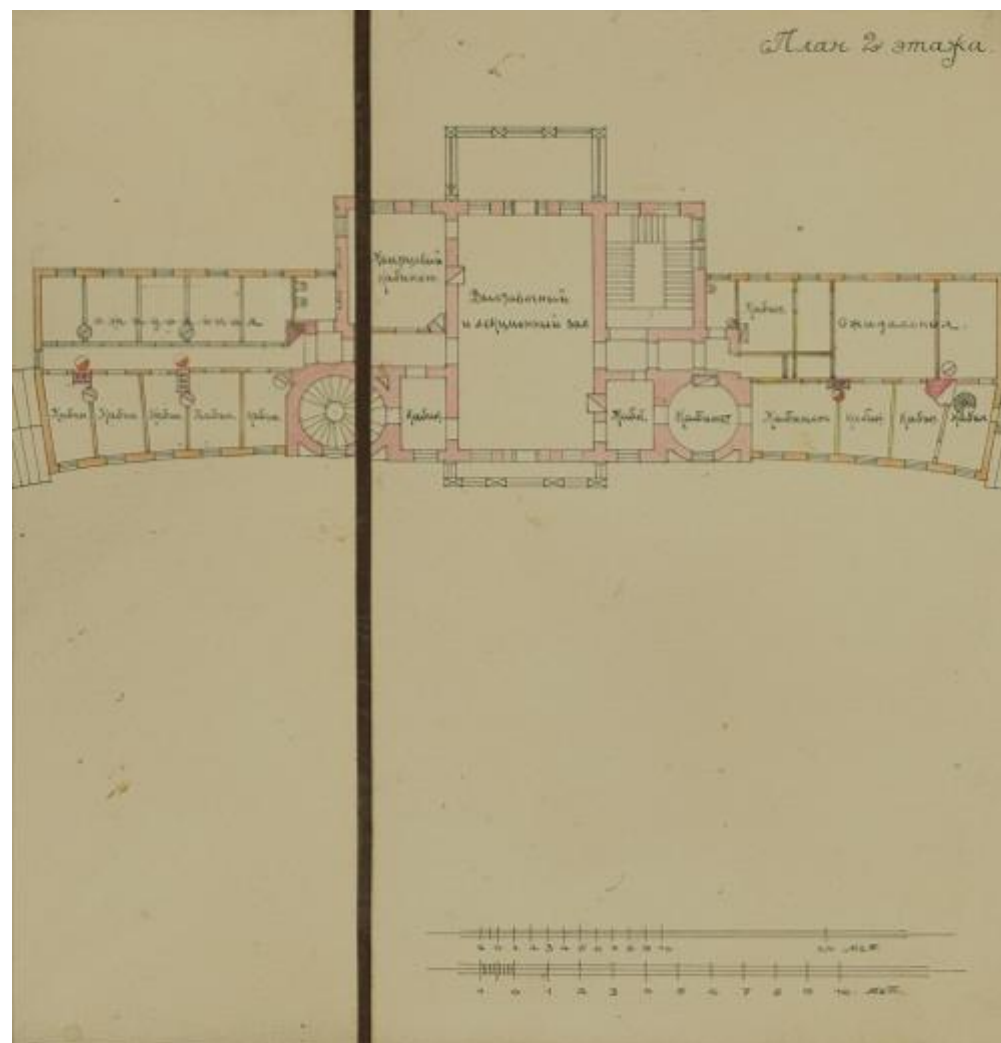
Илл. 23. Проект перепланировки 1927 г. Средняя часть 2-го этажа. ЦГА НТД ф. 192 о. 3-1 д. 3224 д. 9
