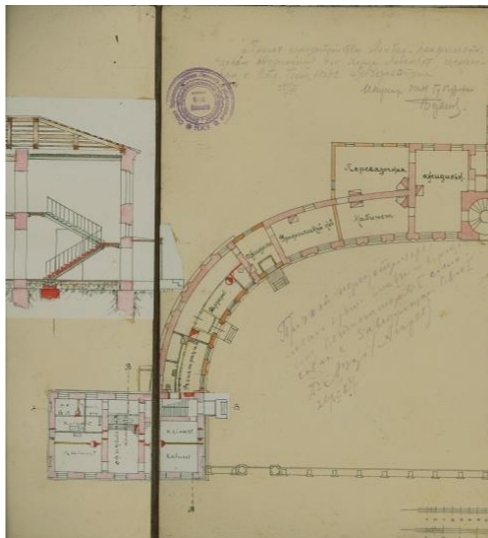
Илл. 19. Проект перепланировки 1927 г. Разрез западного павильона и западная часть 1-го этажа. ЦГА НТД ф. 192 о. 3-1 д. 3224 д. 9
