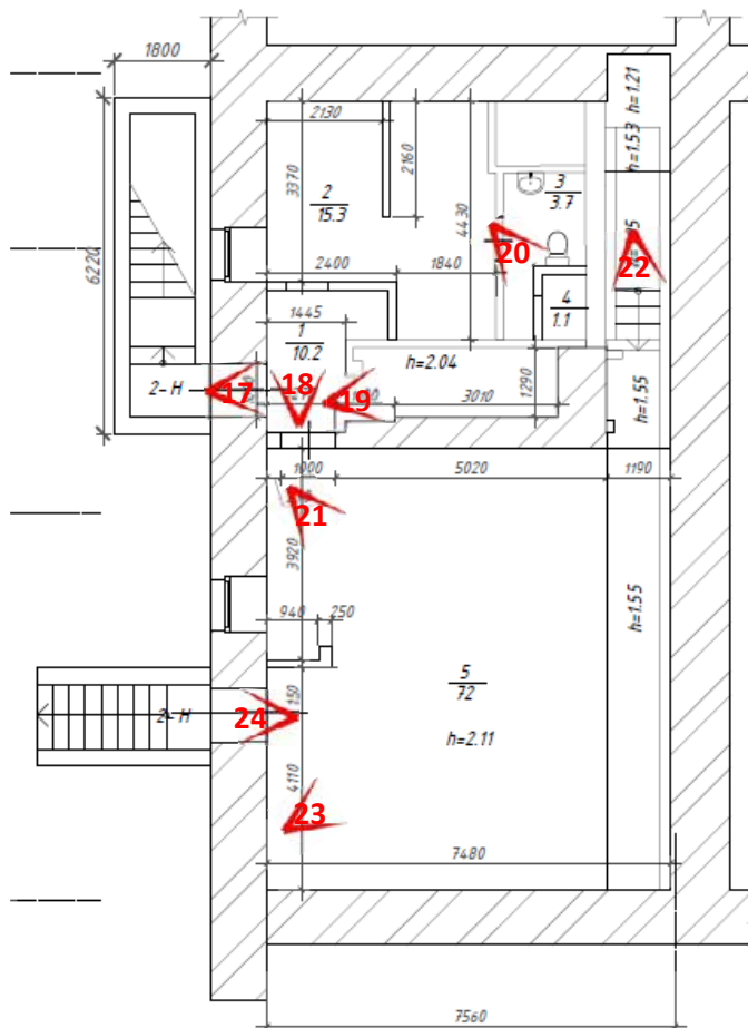
Рисунок 3.Схема фотофиксации на фрагменте плана цокольного этажа, пом. 2-Н
