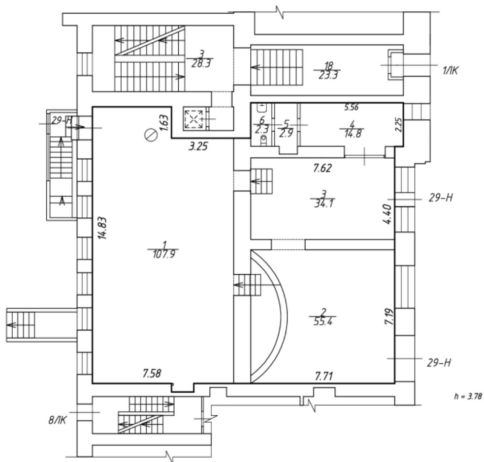
фрагмент Плана 1 этажа, 1ЛК, 8ЛК
