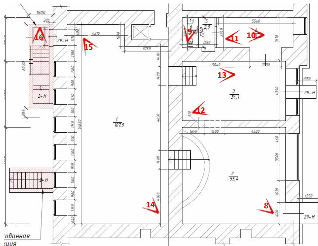
Рисунок 2.Схема фотофиксации на фрагменте плана цокольного этажа, пом. 29-Н
