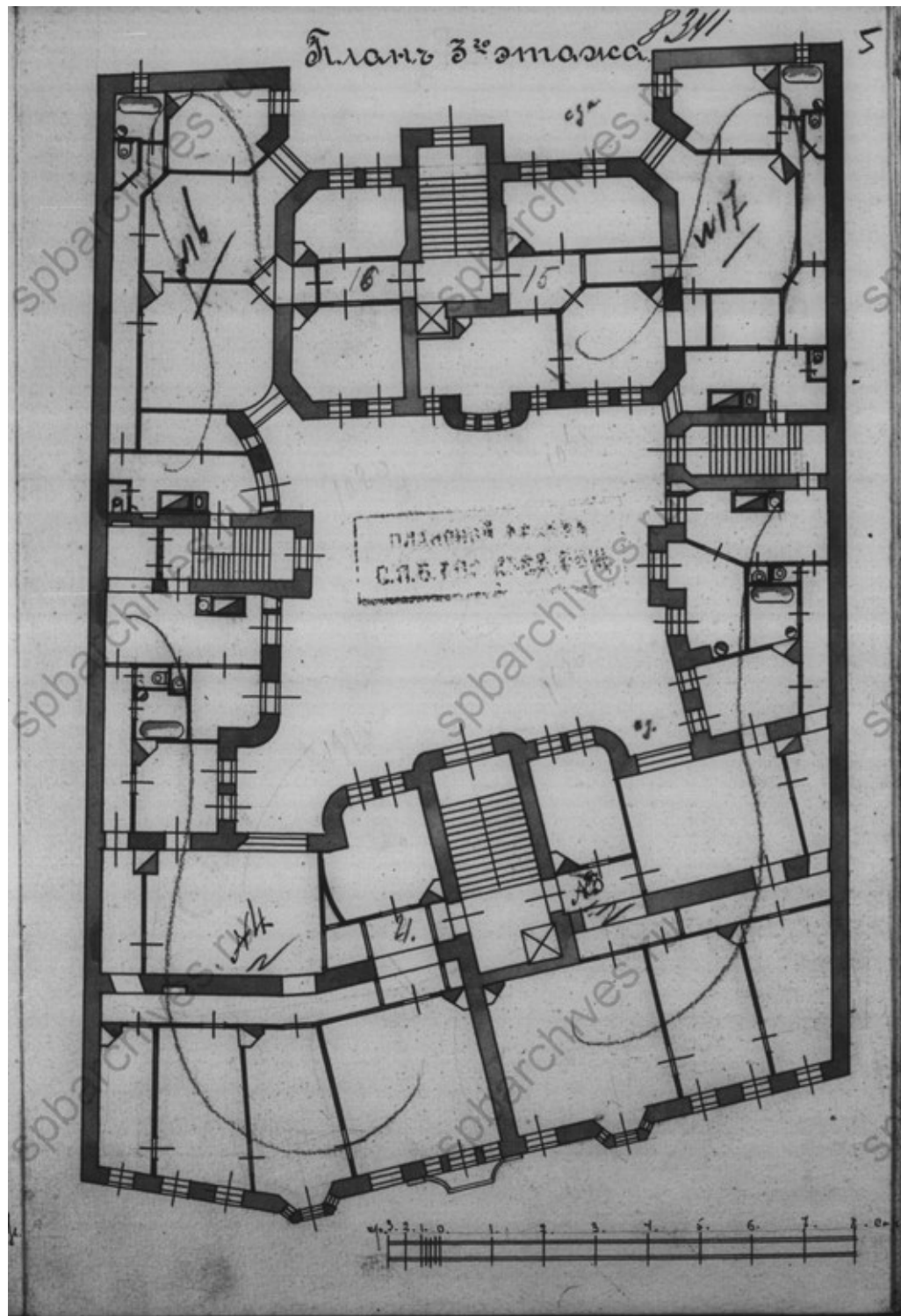
Илл. 5. План 3-го этажа. 1913 гг. ЦГИА СПб. Ф. 515. Оп. 4. Д. 3921. Л. 5.
