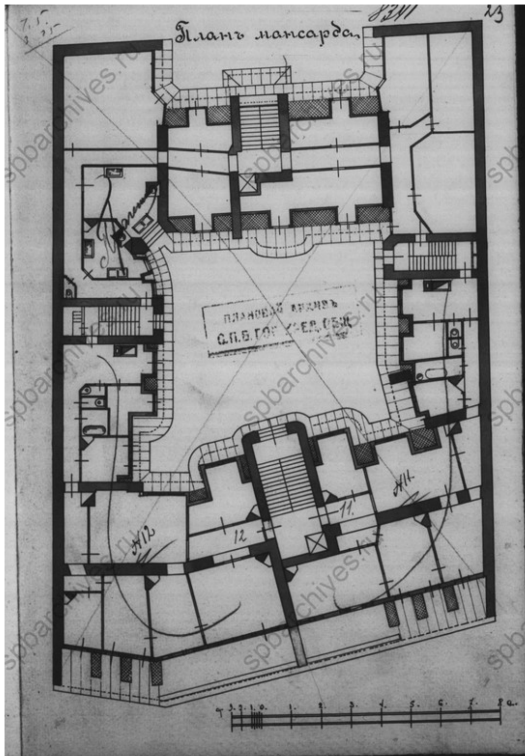
Илл. 9. План мансарда. 1913 гг. ЦГИА СПб. Ф. 515. Оп. 4. Д. 3921. Л. 23.
