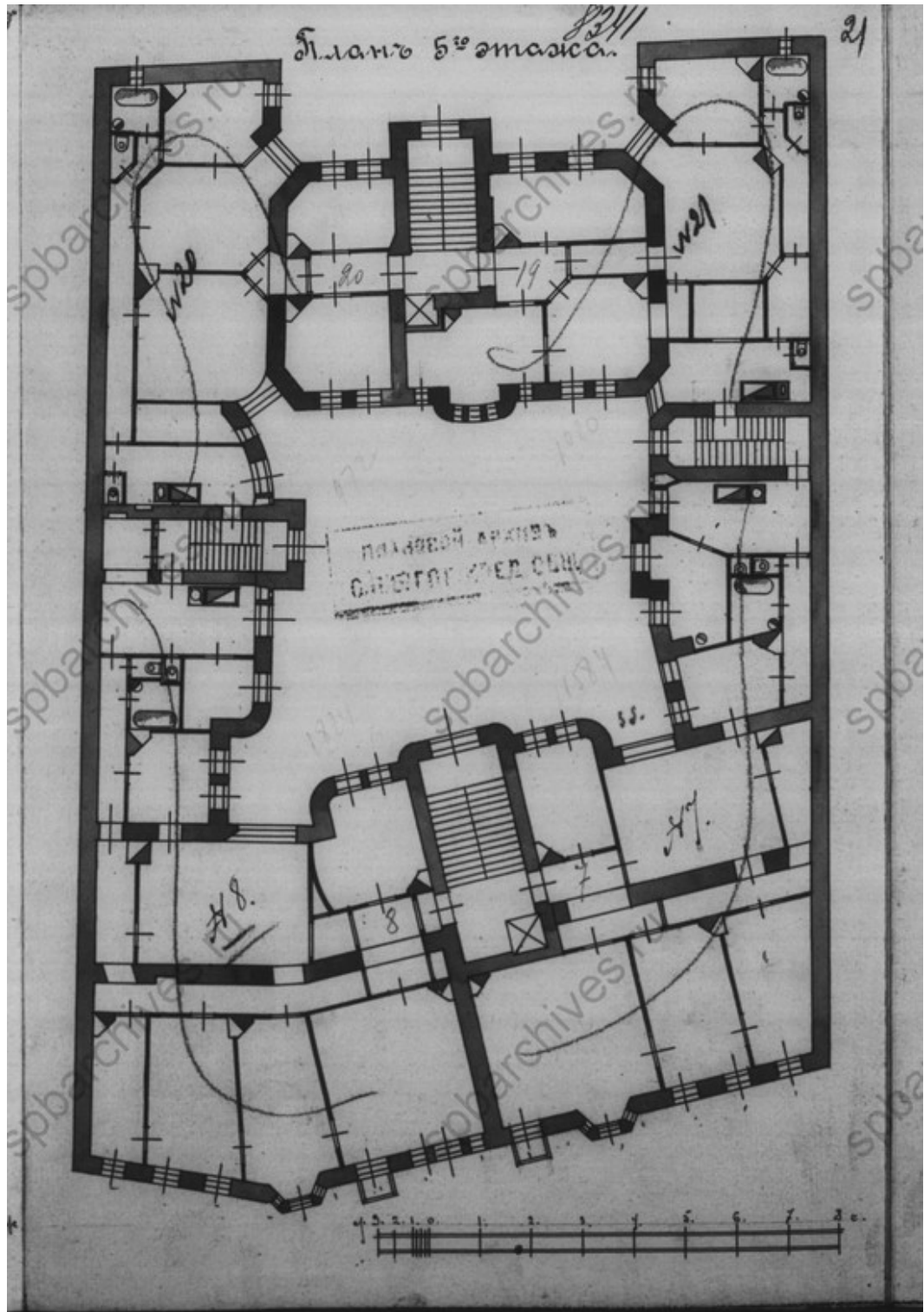
Илл. 7. План 5-го этажа. 1913 гг. ЦГИА СПб. Ф. 515. Оп. 4. Д. 3921. Л. 21.
