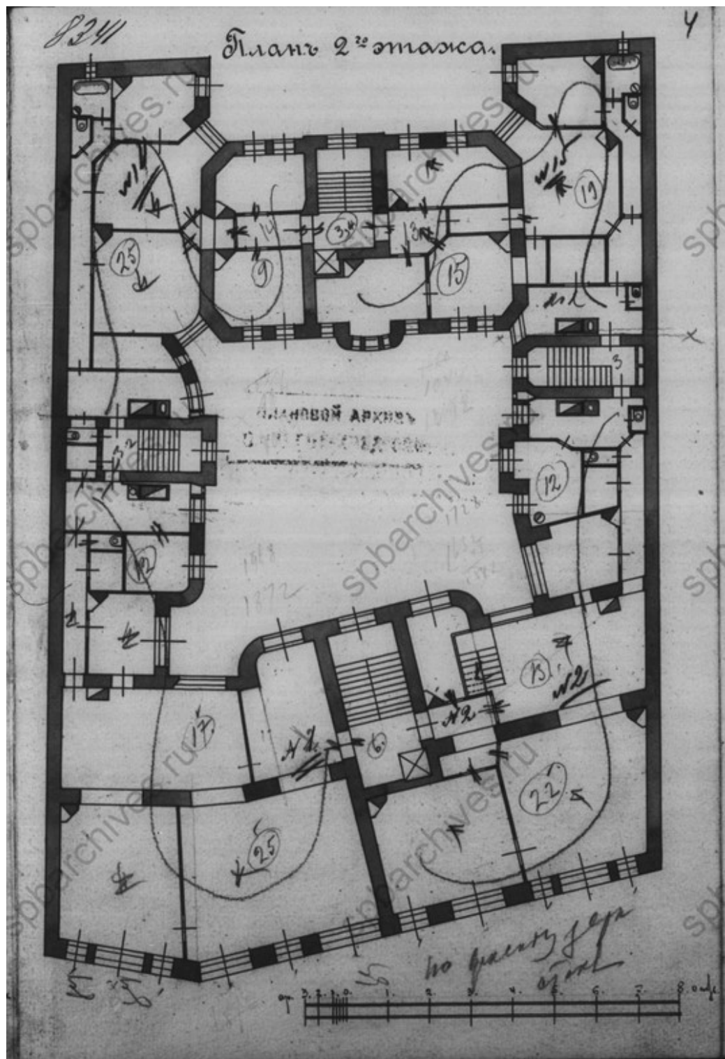
Илл. 4. План 2-го этажа. 1913 гг. ЦГИА СПб. Ф. 515. Оп. 4. Д. 3921. Л. 4.
