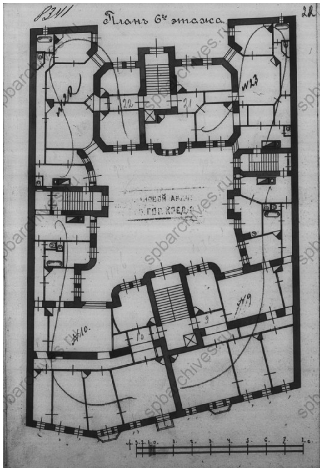
Илл. 8. План 6-го этажа. 1913 гг. ЦГИА СПб. Ф. 515. Оп. 4. Д. 3921. Л. 22.
