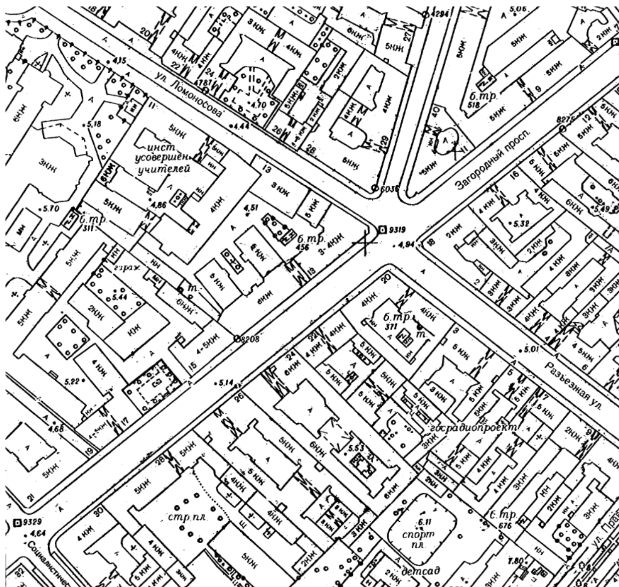
59. Топосъемка 1991 г. Планшет 2429-12.
