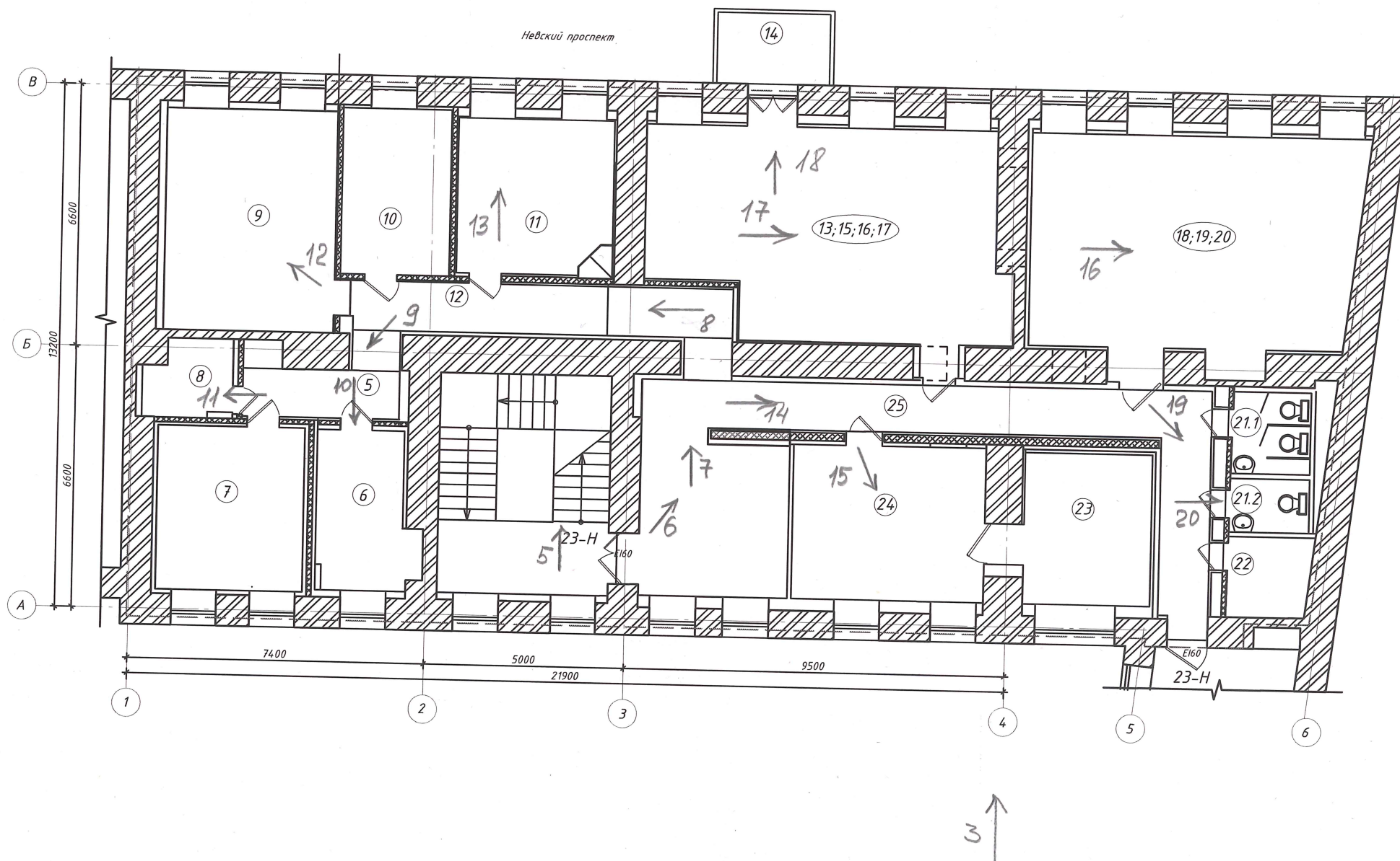
Фрагмент плана 2 этажа помещение 23-Н
