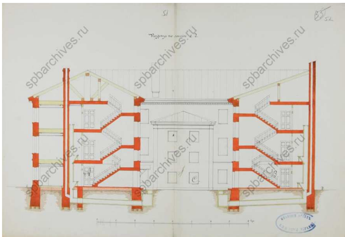
51. Разрез по линии сд. ЦГИА СПб. Фонд 513. Опись 102. Дело 1568
