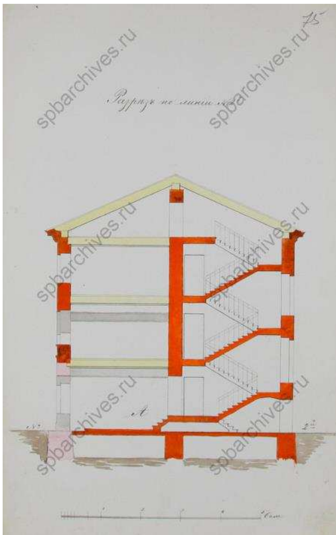
64. Разрез по линии № 2. ЦГИА СПб. Фонд 513. Опись 102. Дело 1568
