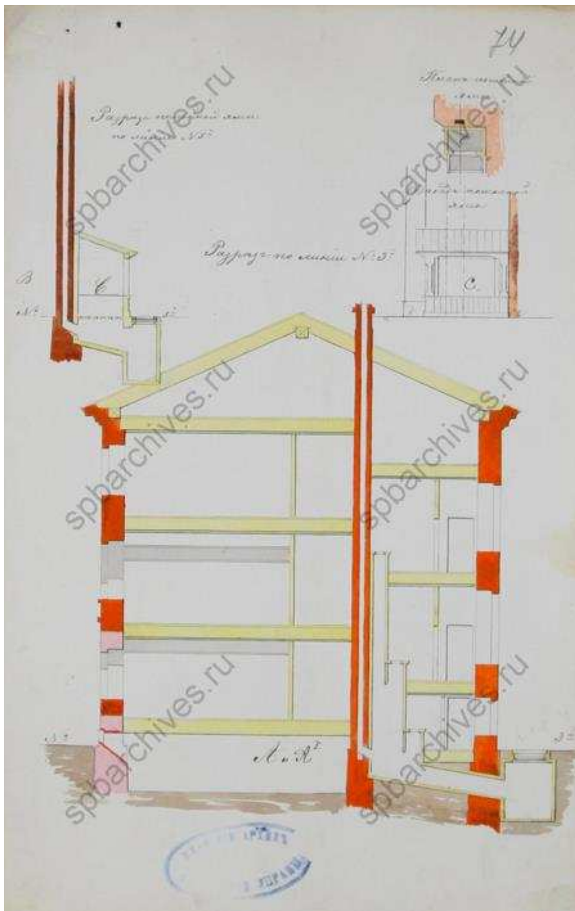
63. Разрез по линии № 3 и фрагмент плана. ЦГИА СПб. Фонд 513. Опись 102. Дело 1568
