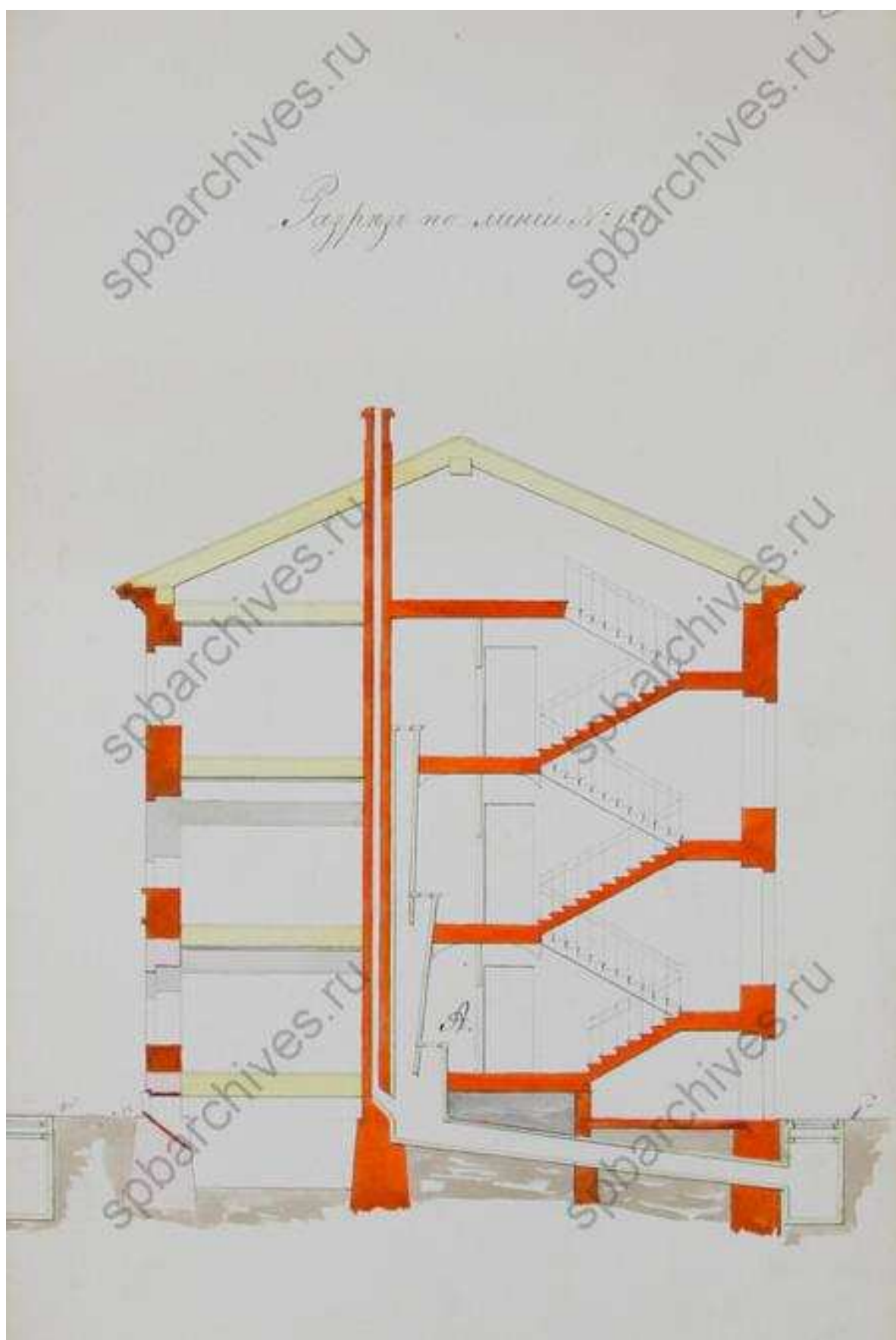
65. Разрез по линии № 1. ЦГИА СПб. Фонд 513. Опись 102. Дело 1568
