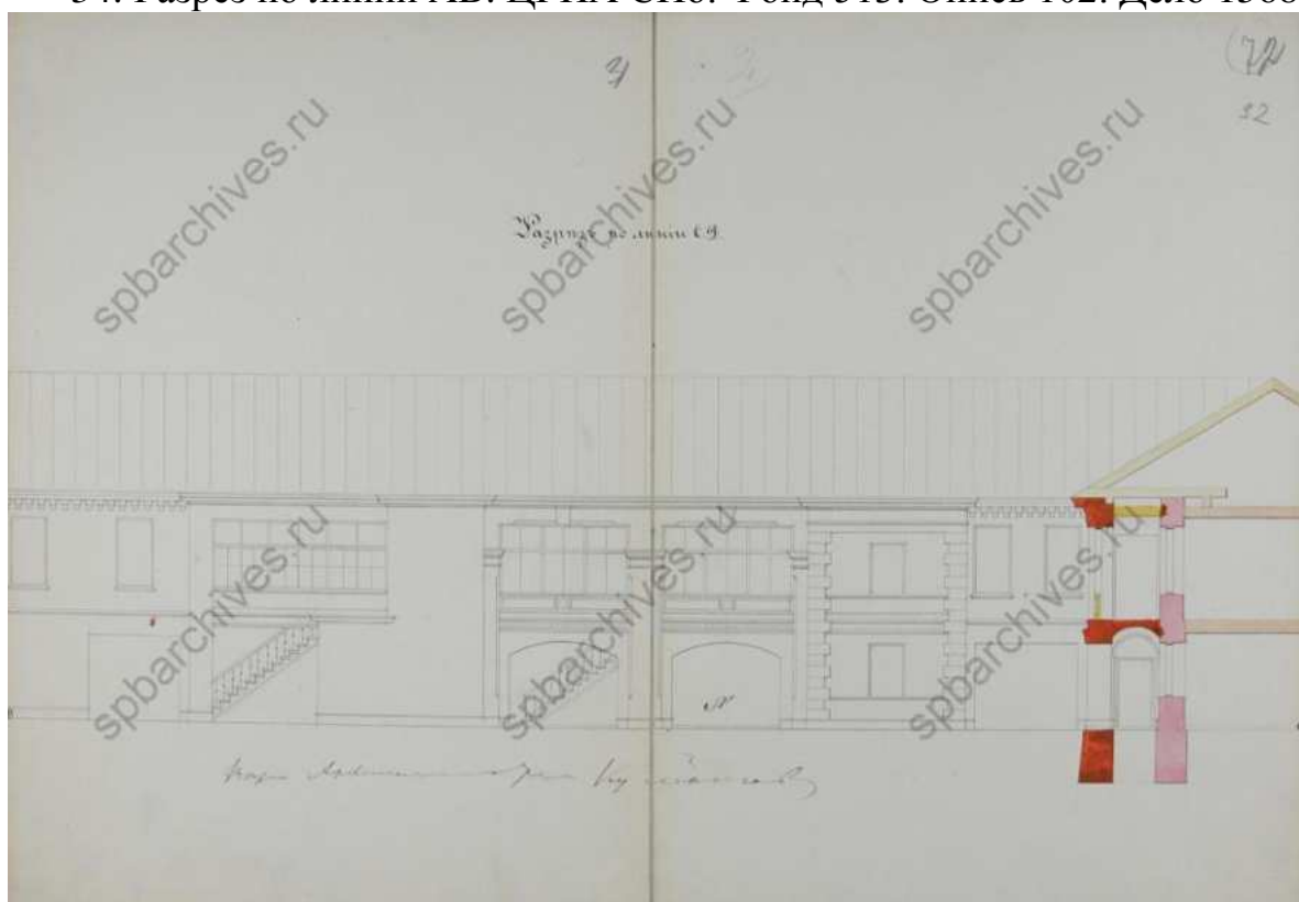
35. Разрез по линии СД. ЦГИА СПб. Фонд 513. Опись 102. Дело 1568
