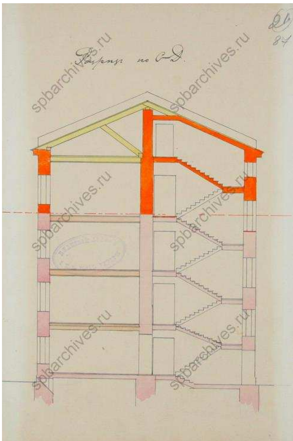
75. Разрез по линии CD. ЦГИА СПб. Фонд 513. Опись 102. Дело 1568
