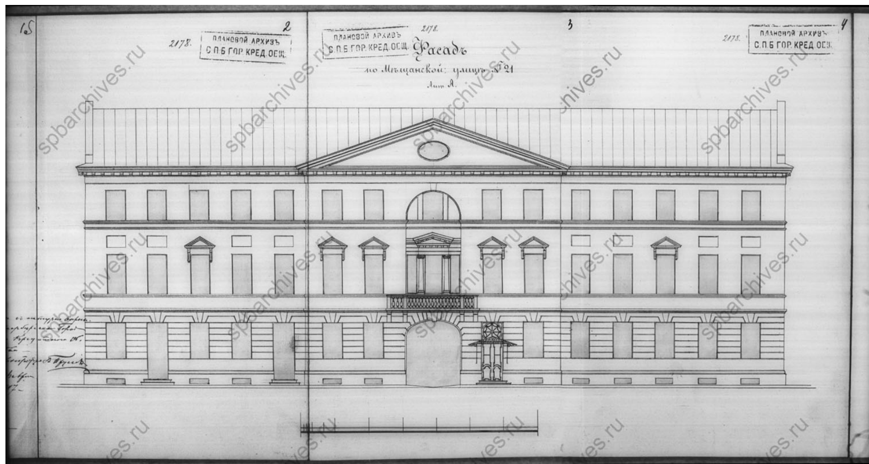
Илл. 9. Фасад по Мещанской улице №21. 1897 г. ЦГИА СПб. Фонд 515, опись 4, дело 802, листы 2, 3, 4.
