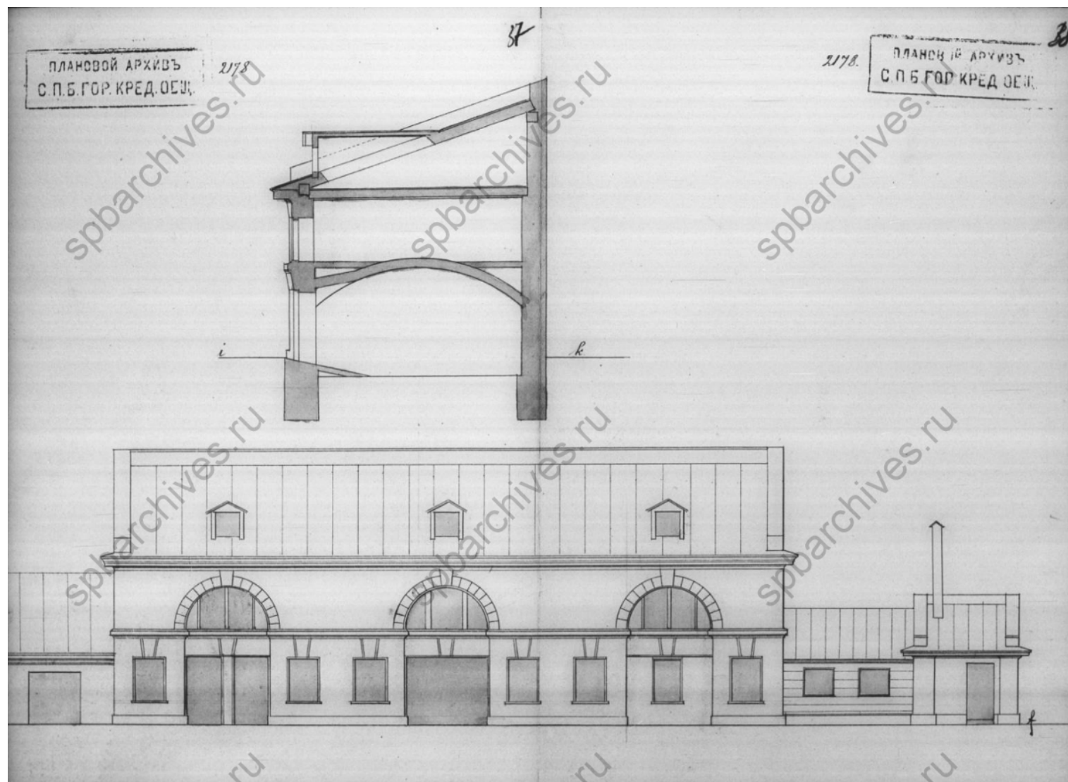
Илл. 19. Фасады и разрезы по левой стороне двора по линии е-ф. 1897 г. ЦГИА СПб. Фонд 515, опись 4, дело 802, листы 37, 38.
