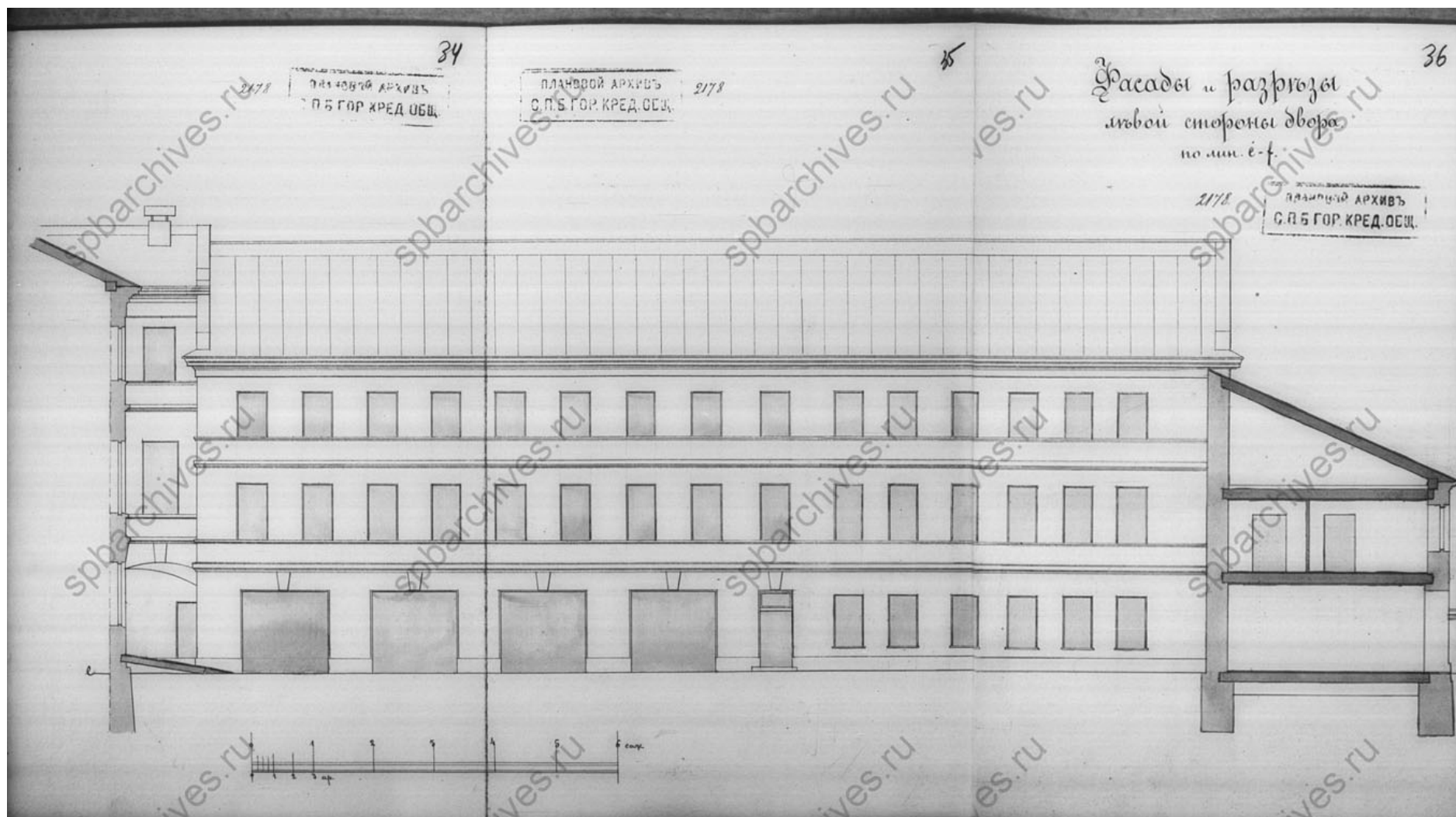
Илл. 18. Фасады и разрезы по левой стороне двора по линии е-ф. 1897 г. ЦГИА СПб. Фонд 515, опись 4, дело 802, листы 34, 35, 36.
