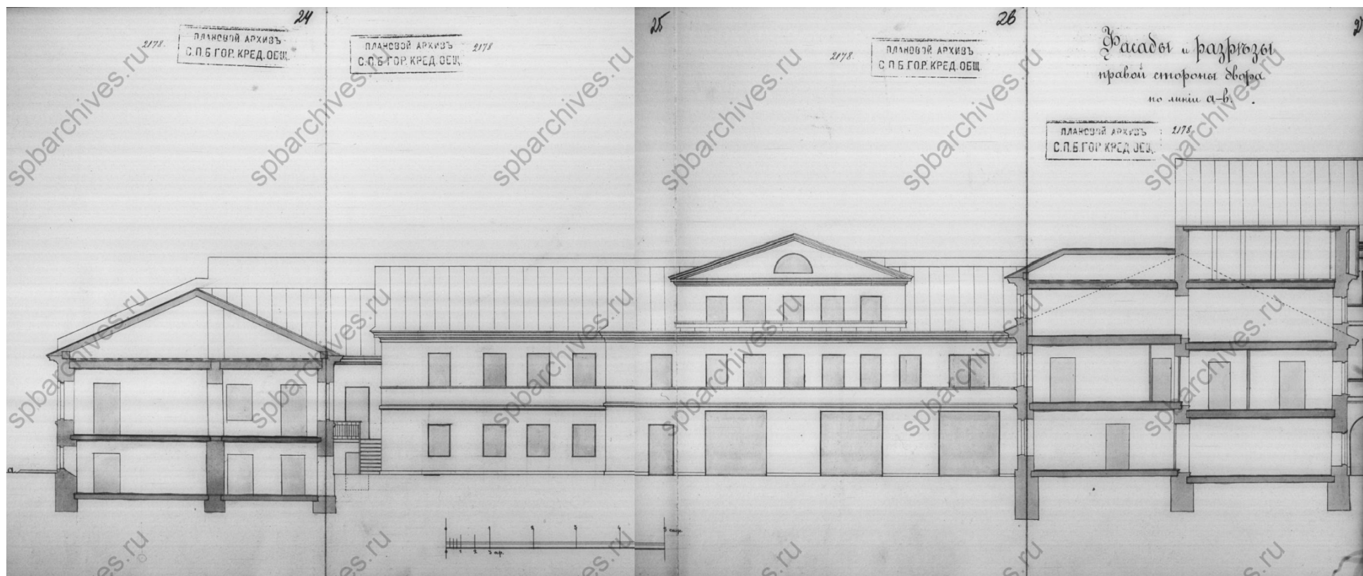
Илл. 15. Фасады и разрез по правой стороне двора по линии а-в. 1897 г. ЦГИА СПб. Фонд 515, опись 4, дело 802, листы 24-27.
