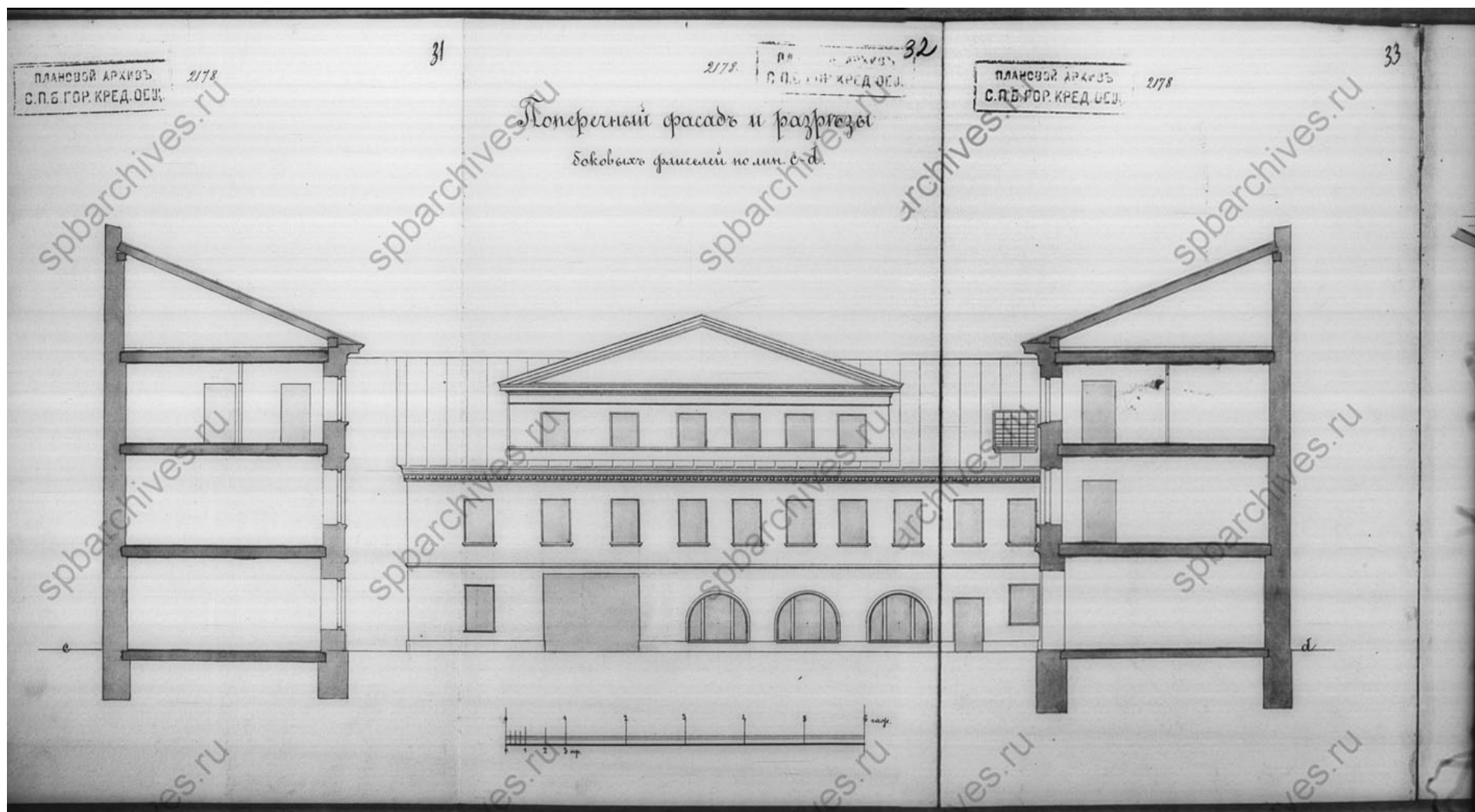
Илл. 17. Поперечный фасад и разрезы боковых флигелей по линии с-д. 1897 г. ЦГИА СПб. Фонд 515, опись 4, дело 802, листы 31, 32, 33.
