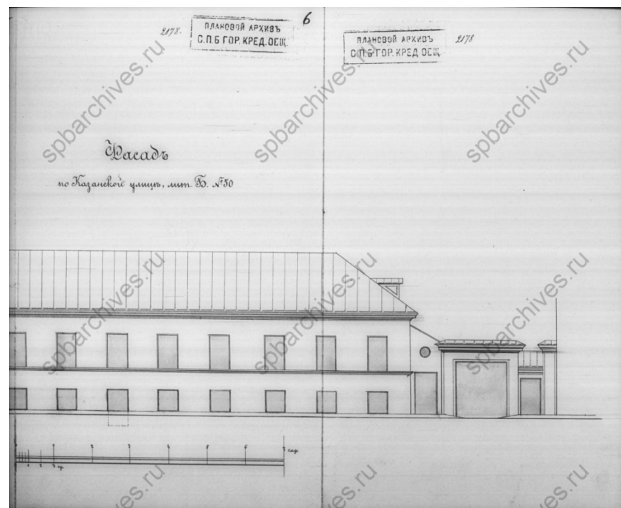
Илл. 10. Фасад по Казанской улице, лит. Б №50. 1897 г. ЦГИА СПб. Фонд 515, опись 4, дело 802, листы 5, 6, 7.
