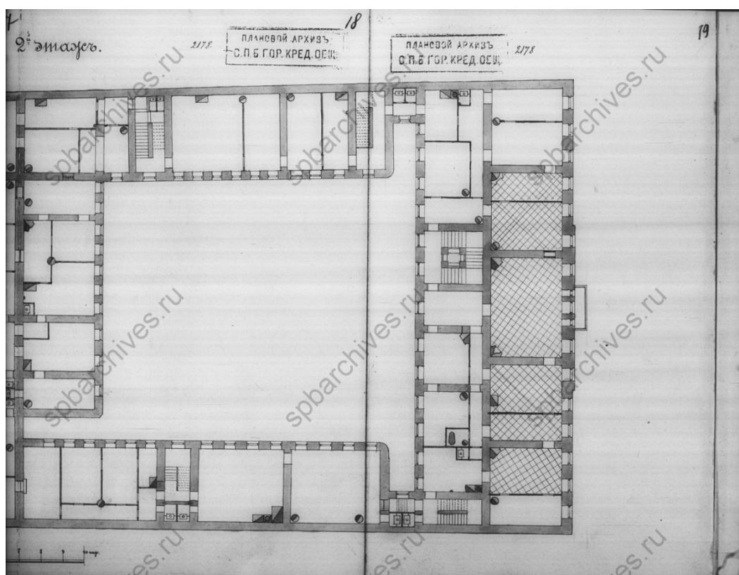
Илл. 13. 2-й этаж. 1897 г. ЦГИА СПб. Фонд 515, опись 4, дело 802, листы 16-19.
