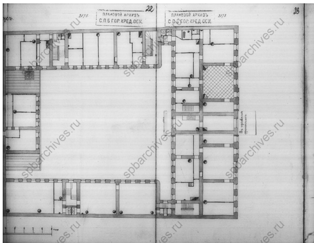
Илл. 14. 3-й этаж. 1897 г. ЦГИА СПб. Фонд 515, опись 4, дело 802, листы 20-23.
