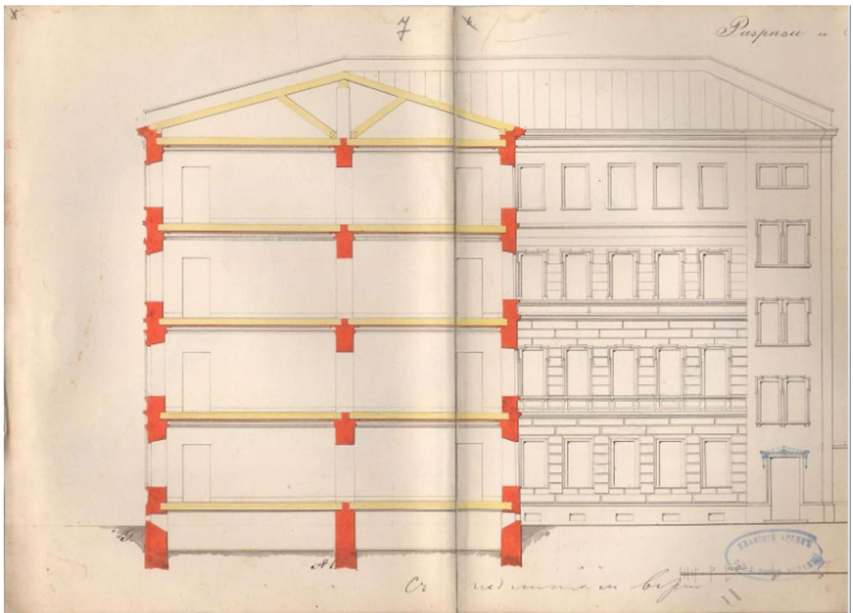
11.Разрез. 1860 г. // Источник: ЦГИА СПб Ф.513 Оп.102 Д.1577 Л.7-8.
