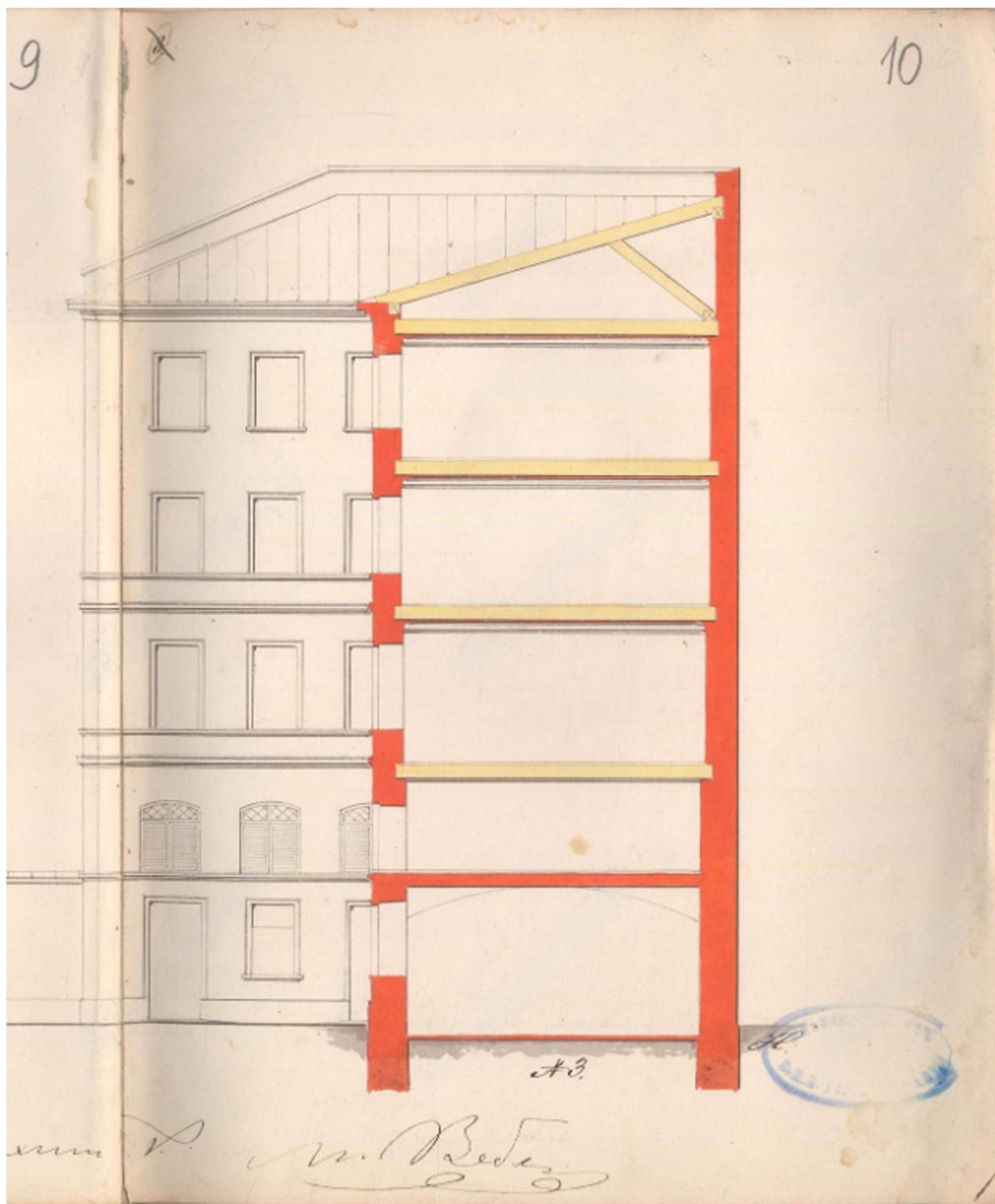
13. Разрез по И. 1860 г. // Источник: ЦГИА СПб Ф.513 Оп.102 Д.1577 Л.9-10.
