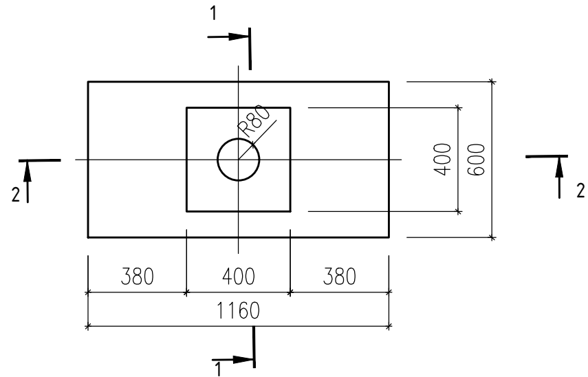
Фундамент Ф1
