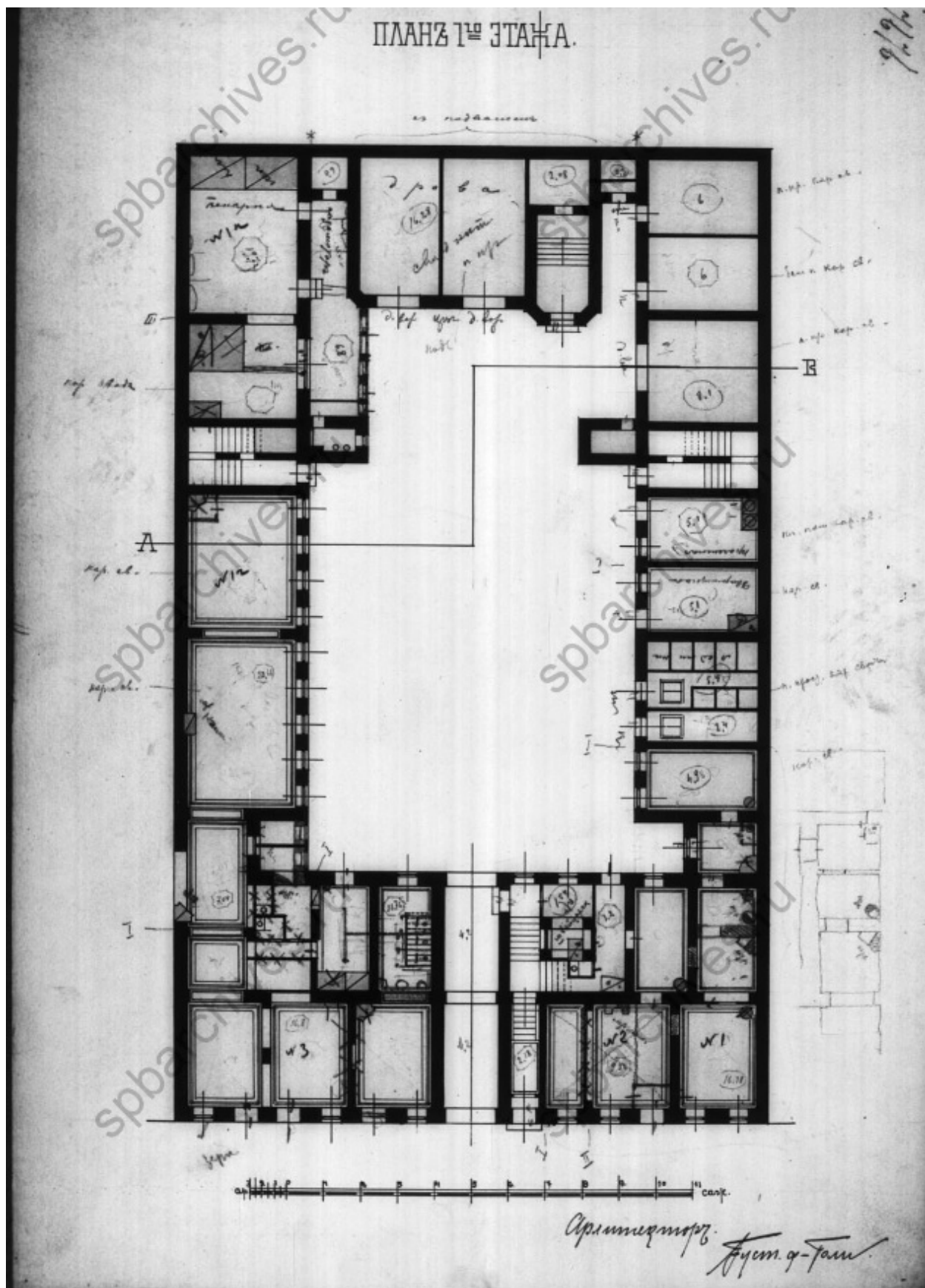
51. План 1-го этажа дома Фольборта Адмиралтейской части, 1-го участка, по Невскому пр., № 6. 1904 г. ЦГИА СПб. Ф. 515. Оп. 4. Д. 3882. Л. 3.
