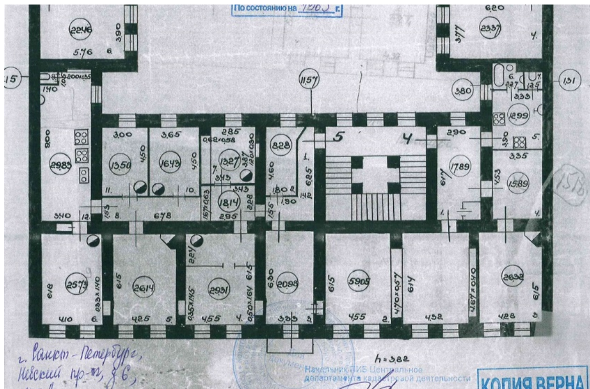
72. План 2 этажа дома № 6 по Невскому проспекту. 1965 г. Филиал ГУП ГУИОН ПИБ Центрального района.
