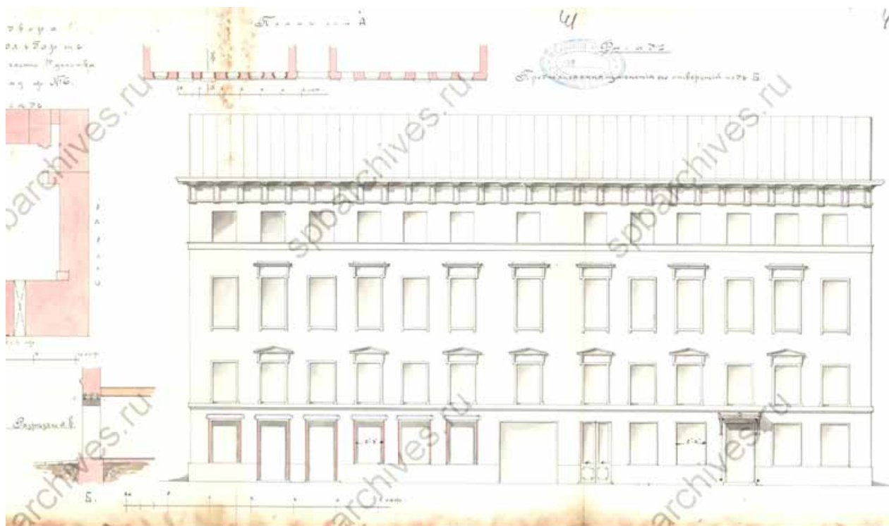
58. Лицевой фасад с показанием предполагаемых изменений дома во дворе наследников Фольборт Адмиралтейской части 1-го участка по Невскому пр., № 6. 1909 г. ЦГИА СПб. Ф. 513. Оп. 102. Д. 208. Лл. 40 об, 41, 42.
