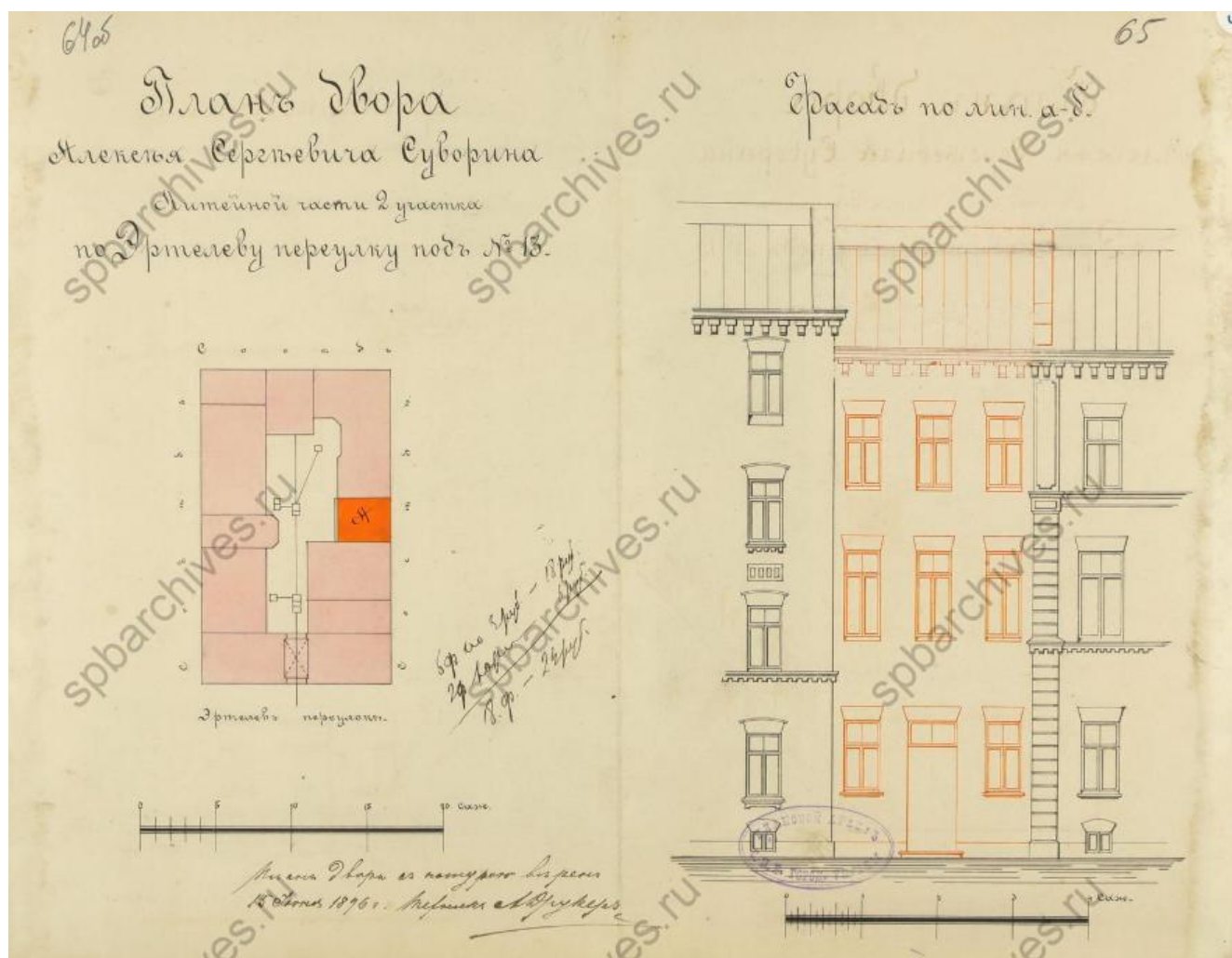
Илл. 32. План двора А.С. Суворина. Литейной части 2-го участка по Эртелеву пер. № 13. 1896 г. ЦГИА СПб. Ф. 513. Оп. 102. Д. 4589. Л. 64б-65.
