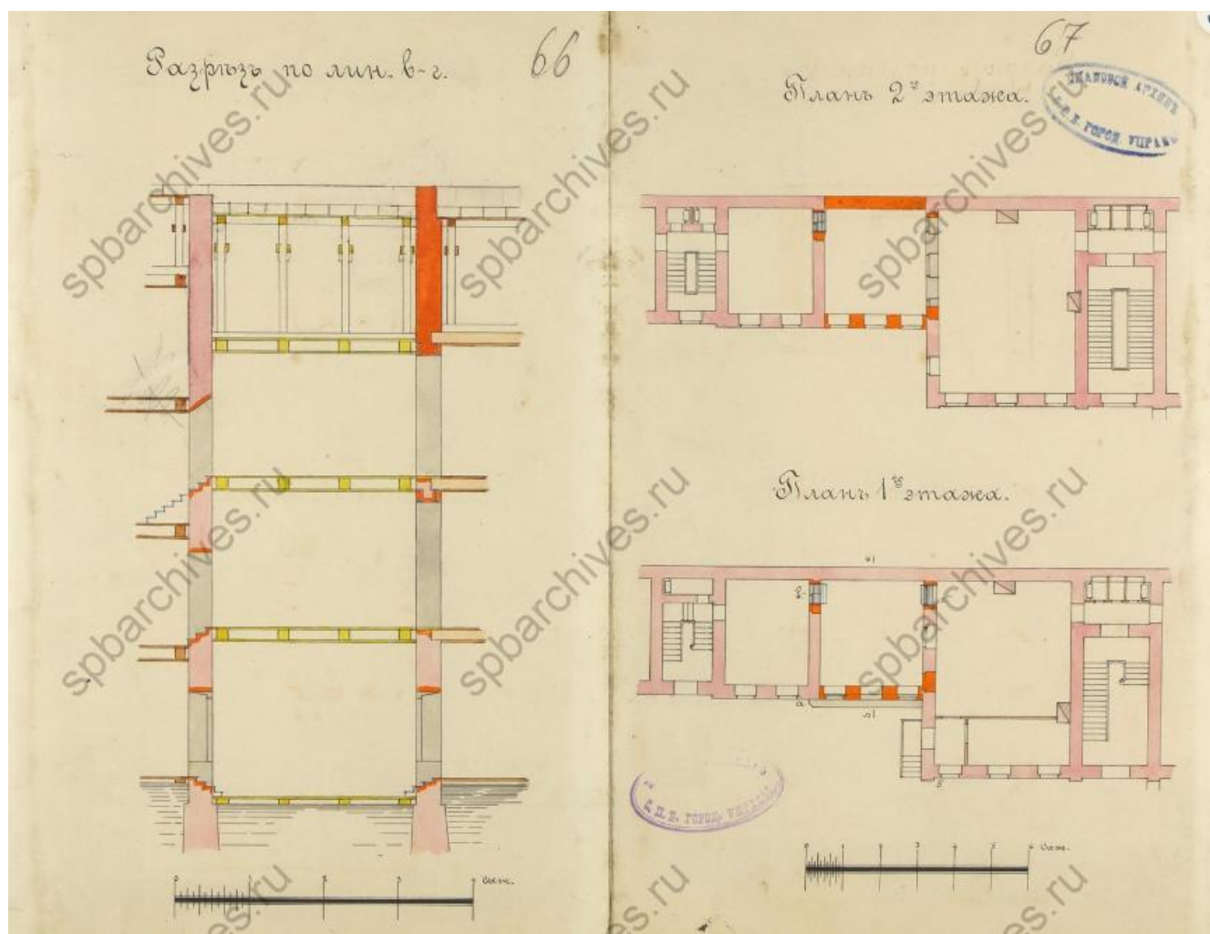
Илл. 33. План двора А.С. Суворина. Литейной части 2-го участка по Эртелеву пер. № 13. Поперечный разрез и поэтажные планы. 1896 г. ЦГИА СПб. Ф. 513. Оп. 102. Д. 4589. Л. 66-67.
