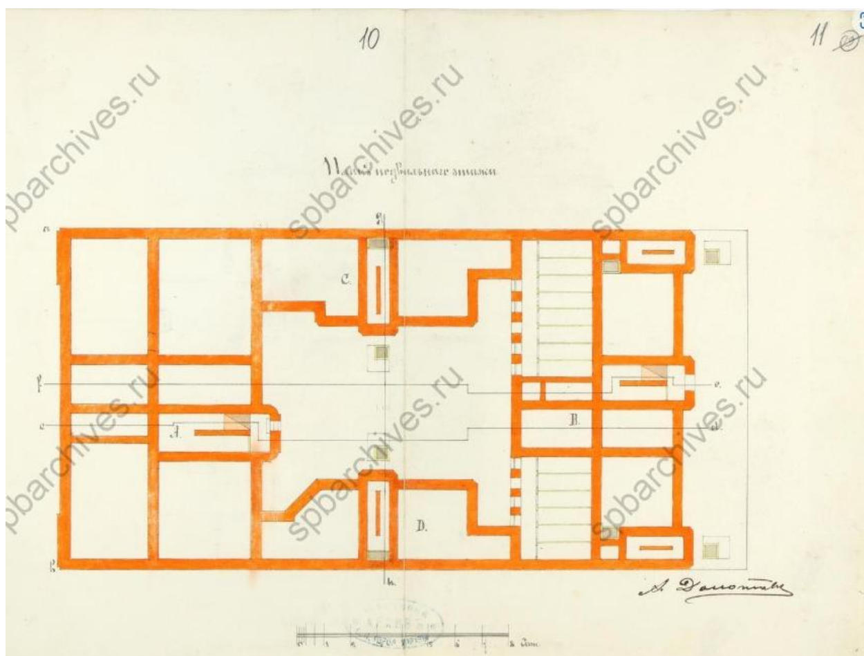
Илл. 13. Фасад дома по Эртелеву переулку под № 11. План подвального этажа. А. Долотов. 1876. ЦГИА СПб. Ф. 513. Оп. 102. Д. 4587. Л. 10-11.
