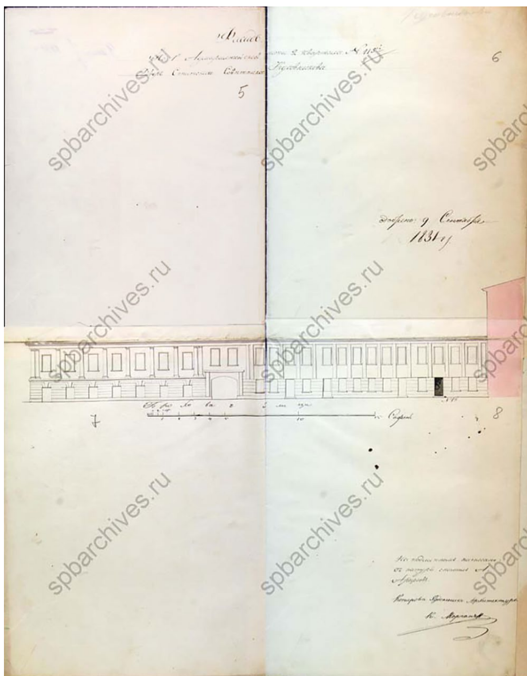
19. Фасад [по Гороховой ул.] по 1-й Адмиралтейской части 2-го квартала № 115. Двор статского советника Кусовникова. 1831 г. ЦГИА СПб. Ф. 513. Оп. 102. Д. 151. Л. 5-8.
