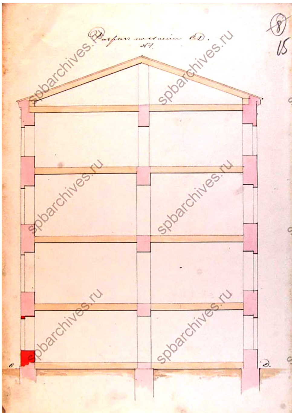
24. Разрез по линии сд. № 1. Арх. Н. В. Трусов. 1866 г. ЦГИА СПб. Ф. 513. Оп. 102. Д. 151. Л. 15.
