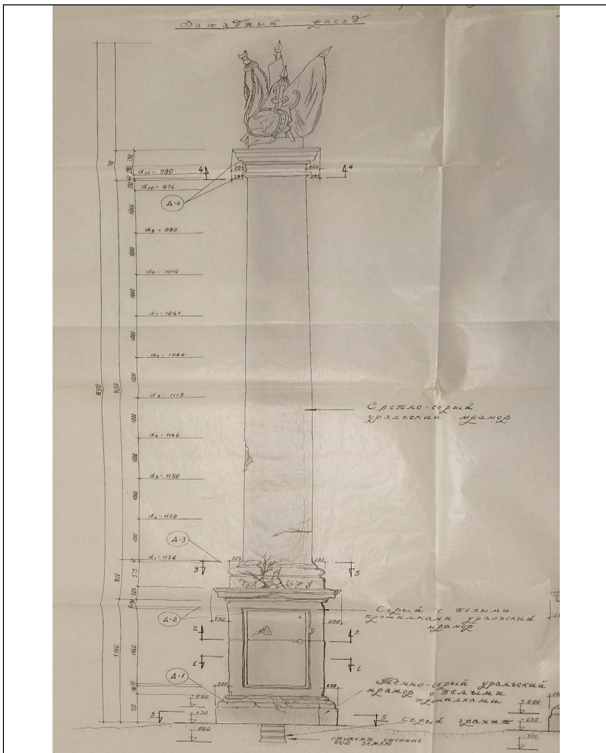
6. Обмерный чертеж западного фасада. Совмещенный обмер и проект реставрации Крымской колонны, 1983 г. ЦГАНТД СПб. Ф.Р-488. Оп.325. Д.590. Л.1.
