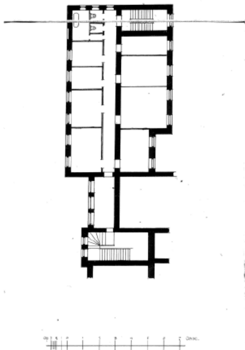
7. План 3-го этажа особняка В.П. Кочубя. Проект. Арх. А. Таманов (Таманян). 1911 г. РГИА Ф. 971. Оп. 1. Д. 72.
