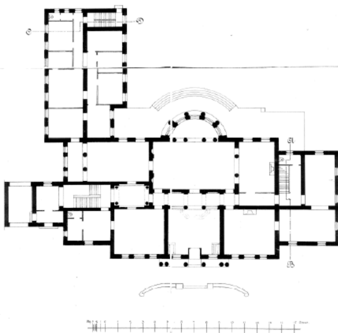
5. План 1-го этажа особняка В.П. Кочубея.
