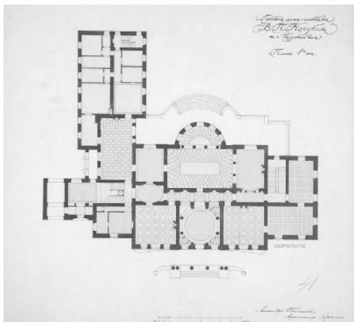
15. Проект раскладки паркета в 1-м этаже особняка В.П. Кочубей. Арх. А.Таманов. 1912 г. ГМЗ «Царское Село», ЕД – 2189-ХІІІ.
