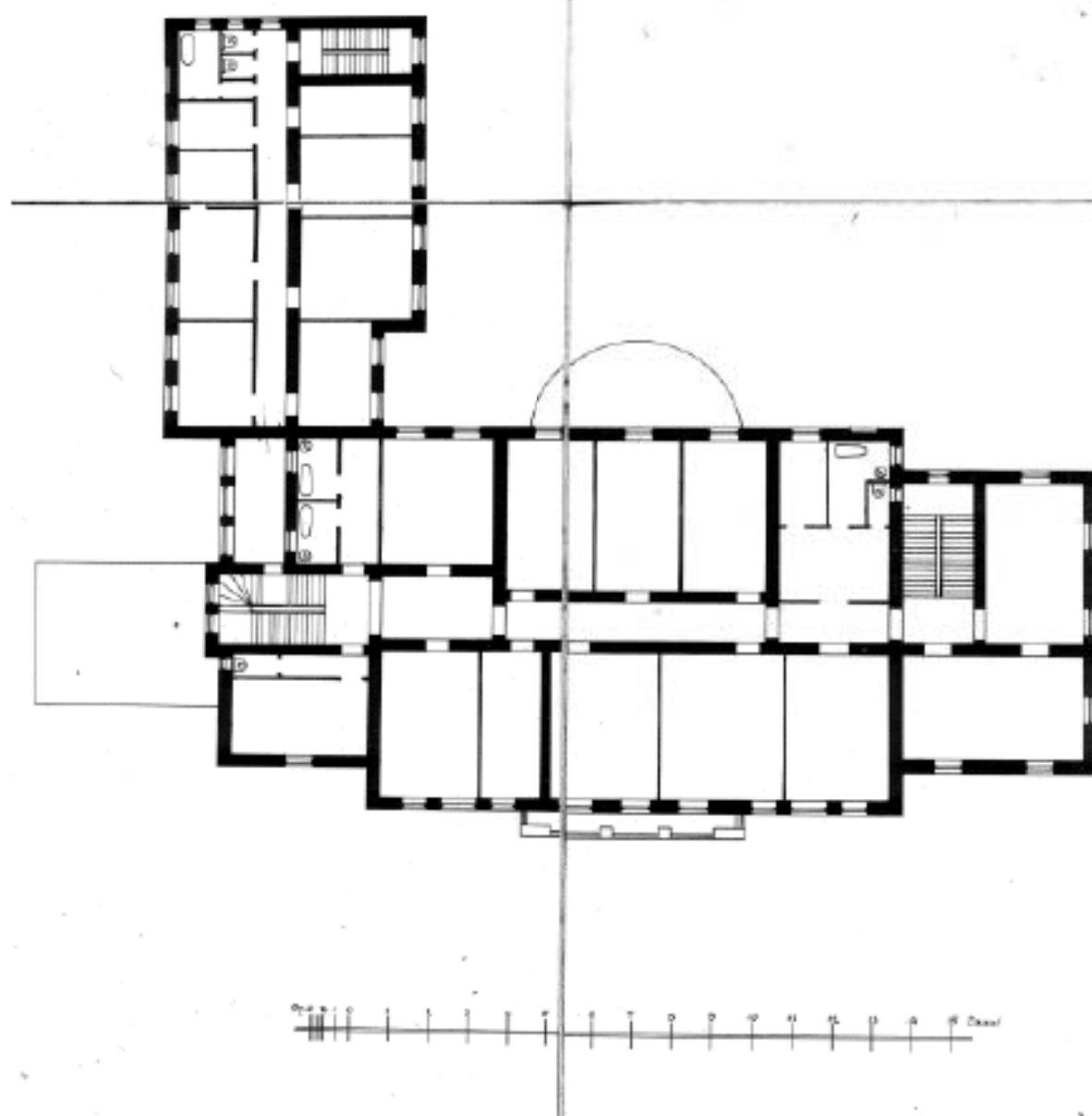
6. План 2-го этажа особняка В.П. Кочубея.
