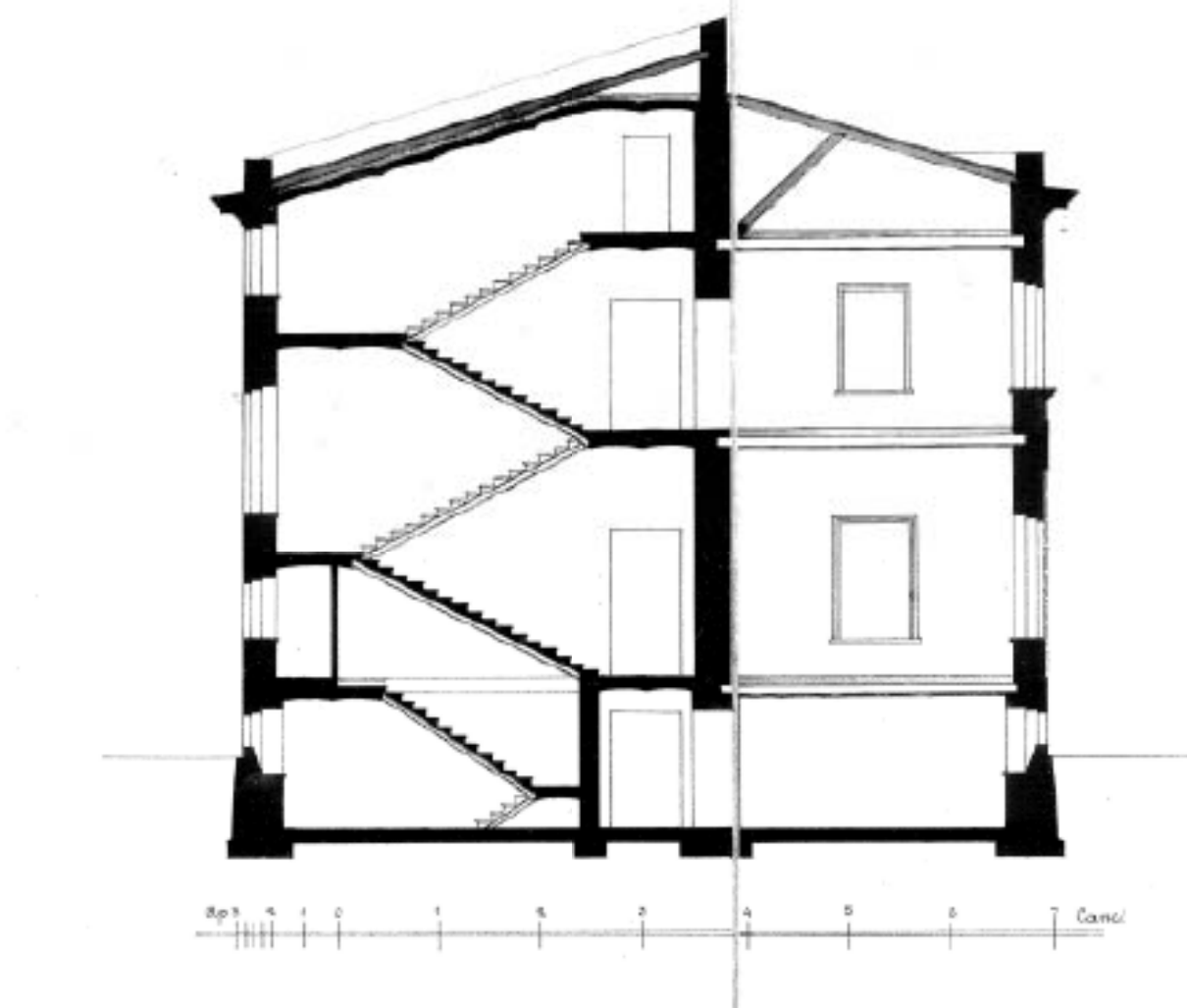
8. Разрез особняка В.П. Кочубя.
