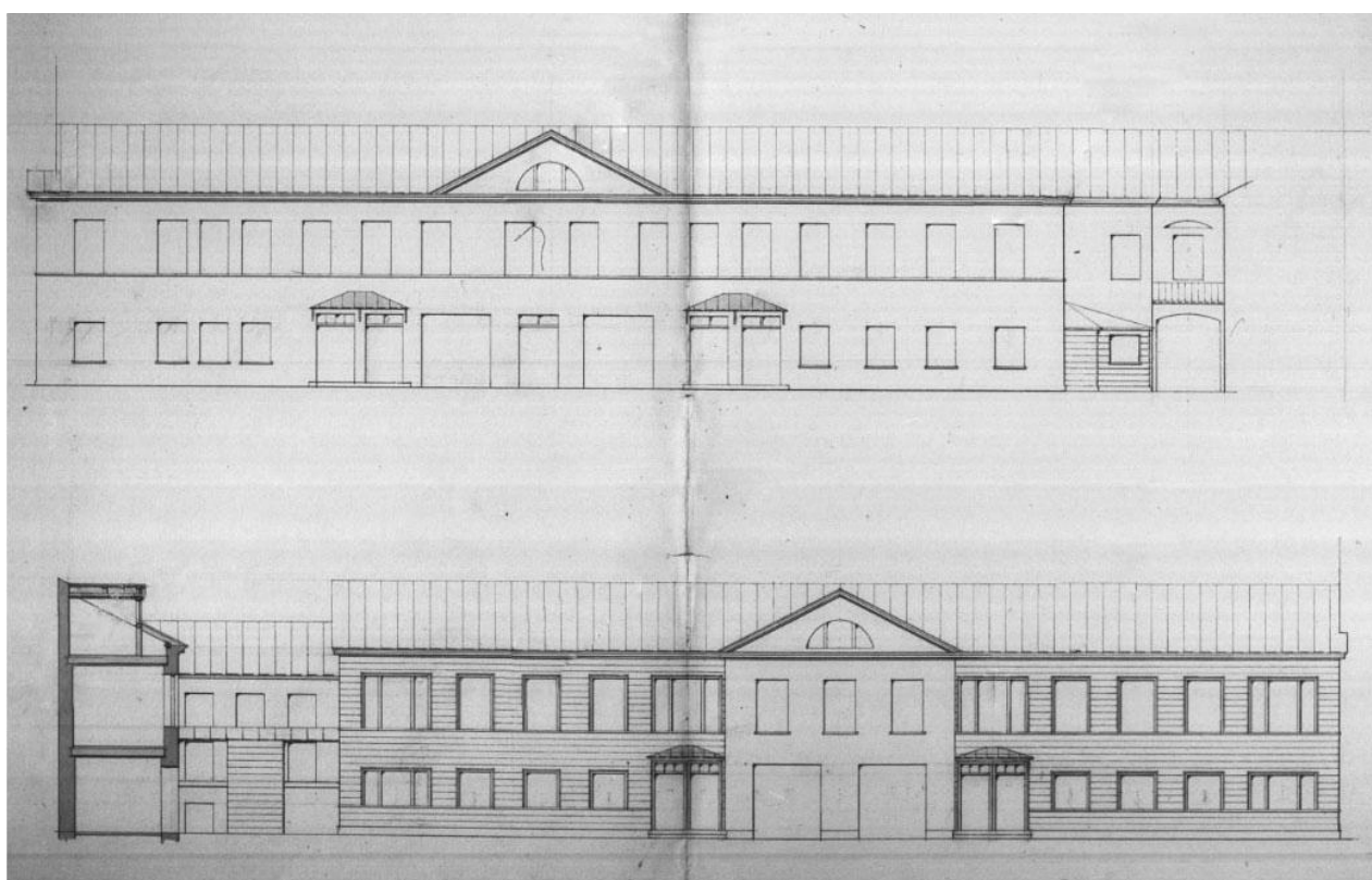
Илл. 9. Фасады. — ЦГИА СПб. Ф. 515. Оп. 4. Д. 2794
