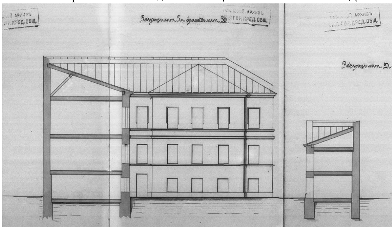
Илл. 20. Разрез лит. Г и фасад лит. В. — ЦГИА СПб. Ф. 515. Оп. 4. Д. 2794
