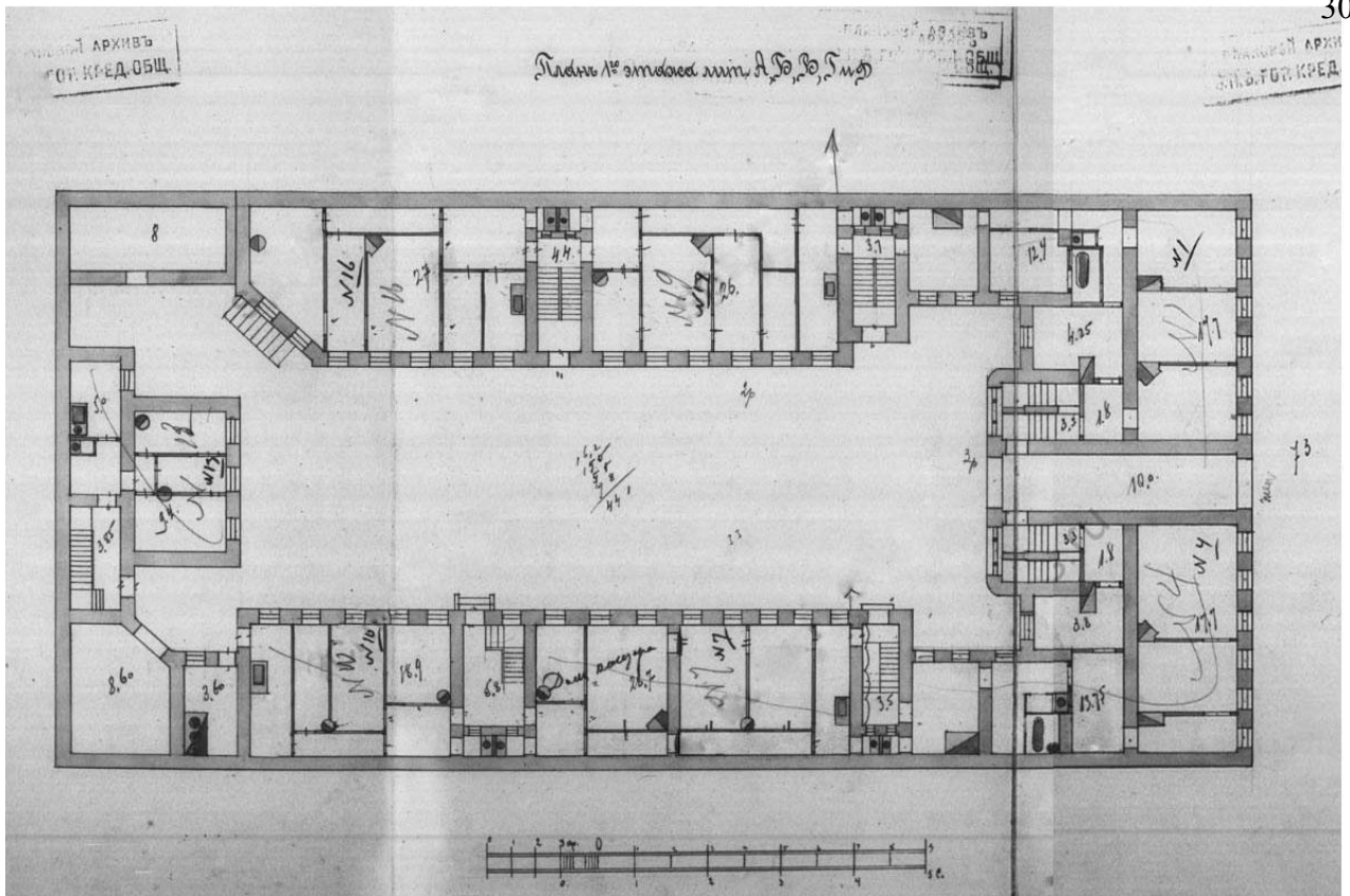
Илл. 13. План 1-го этажа лит. А, Б, В, Г и Д. — ЦГИА СПб. Ф. 515. Оп. 4. Д. 2794
