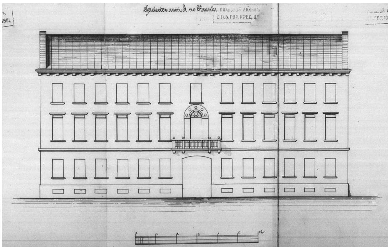
Илл. 11. Фасад лит. А по 8-ой линии. — ЦГИА СПб. Ф. 515. Оп. 4. Д. 2794
