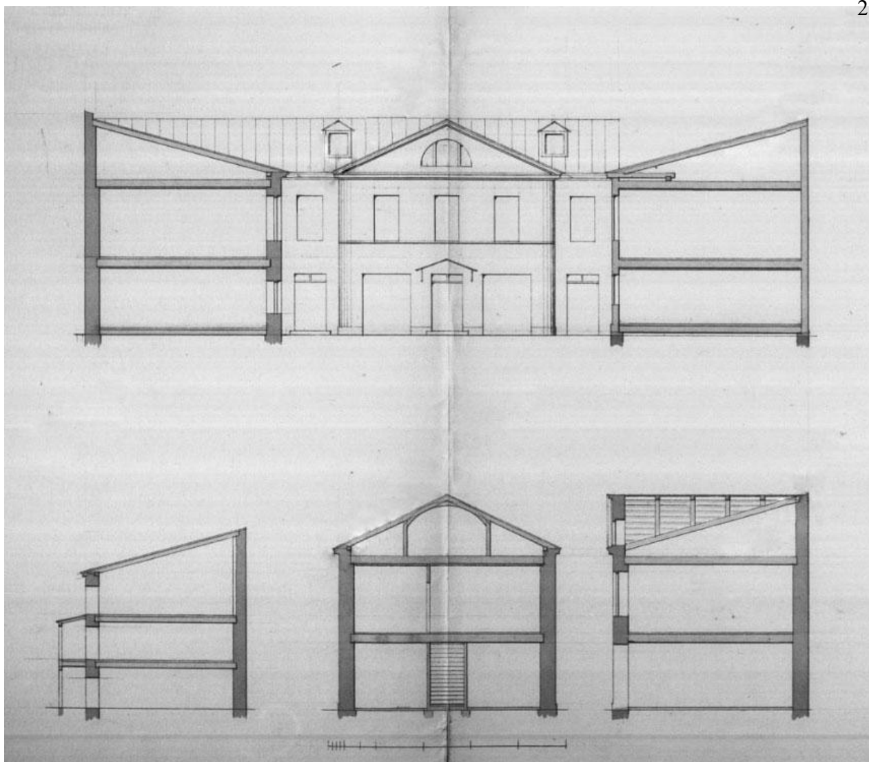
Илл. 8. Разрез. — ЦГИА СПб. Ф. 515. Оп. 4. Д. 2794
