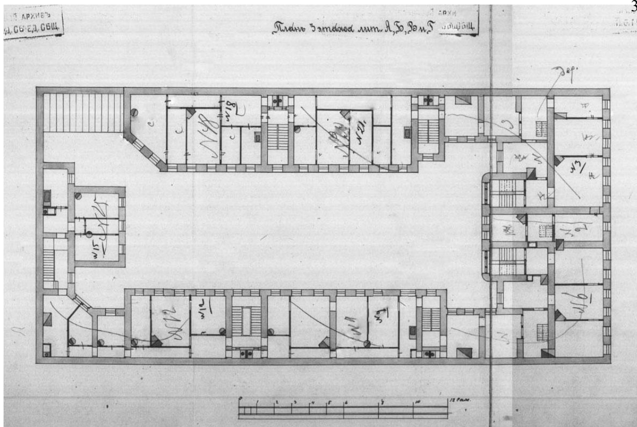
Илл. 15. План 3-го этажа лит. А, Б, В, Г и Д. — ЦГИА СПб. Ф. 515. Оп. 4. Д. 2794
