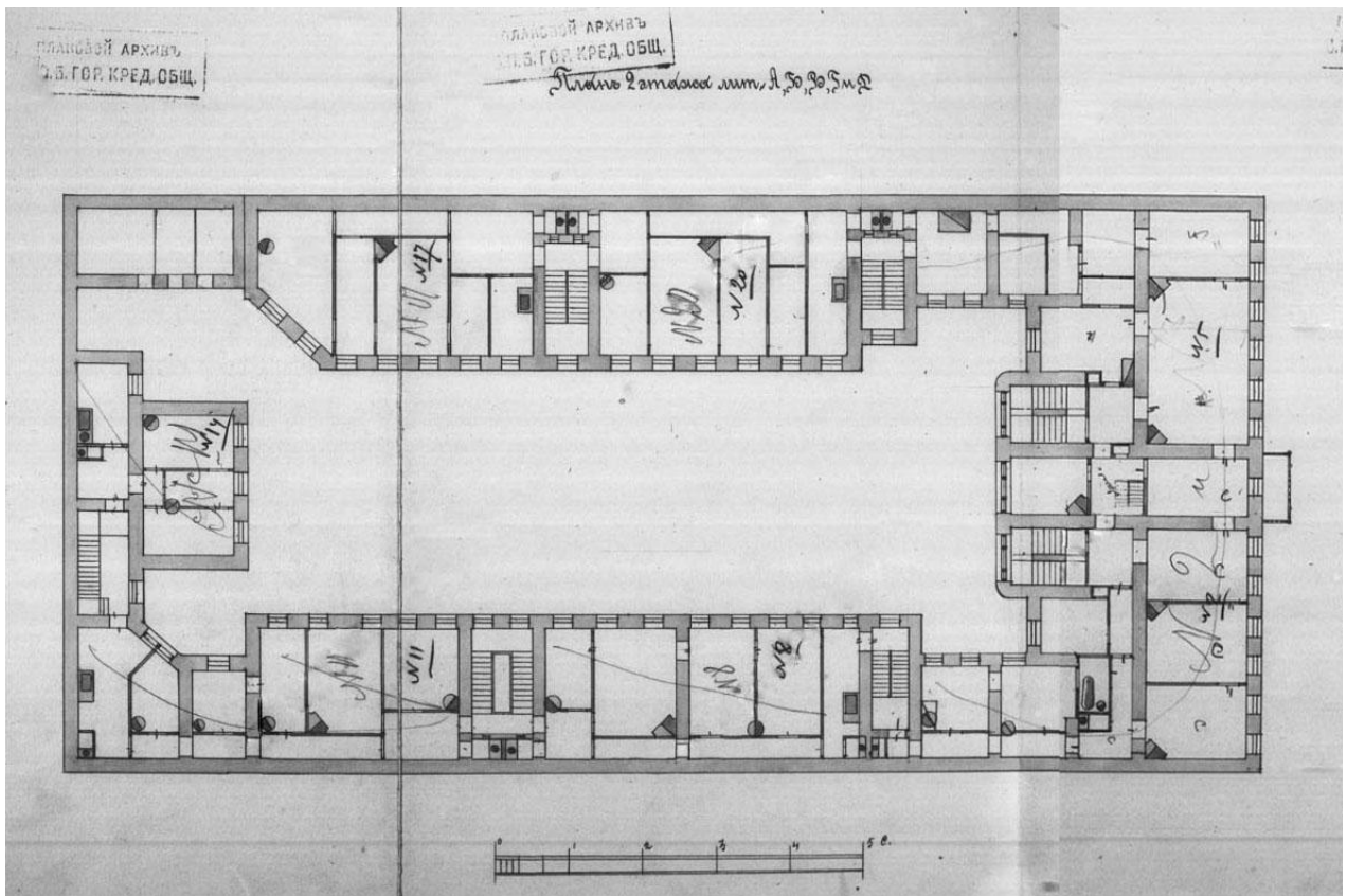
Илл. 14. План 2-го этажа лит. А, Б, В, Г и Д. — ЦГИА СПб. Ф. 515. Оп. 4. Д. 2794
