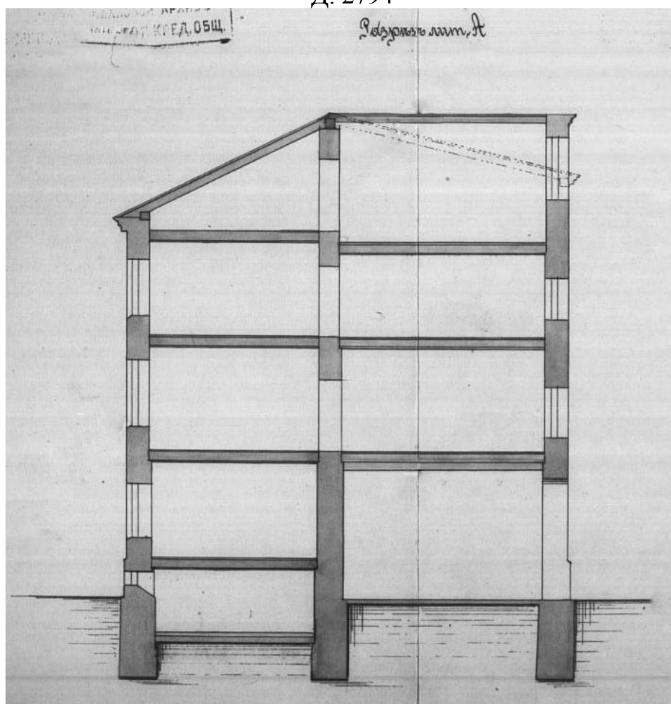
Илл. 18. Разрез лит. А. — ЦГИА СПб. Ф. 515. Оп. 4. Д. 2794
