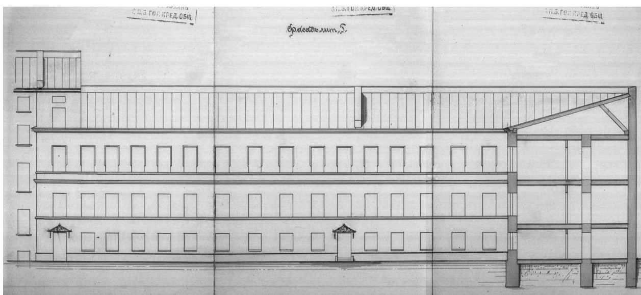
Илл. 21. Фасад лит. Г. — ЦГИА СПб. Ф. 515. Оп. 4. Д. 2794
