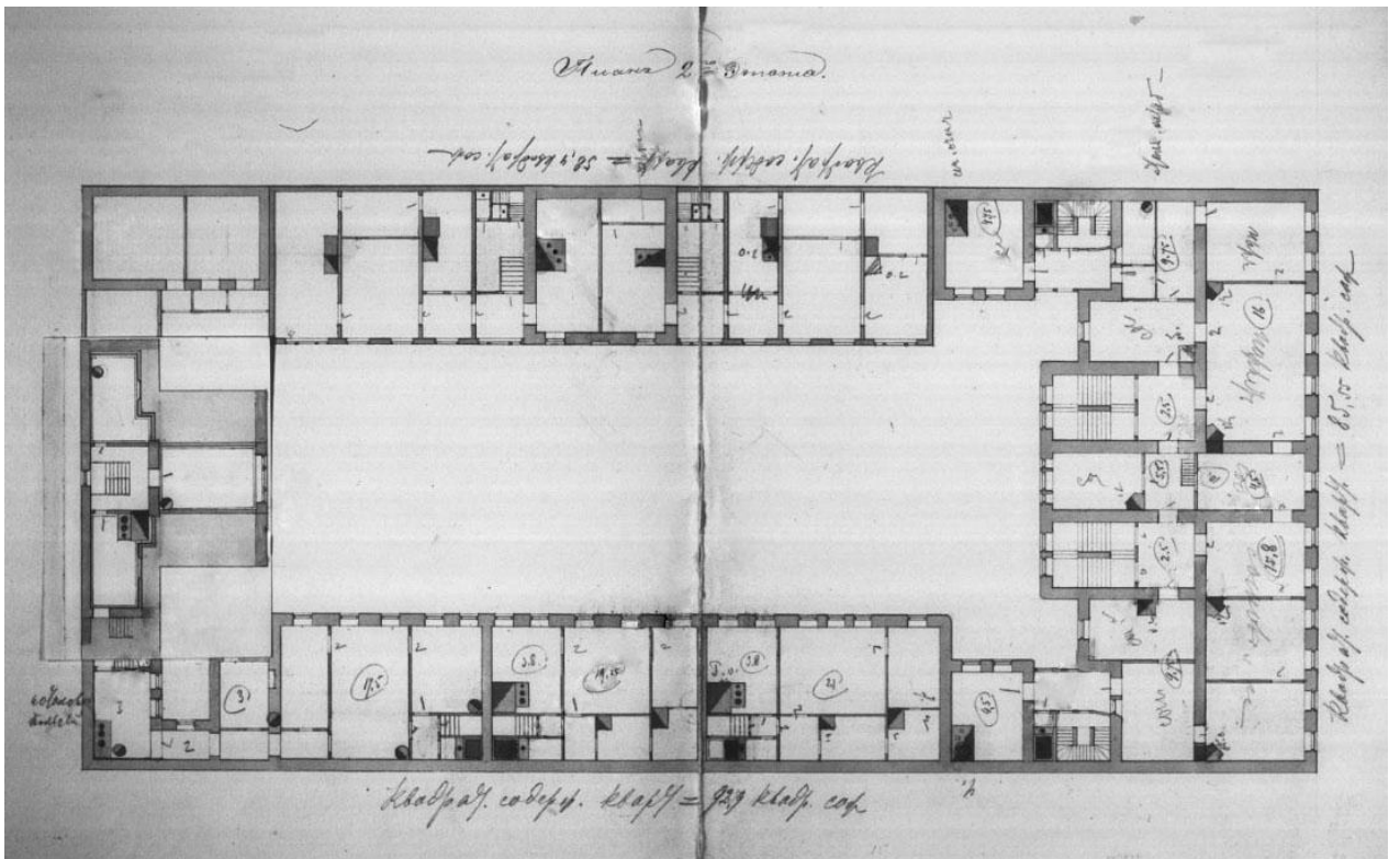
Илл. 5. План 2-го этажа. — ЦГИА СПб. Ф. 515. Оп. 4. Д. 2794
