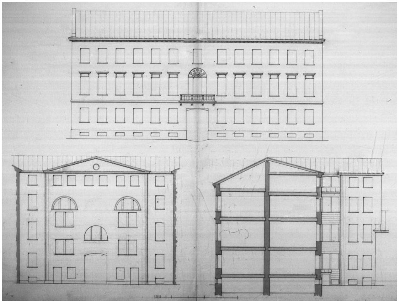
Илл. 7. Лицевой фасад. Дворовой фасад. Разрез. — ЦГИА СПб. Ф. 515. Оп. 4. Д. 2794
