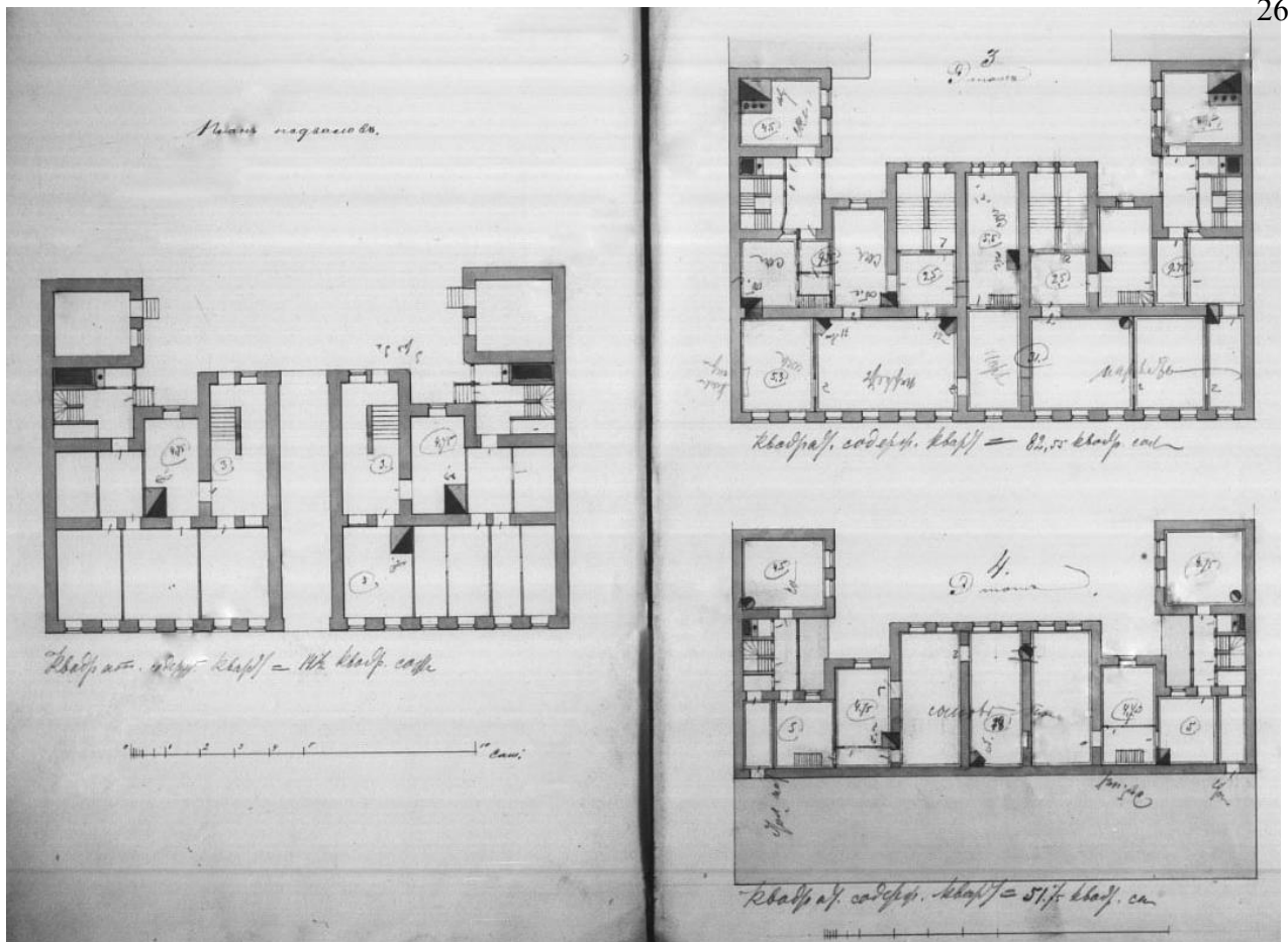
Илл. 6. План подвала. План 3-го этажа. План 4-го этажа. — ЦГИА СПб. Ф. 515. Оп. 4. Д. 2794
