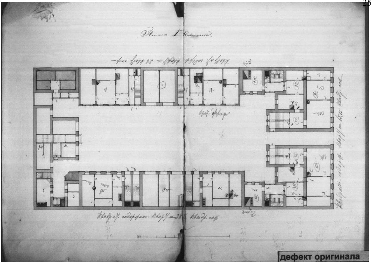
Илл. 4. План 1-го этажа. — ЦГИА СПб. Ф. 515. Оп. 4. Д. 2794
