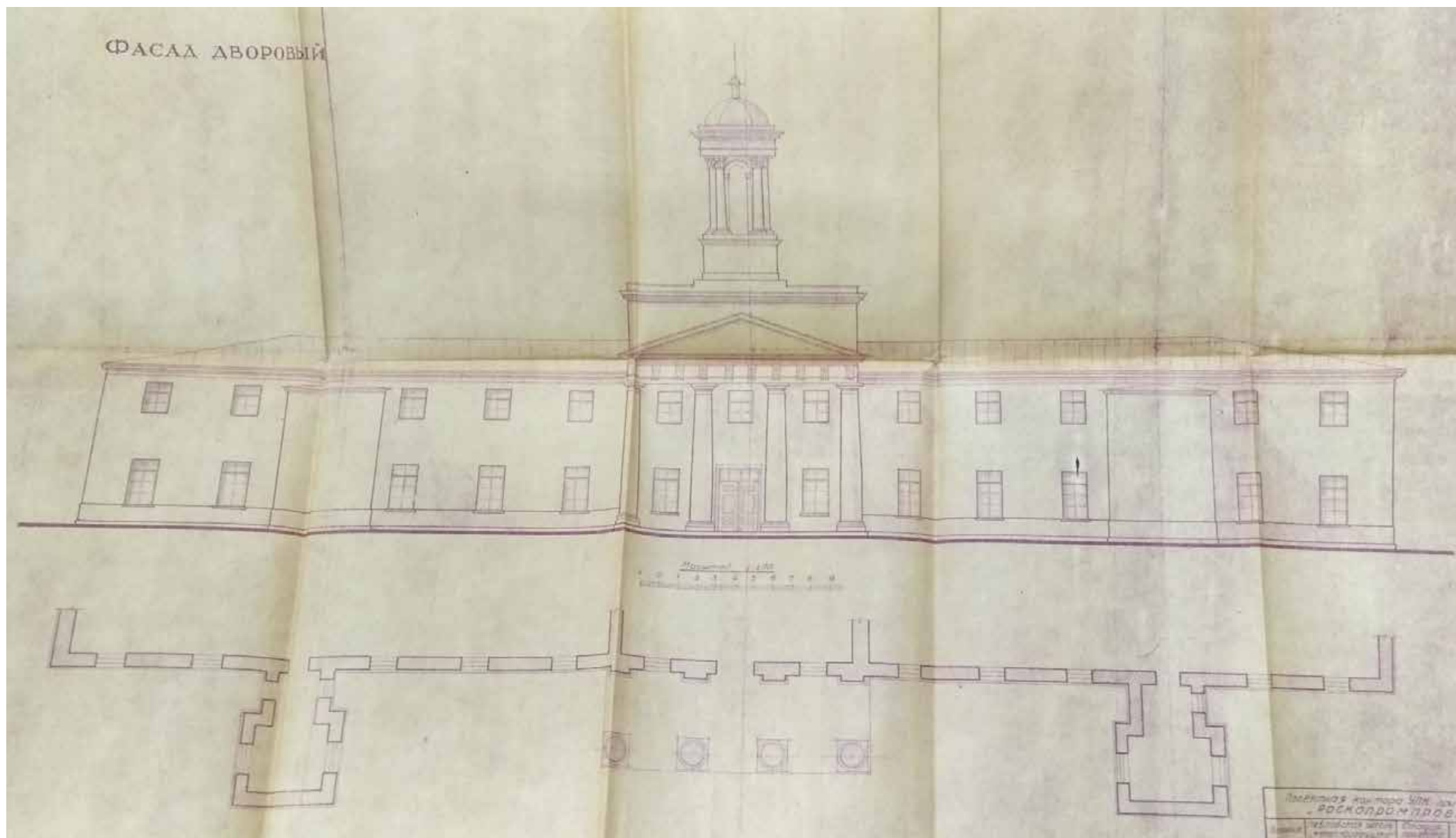
Ил. 28. Павловская ателье "Металлоигрушка". Главный производственный корпус. Дворовый /западный/ фасад. 1945 г. КГИОП. № 249. Пр-1. Проект восстановления з-да Артели "Точмех" в г. Павловске. Ленинградской обл. Часть Архитектурная. / Роскопромпроект. 1946 г.
