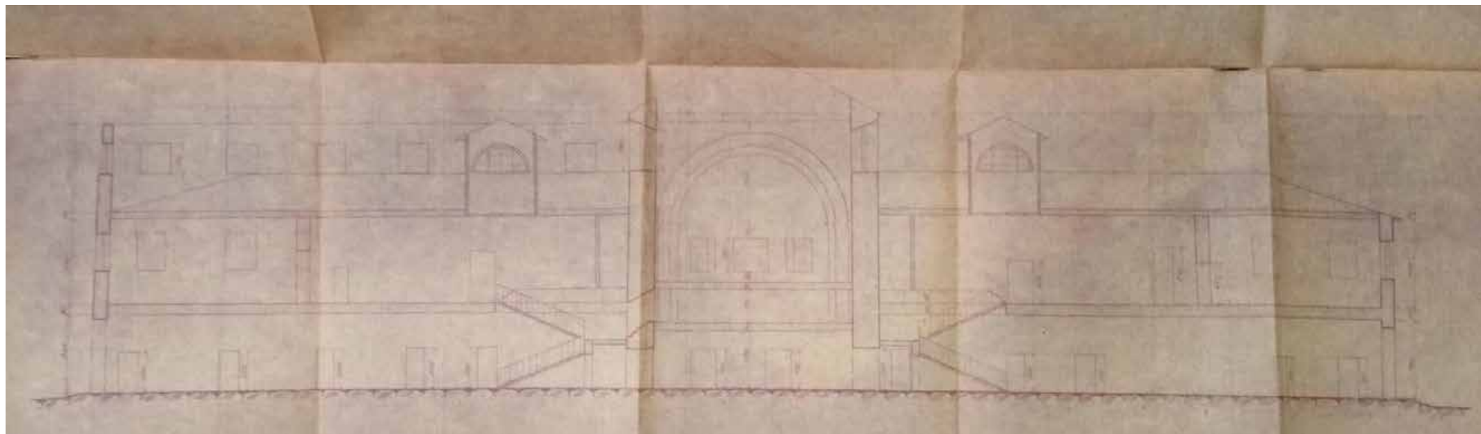
Ил. 35. Павловская ателье "Металлоигрушка". Главный корпус. Продольный разрез. Обмерные чертежи. 1945 г. КГИОП. № 249. Пр-1. Проект восстано- вления 3-да Артели "Точмех" в г. Павловске. Ленинградской обл. Часть 1. Строительно- обмерочные чертежи. / Роскопромпроект. 1946 г.
