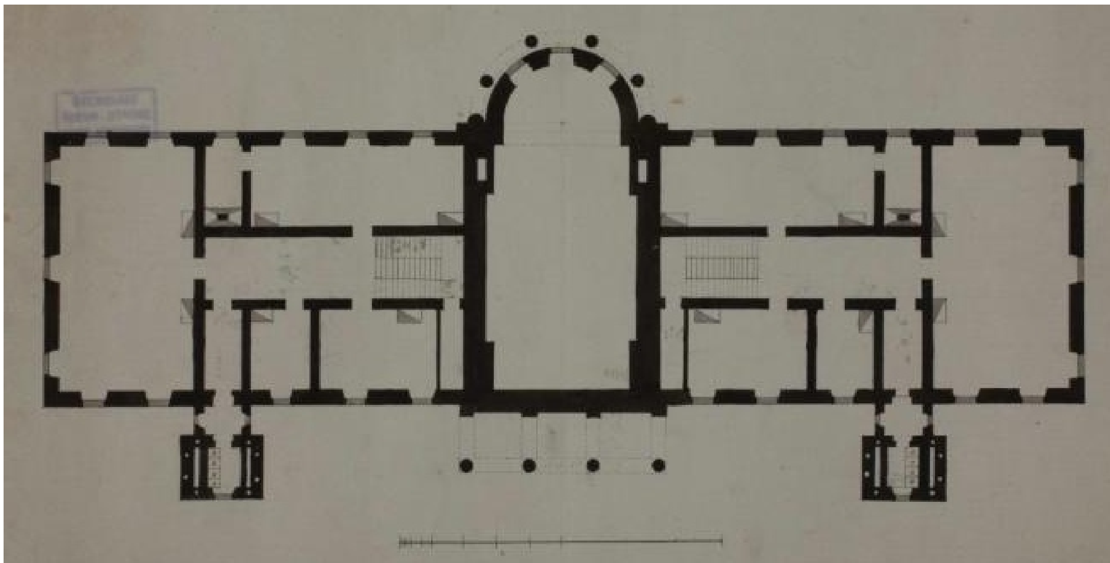
Ил. 14. Кваренги Джакомо (?). Павловск. Мариинский госпиталь. Проект перестройки. План 2-го этажа. Первая половина XIX века /1809 г.?! Хранится: ФГБУК "Государственный музей-заповедник "Павловск", № Ч-441.
