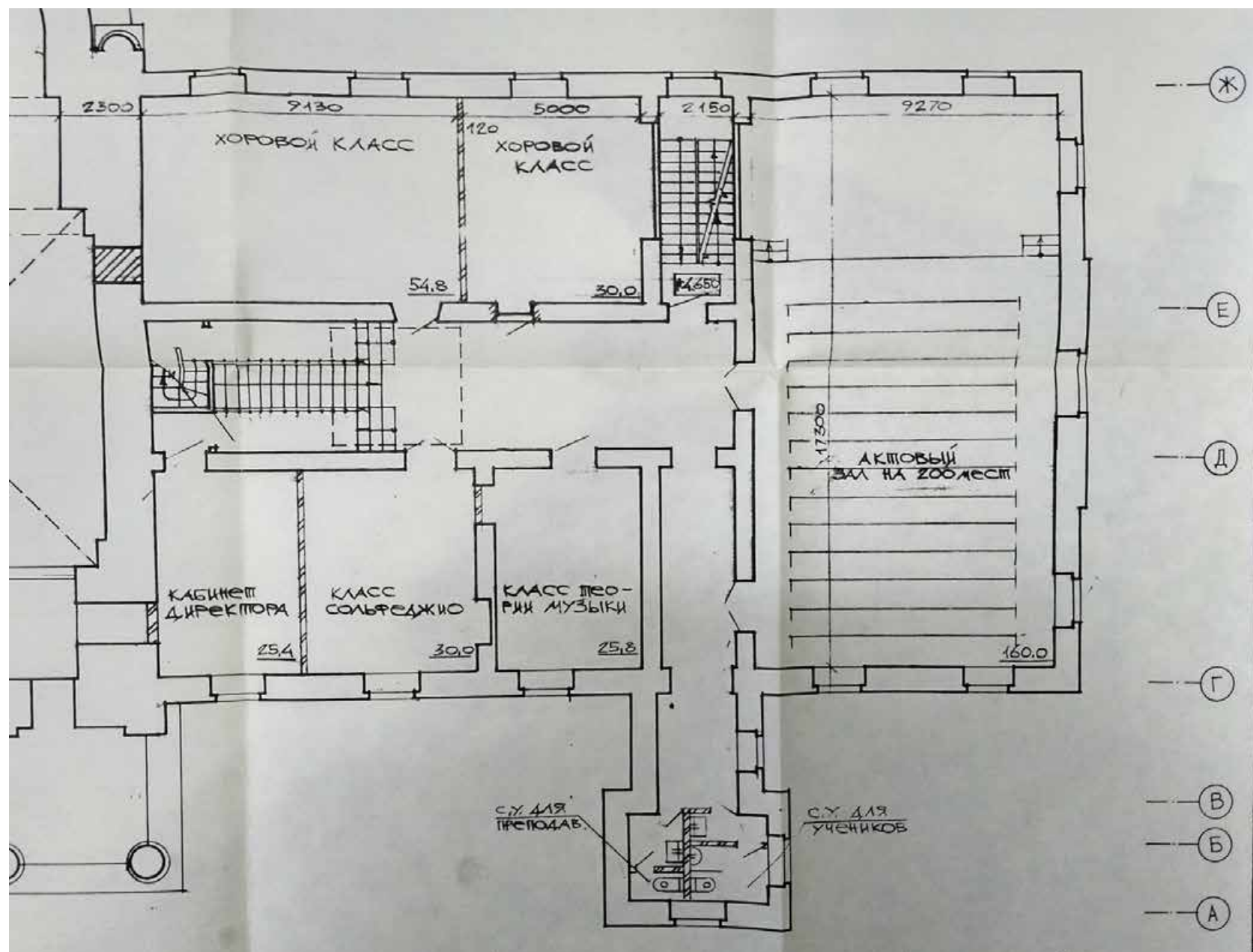
Ил. 68. Госпиталь с церковью Св. Марии Магдалины в г. Павловске. Эскиз. План приспособления помещений 2-го этажа южного корпуса. 1997 г. КГИОП. № 249. Пр-6. г. Павловск. Госпиталь с ц. Св. Марии Магдалины. Проект реставрации и приспособления. Проектные работы. Эскизный проект реставрации и приспособления. СФР. Т.3. Кн.1. / ИЧП АРМ Павловой И.Е. "ИРИНА". СПб., 1997.
