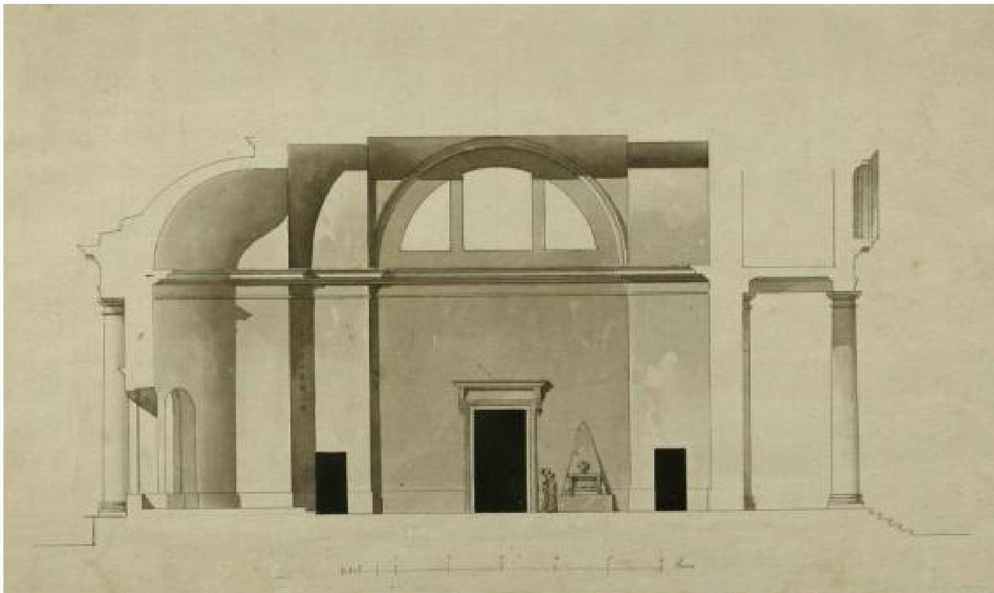
Ил. 7. Кваренги Джакомо. Павловск. Мариинский госпиталь. Ц-вь св. Марии Магдалины. Продольный разрез. Около 1784 г. Хранится: ФГБУК "Государственный музей-заповедник "Павловск", № Ч-446.
