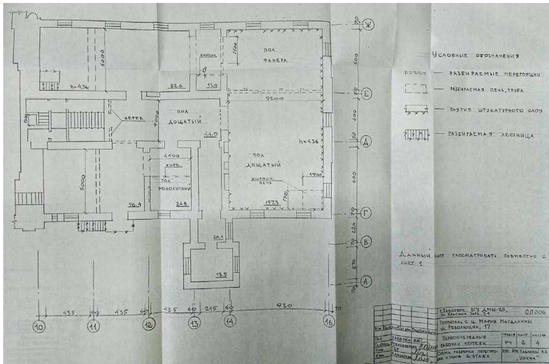
Ил. 48. Госпиталь с ц. Св. Марии Магдалины. ул. Революции, 17. Схема разборки перегородок и полов 2-го этажа южного корпуса. 1996 г. КГИОП. № 249. Пр-4. г. Павловск. Госпиталь с ц. Св. Марии Магдалины. Проект реставрации и приспособления под детскую музыкальную школу №25. Предварительные работы. Первоочередные рабочие чертежи. Т.1. Кн.2. / ИЧП АРМ Павловой И.Е. "ИРИНА". СПб., 1996.
