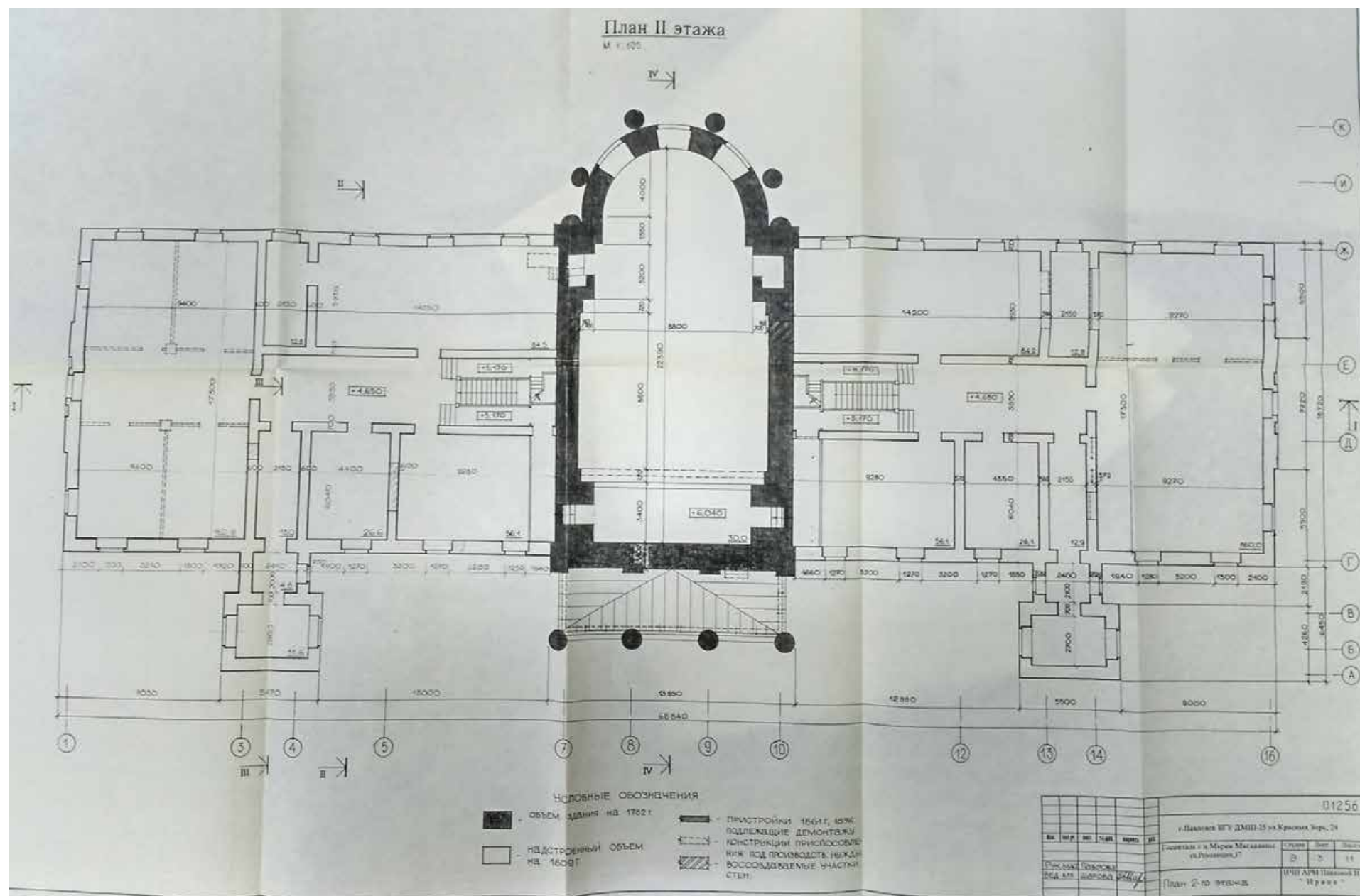
Ил. 53. Госпиталь с церковью Св. Марии Магдалины в г. Павловске. Эскизный проект. План 2-го этажа. 1997 г. КГИОП. № 249. Пр-6. г. Павловск. Госпиталь с ц. Св. Марии Магдалины. Проект реставрации и приспособления. Проектные работы. Эскизный проект реставрации и приспособления. СФР. Т.3. Кн.1. / ИЧП АРМ Павловой И.Е. "ИРИНА". СПб., 1997.
