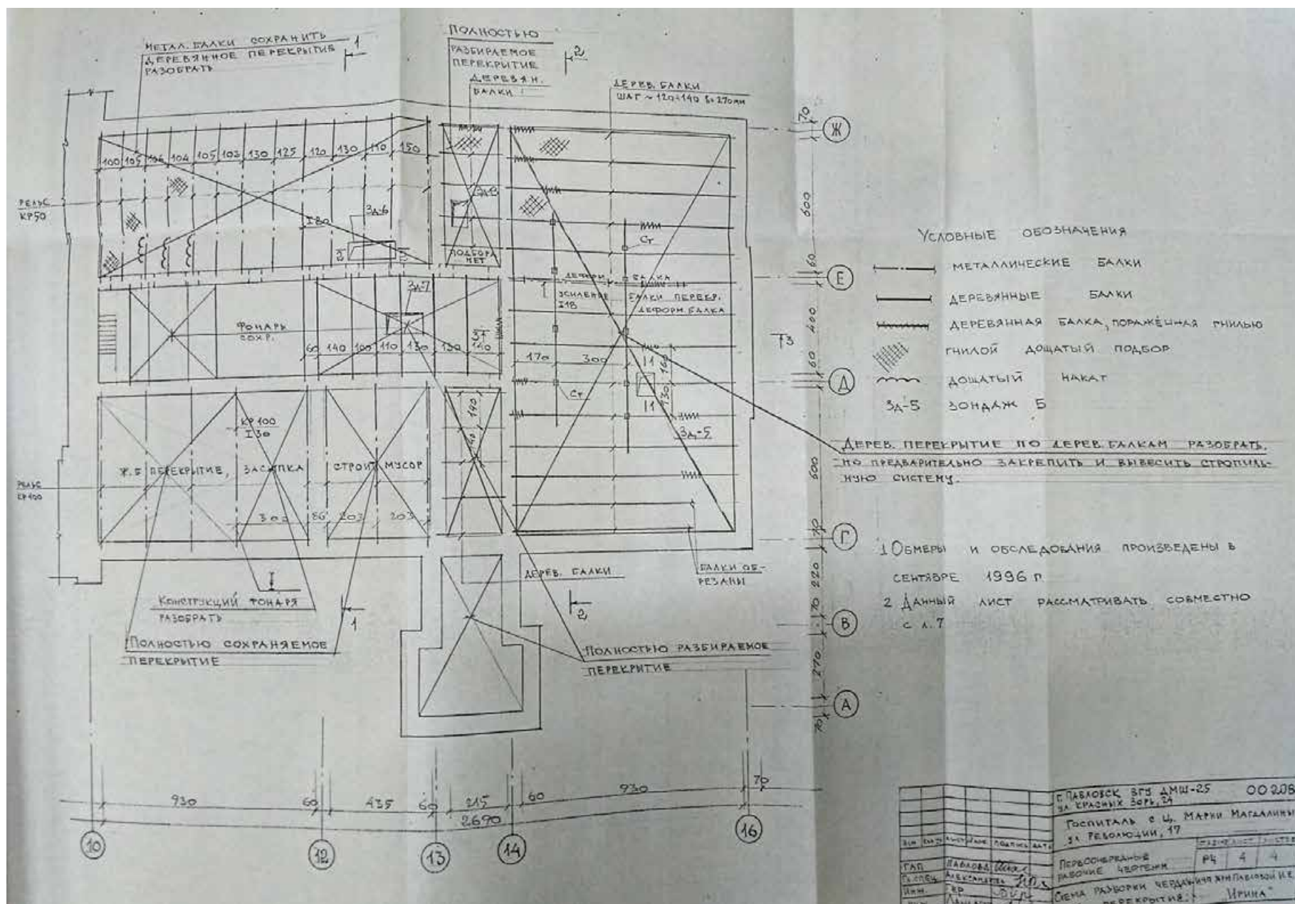
Ил. 50. Госпиталь с ц. Св. Марии Магдалины. ул. Революции, 17. Схема разборки чердачного перекрытия южного корпуса. 1996 г. КГИОП. № 249. Пр-4. г. Павловск. Госпиталь с ц. Св. Марии Магдалины. Проект реставрации и приспособления под детскую музыкальную школу №25. Предварительные работы. Первоочередные рабочие чертежи. Т.1. Кн.2. / ИЧП АРМ Павловой И.Е. "ИРИНА". СПб., 1996.
