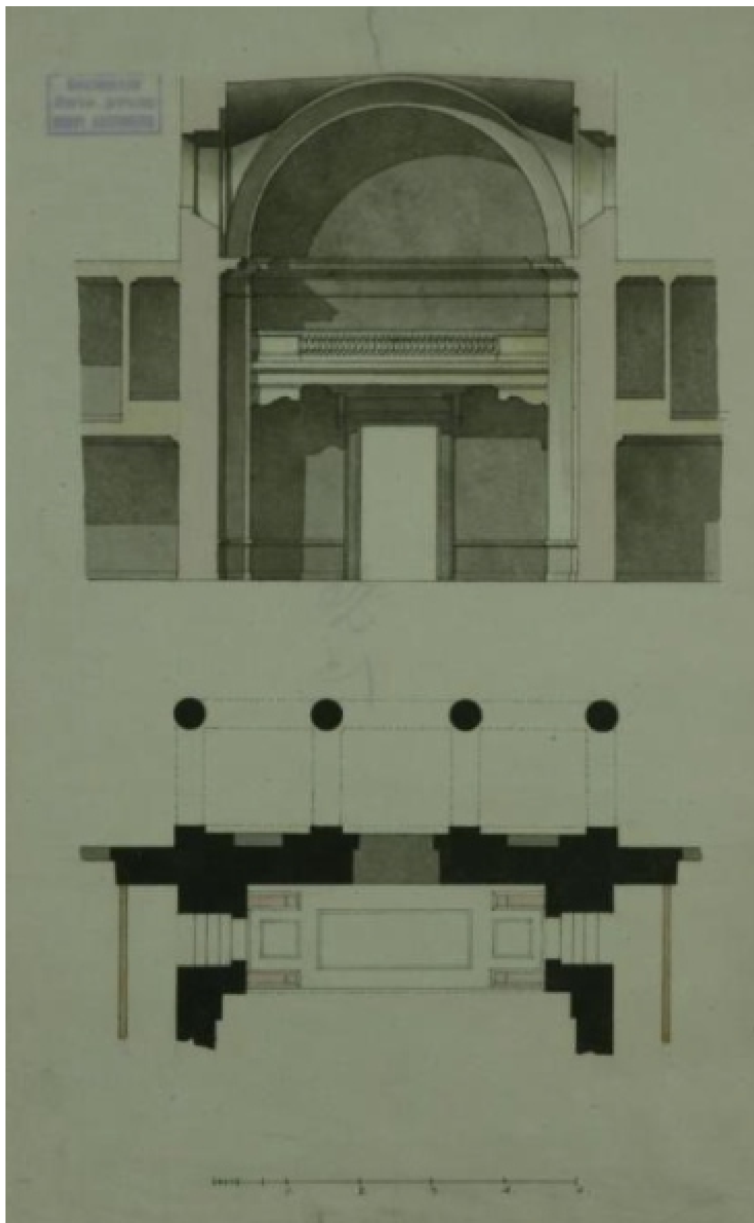
Ил. 6. Кваренги Джакомо. Павловск. Мариинский госпиталь. Церковь святой Марии Магдалины. Проект устройства хоров. Вариант с балюстрадой. 1780-е гг. Хранится: ФГБУК "Государственный музей-заповедник "Павловск". № Ч-448.
