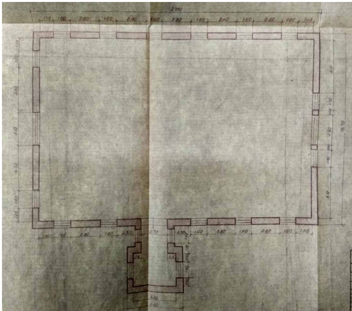
Ил. 34. Павловская ателье "Металлоигрушка". Главный корпус. План 3-го этажа. Над северным корпусом. Обмерные чертежи. 1945 г. КГИОП. № 249. Пр-1. Проект восстановления з-да Артели "Точмех" в г. Павловске. Ленинградской обл. Часть 1. Строительно-обмерочные чертежи. / Роскопромпроект. 1946 г.
