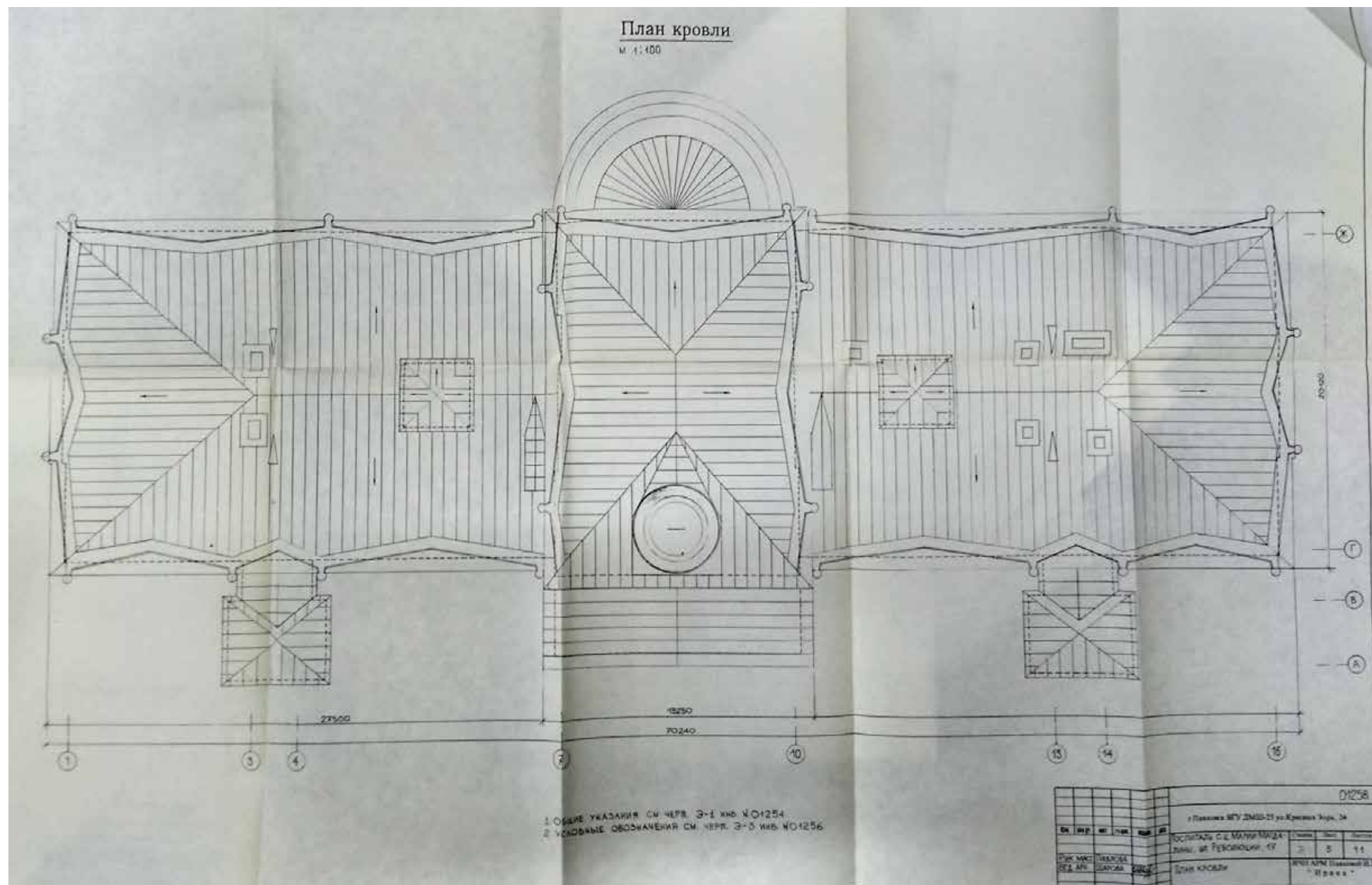
Ил. 56. Госпиталь с церковью Св. Марии Магдалины в г. Павловске. Эскизный проект. План кровли. 1997 г. КГИОП. № 249. Пр-6. г. Павловск. Госпиталь с ц. Св. Марии Магдалины. Проект реставрации и приспособления. Проектные работы. Эскизный проект реставрации и приспособления. СФР. Т.3. Кн.1. / ИЧП АРМ Павловой И.Е. "ИРИНА". СПб., 1997.
