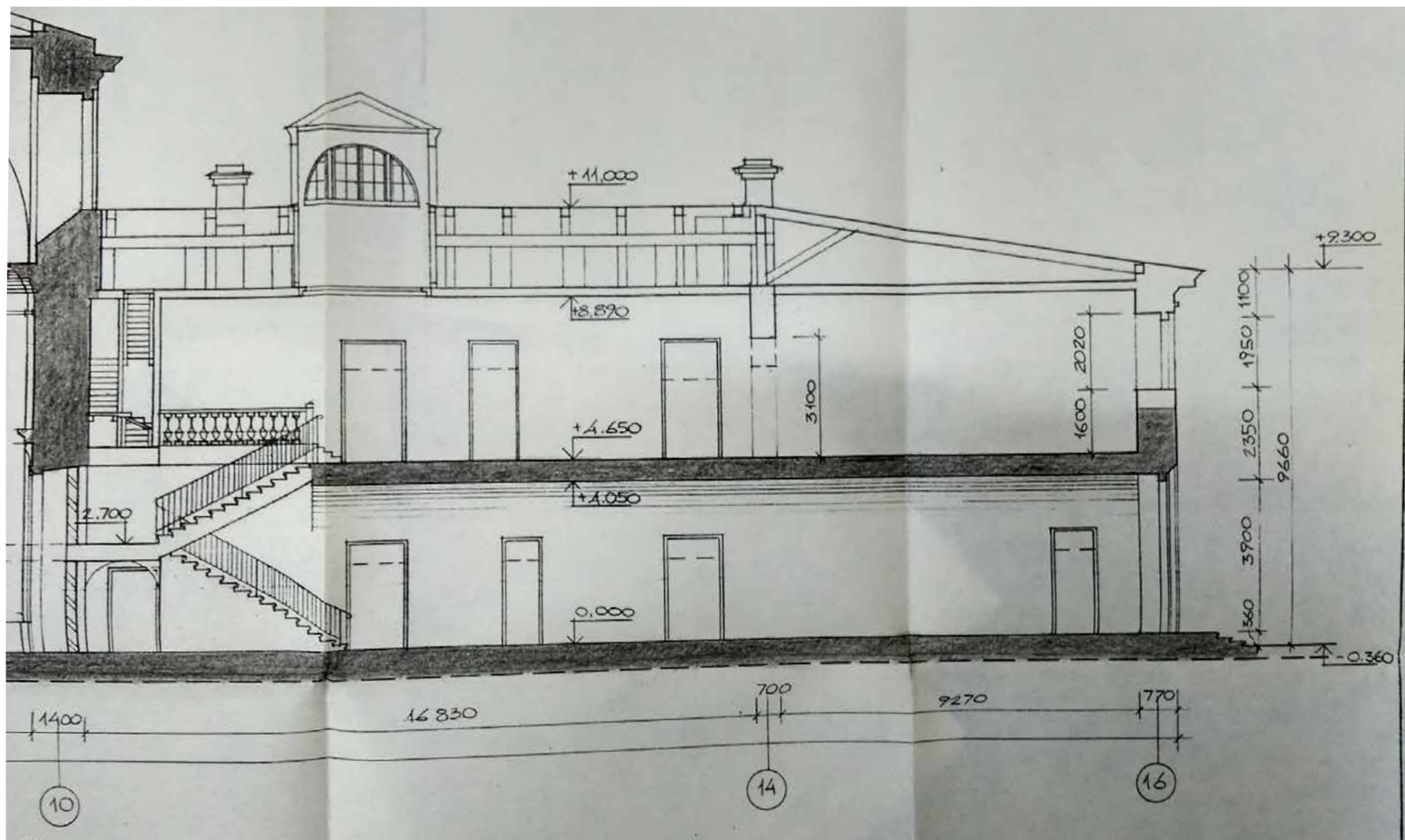
Ил. 58. Госпиталь с церковью Св. Марии Магдалины в г. Павловске. Эскизный проект. Разрезы 1-1. Фрагмент с южным корпусом. 1997 г. КГИОП. № 249. Пр-6. г. Павловск. Госпиталь с ц. Св. Марии Магдалины. Проект реставрации и приспособления. Проектные работы. Эскизный проект реставрации и приспособления. СФР. Т.З. Кн.1. / ИЧП АРМ Павловой И.Е. "ИРИНА". СПб., 1997.
