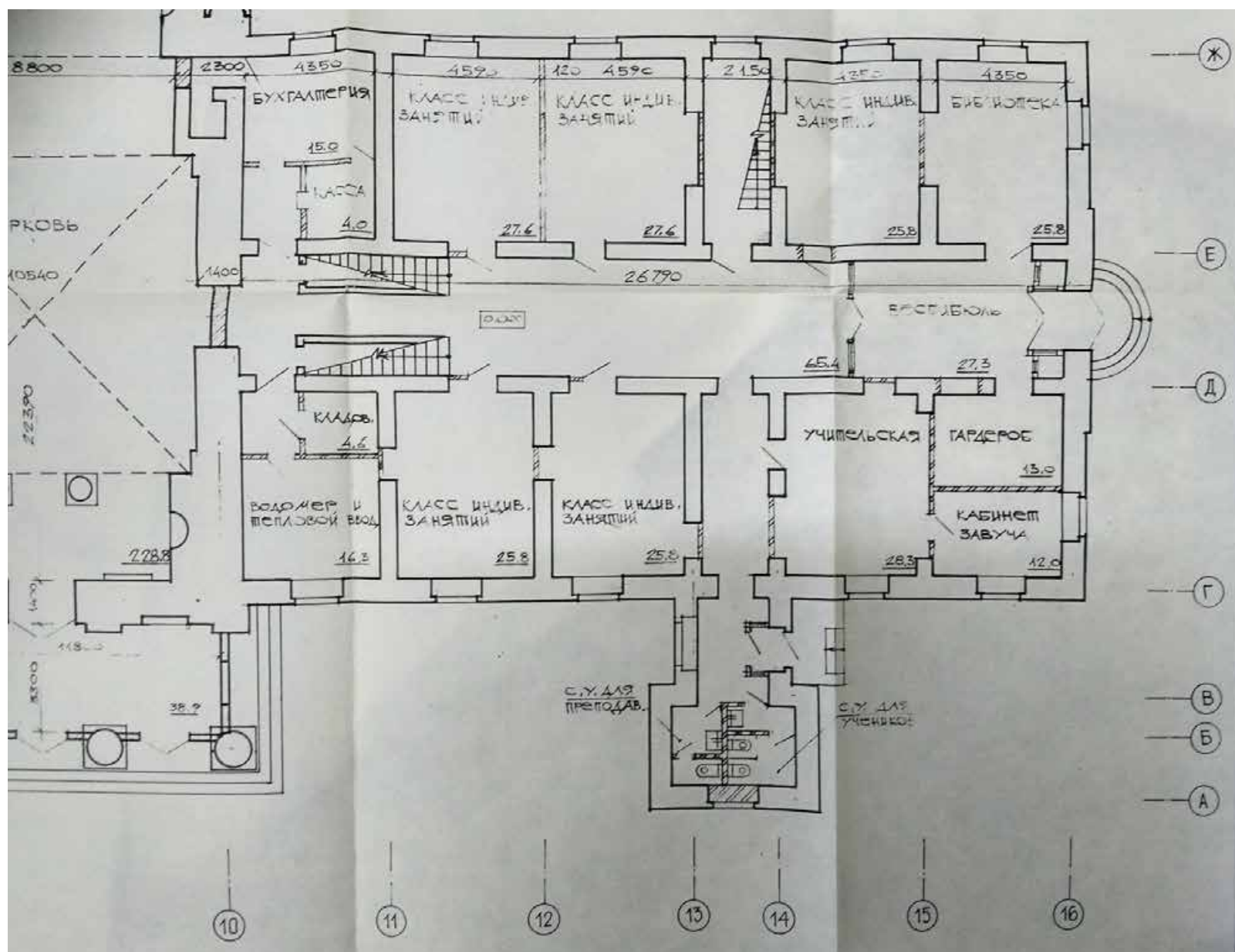
Ил. 66. Госпиталь с церковью Св. Марии Магдалины в г. Павловске. Эскиз. План приспособления помещений 1-го этажа южного корпуса. 1997 г. КГИОП. № 249. Пр-6. г. Павловск. Госпиталь с ц. Св. Марии Магдалины. Проект реставрации и приспособления. Проектные работы. Эскизный проект реставрации и приспособления. СФР. Т.3. Кн.1. / ИЧП АРМ Павловой И.Е. "ИРИНА". СПб., 1997.
