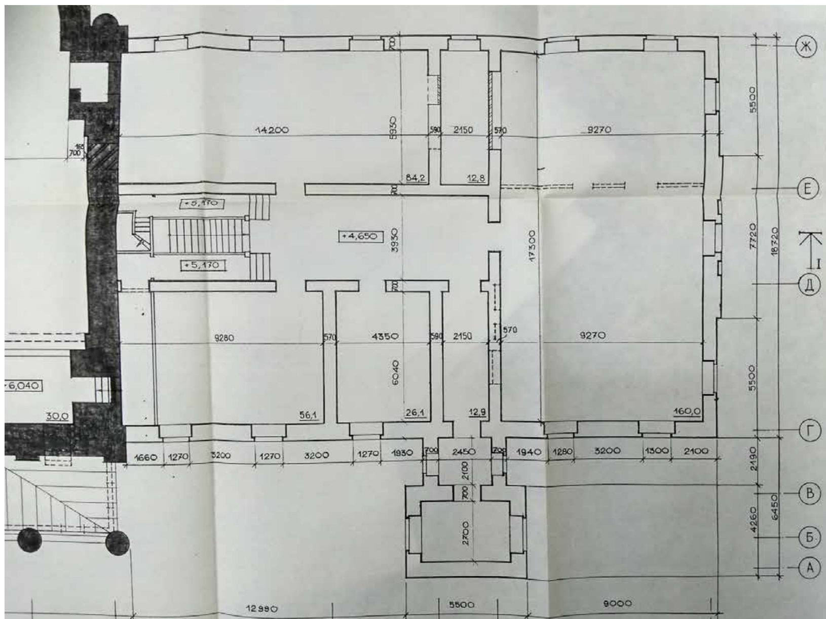
Ил. 54. Госпиталь с церковью Св. Марии Магдалины в г. Павловске. Эскизный проект. План 2-го этажа южного корпуса. 1997 г. КГИОП. № 249. Пр-6. г. Павловск. Госпиталь с ц. Св. Марии Магдалины. Проект реставрации и приспособления. Проектные работы. Эскизный проект реставрации и приспособления. СФР. Т.3. Кн.1. / ИЧП АРМ Павловой И.Е. "ИРИНА". СПб., 1997.
