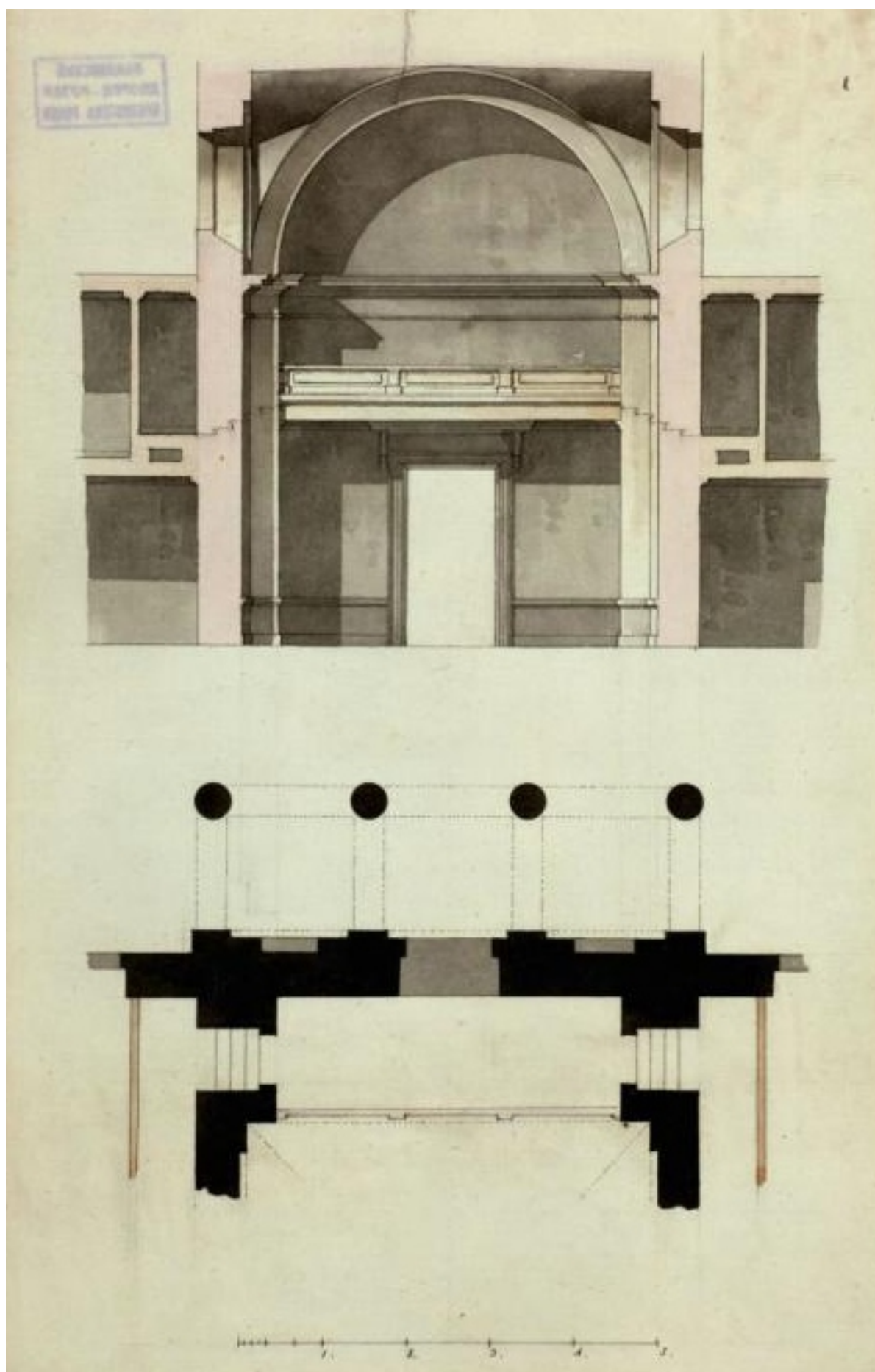
Ил. 5. Кваренги Джакомо. Павловск. Мариинский госпиталь. Церковь святой Марии Магдалины. Проект устройства хоров. 1780-е гг. Хранится: ФГБУК "Государственный музей-заповедник "Павловск". № Ч-447.
