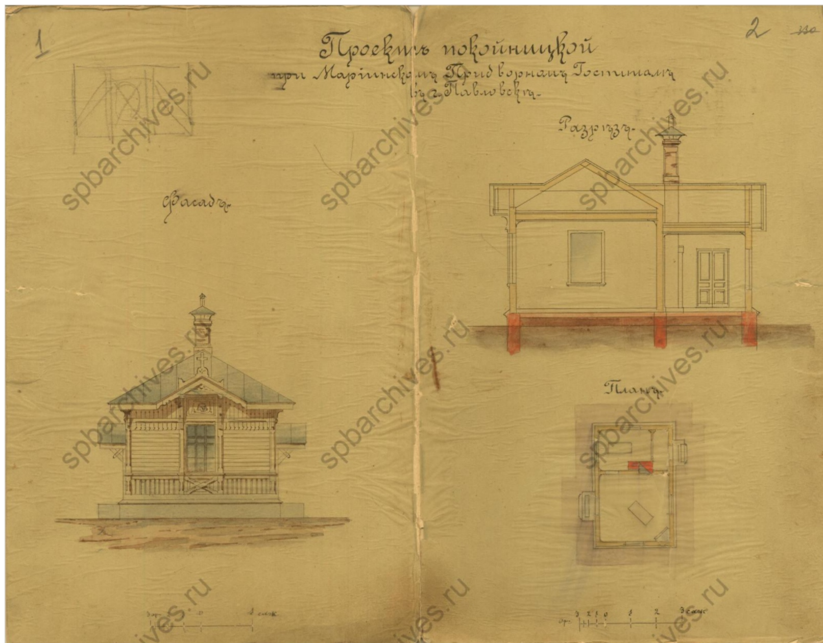
Ил. 18. Проект покойницкой при Мариинском госпитале в Павловске. Конец XIX - начало XX в. ЦГИА СПб. Ф.2257. Оп.1. Д.99. Л.1-2.
