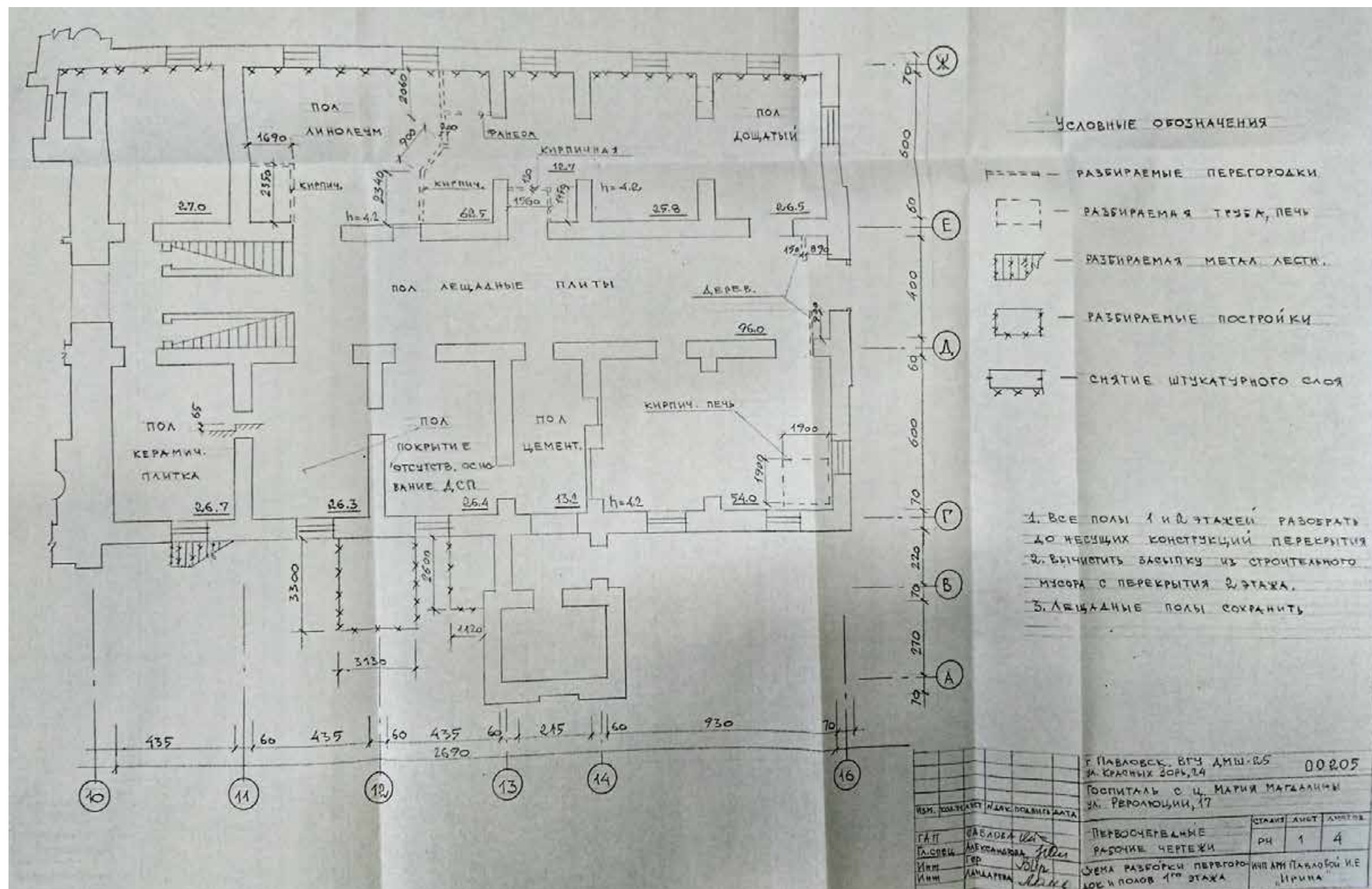
Ил. 47. Госпиталь с ц. Св. Марии Магдалины. ул. Революции, 17. Схема разборки перегородок и полов 1-го этажа южного корпуса. 1996 г. КГИОП. № 249. Пр-4. г. Павловск. Госпиталь с ц. Св. Марии Магдалины. Проект реставрации и приспособления под детскую музыкальную школу №25. Предварительные работы. Первоочередные рабочие чертежи. Т.1. Кн.2. / ИЧП АРМ Павловой И.Е. "ИРИНА". СПб., 1996.
