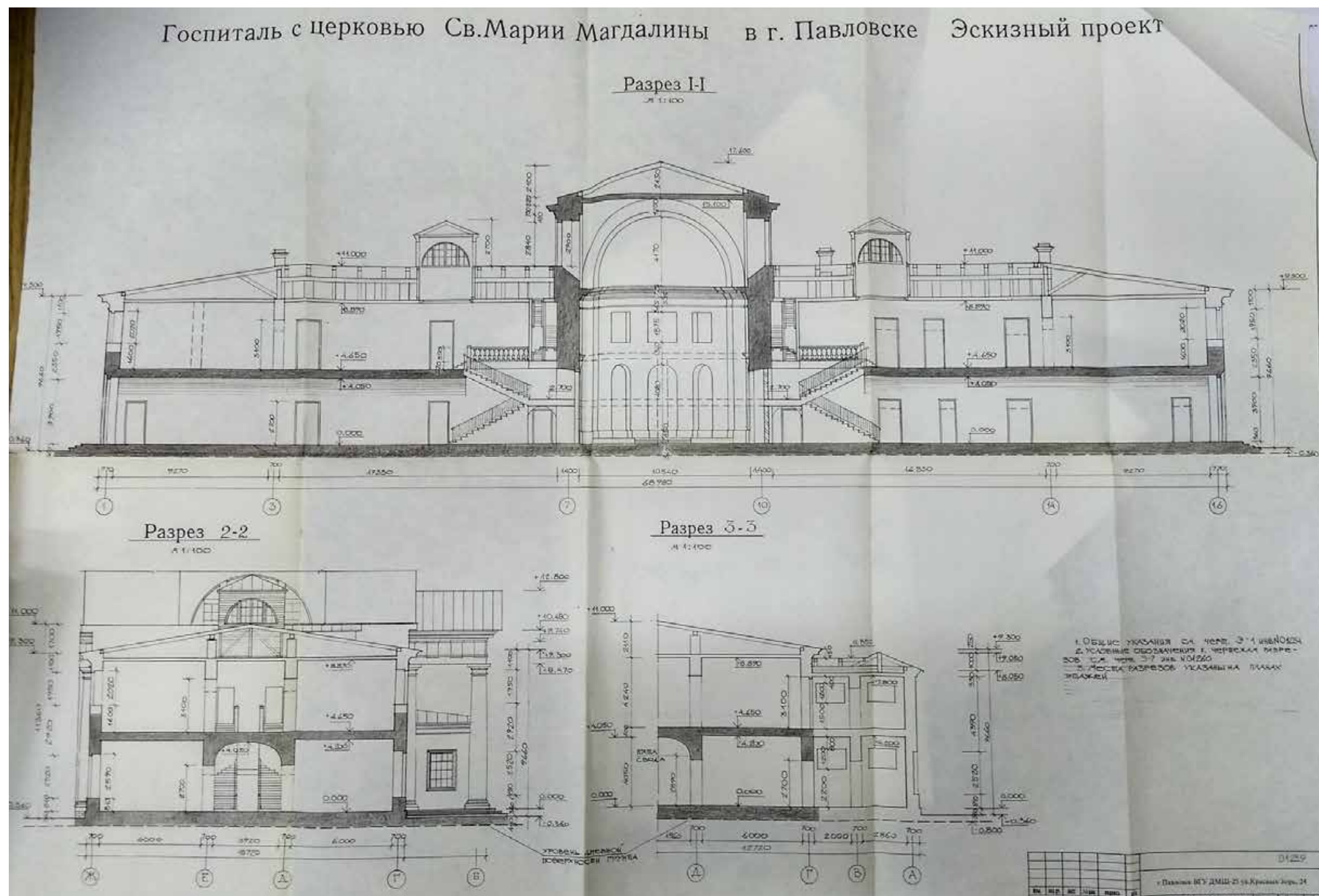
Ил. 57. Госпиталь с церковью Св. Марии Магдалины в г. Павловске. Эскизный проект. Разрезы 1-1, 2-2, 3-3. 1997 г. КГИОП. № 249. Пр-6. г. Павловск. Госпиталь с ц. Св. Марии Магдалины. Проект реставрации и приспособления. Проектные работы. Эскизный проект реставрации и приспособления. СФР. Т.3. Кн.1. / ИЧП АРМ Павловой И.Е. "ИРИНА". СПб., 1997.
