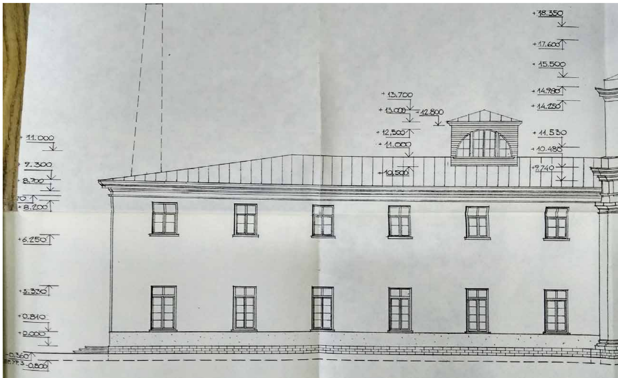
Ил. 64. Госпиталь с церковью Св. Марии Магдалины в г. Павловске. Эскизный проект. Восточный фасад южного корпуса. 1997 г. КГИОП. № 249. Пр-6. г. Павловск. Госпиталь с ц. Св. Марии Магдалины. Проект реставрации и приспособления. Проектные работы. Эскизный проект реставрации и приспособления. СФР. Т.3. Кн.1. / ИЧП АРМ Павловой И.Е. "ИРИНА". СПб., 1997.
