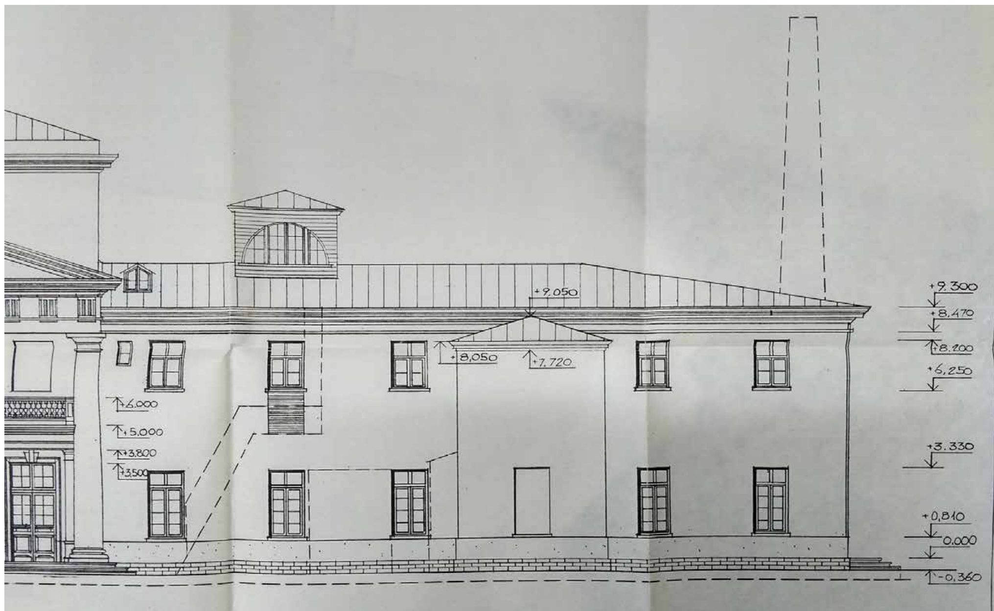
Ил. 62. Госпиталь с церковью Св. Марии Магдалины в г. Павловске. Эскизный проект. Западный фасад южного корпуса. 1997 г. КГИОП. № 249. Пр-6. г. Павловск. Госпиталь с ц. Св. Марии Магдалины. Проект реставрации и приспособления. Проектные работы. Эскизный проект реставрации и приспособления. СФР. Т.3. Кн.1. / ИЧП АРМ Павловой И.Е. "ИРИНА". СПб., 1997.
