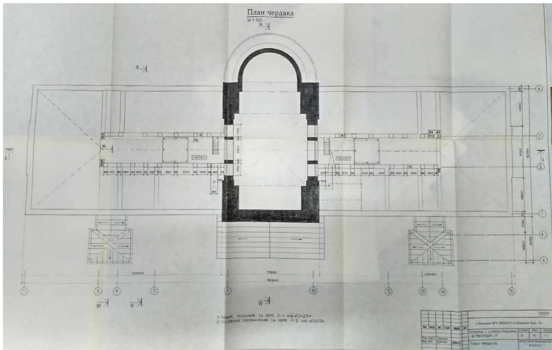
Ил. 55. Госпиталь с церковью Св. Марии Магдалины в г. Павловске. Эскизный проект. План чердака. 1997 г. КГИОП. № 249. Пр-6. г. Павловск. Госпиталь с ц. Св. Марии Магдалины. Проект реставрации и приспособления. Проектные работы. Эскизный проект реставрации и приспособления. СФР. Т.3. Кн.1. / ИЧП АРМ Павловой И.Е. "ИРИНА". СПб., 1997.
