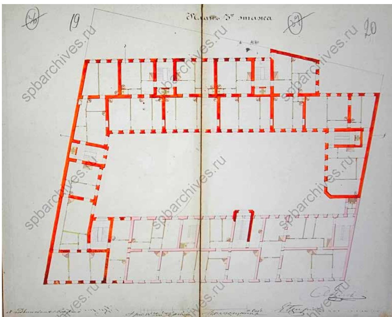
7. План 3-го этажа предполагаемого к постройке нового дома. 1858 г. Арх. Пель. ЦГИА СПб. Ф.513. Оп.102. Д.4684. Л.19-20.
