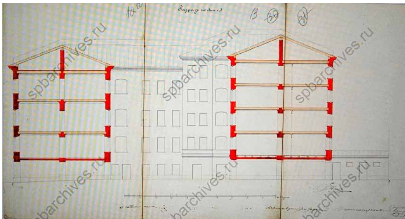
10. Разрез по линии с-д. Фасад южного дворового флигеля. 1858 г. Арх. Пель. ЦГИА СПб. Ф.513. Оп.102. Д.4684. Л.12-14.
