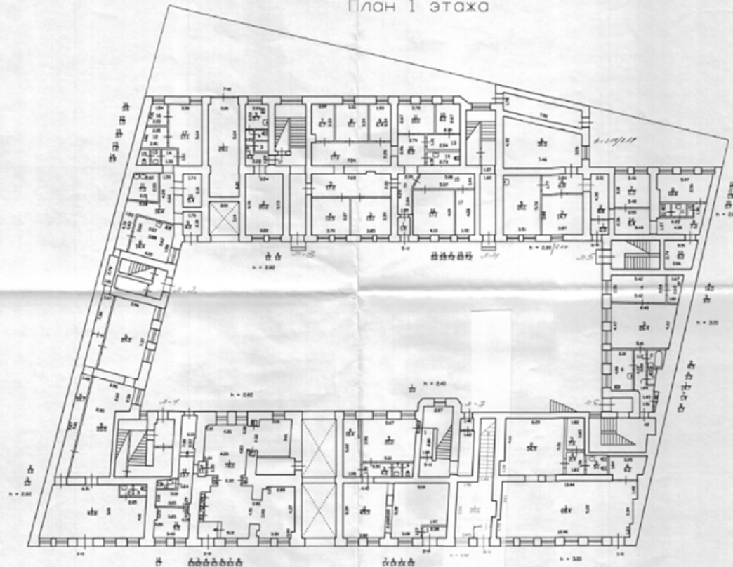
План 1 этажа
