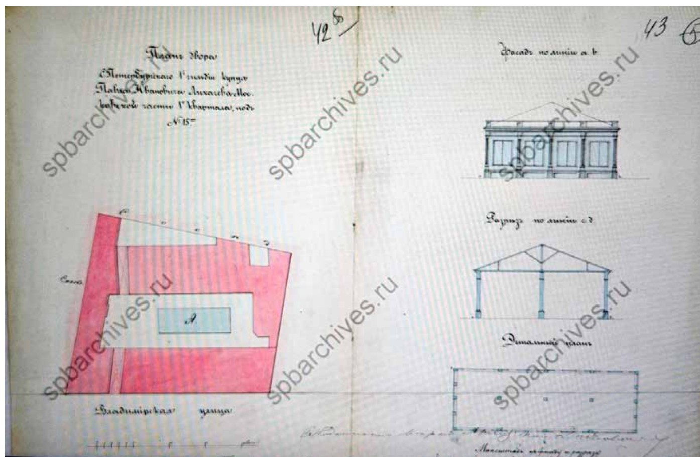
22. Генплан двора №3 по Владимирской ул., принадлежащего купцу Павлу Лихачеву с показанием под лит. А предполагаемого металлического сарая для дров, плен. 1866 г. ЦГИА СПб. Ф.513. Оп.102. Д.4684. Л.42-43.
