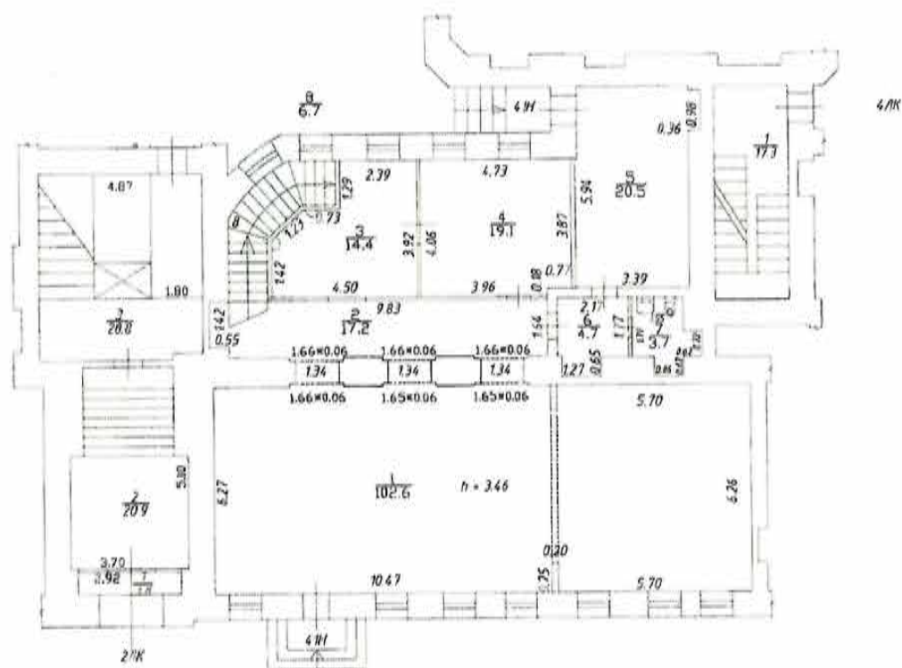
План части 1 этажа
