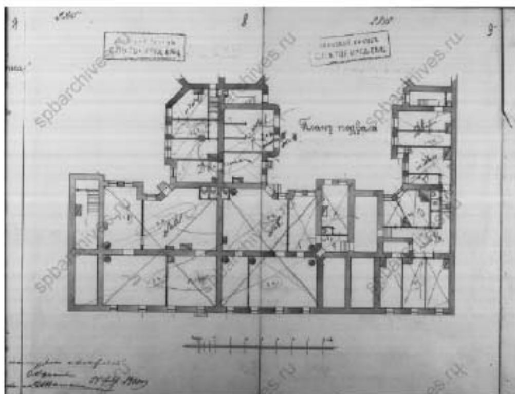
17. Дом Н.В. Чайковского по Надеждинской ул., 38 и Батарейному пер., 10 (совр. дом №36-38 по ул. Маяковского). Инвентаризационный чертеж. План подвала. 1910 г. // ЦГИА СПб. Ф. 515. Оп. 4. Д. 3663. Лл. 8-9.
