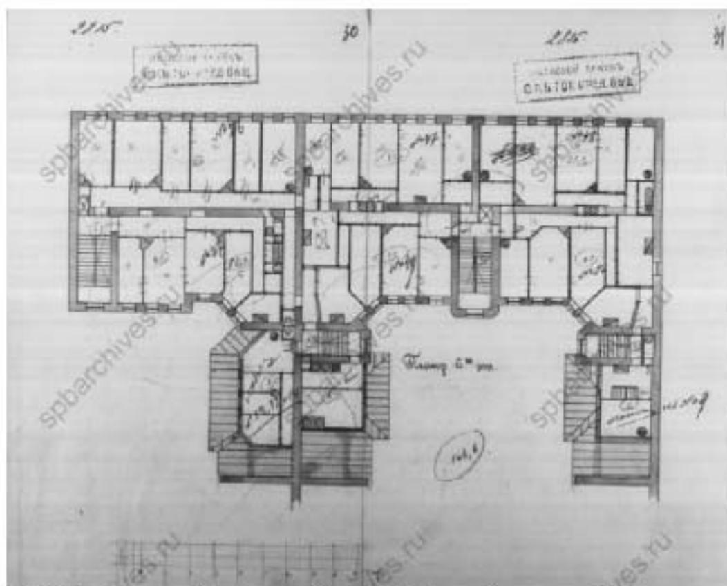
23. Дом Н.В. Чайковского по Надеждинской ул., 38 и Батарейному пер., 10 (совр. дом №36-38 по ул. Маяковского). Инвентаризационный чертёж. План 6-го этажа. 1910 г. // ЦГИА СПб. Ф. 515. Оп. 4. Д. 3663. Лл. 30-31.
