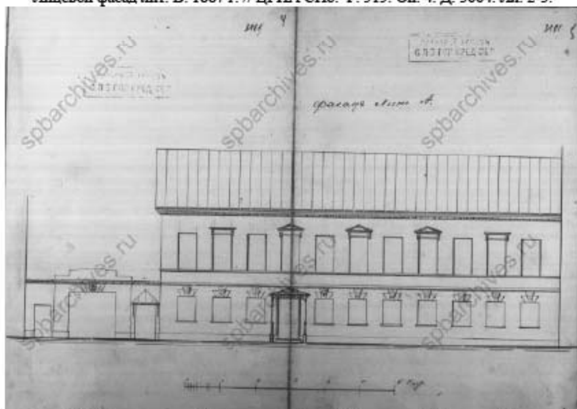
13. Дом купца В.С. Татаринова по Надеждинской ул., 32 (участок №38 по ул. Маяковского). Лицевой фасад лит. А. 1887 г. // ЦГИА СПб. Ф. 515. Оп. 4. Д. 3664. Лл. 4-5.
