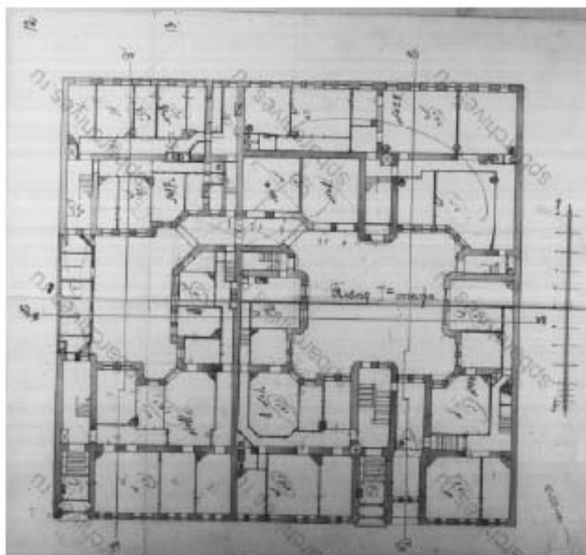
19. Дом Н.В. Чайковского по Надеждинской ул., 38 и Батарейному пер., 10 (совр. дом №36-38 по ул. Маяковского). Инвентаризационный чертеж. План 2-го этажа. 1910 г. // ЦГИА СПб. Ф. 515. Оп. 4. Д. 3663. Лл. 14-17.
