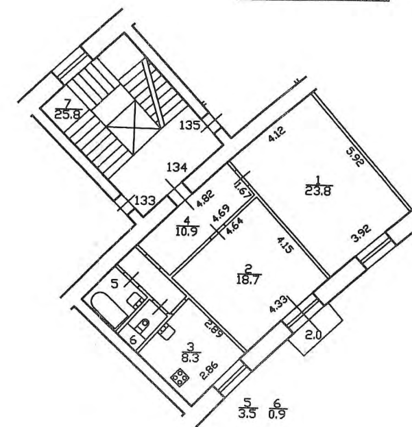
План 6 этажа
