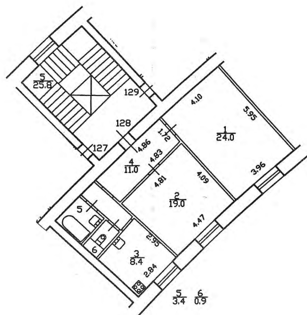
План 4 этажа
