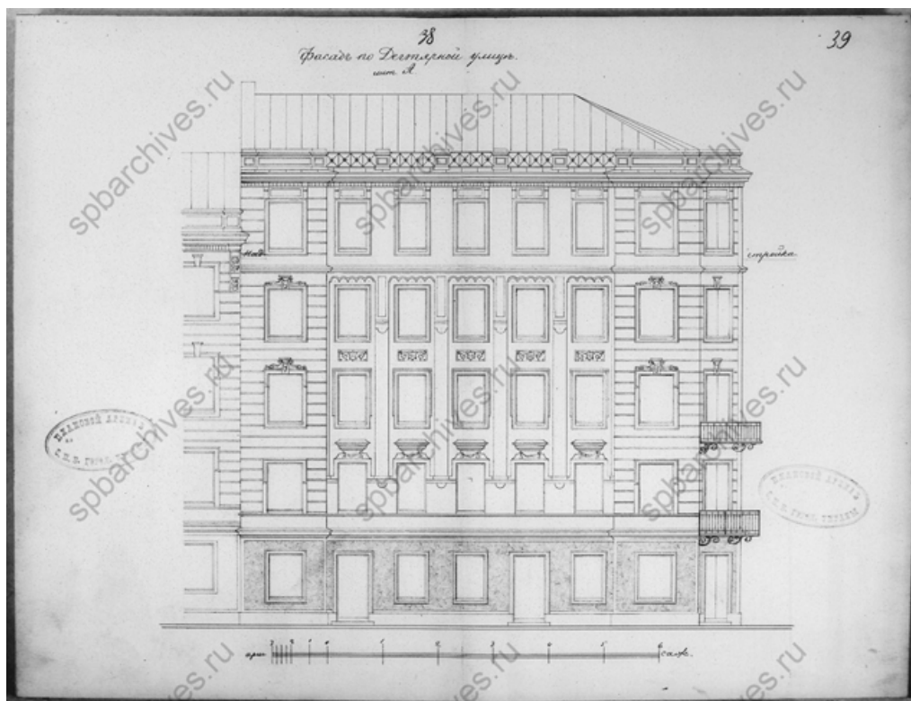
26. Фасад. ЦГИА СПб. Фонд 513. Описание 102. Дело 9468. Чертежи дома на участке, принадлежавшем Н.Д.Егорову, А.Д.Егорову, А.А.Аксенову по 9-й Рождественской ул., 22 и Дегтярной ул., 35-37.
