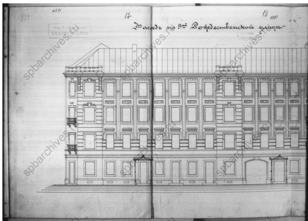
38. Фасад. ЦГИА СПб. Фонд 515. Опись 4. Дело 5190. Чертежи дома А.Д.Егорова, А.Н., Я.А. и А.А.Томиловых, А.А.Аксенова по 9-й Рождественской ул.,22 и Дегтярной ул.,35.
