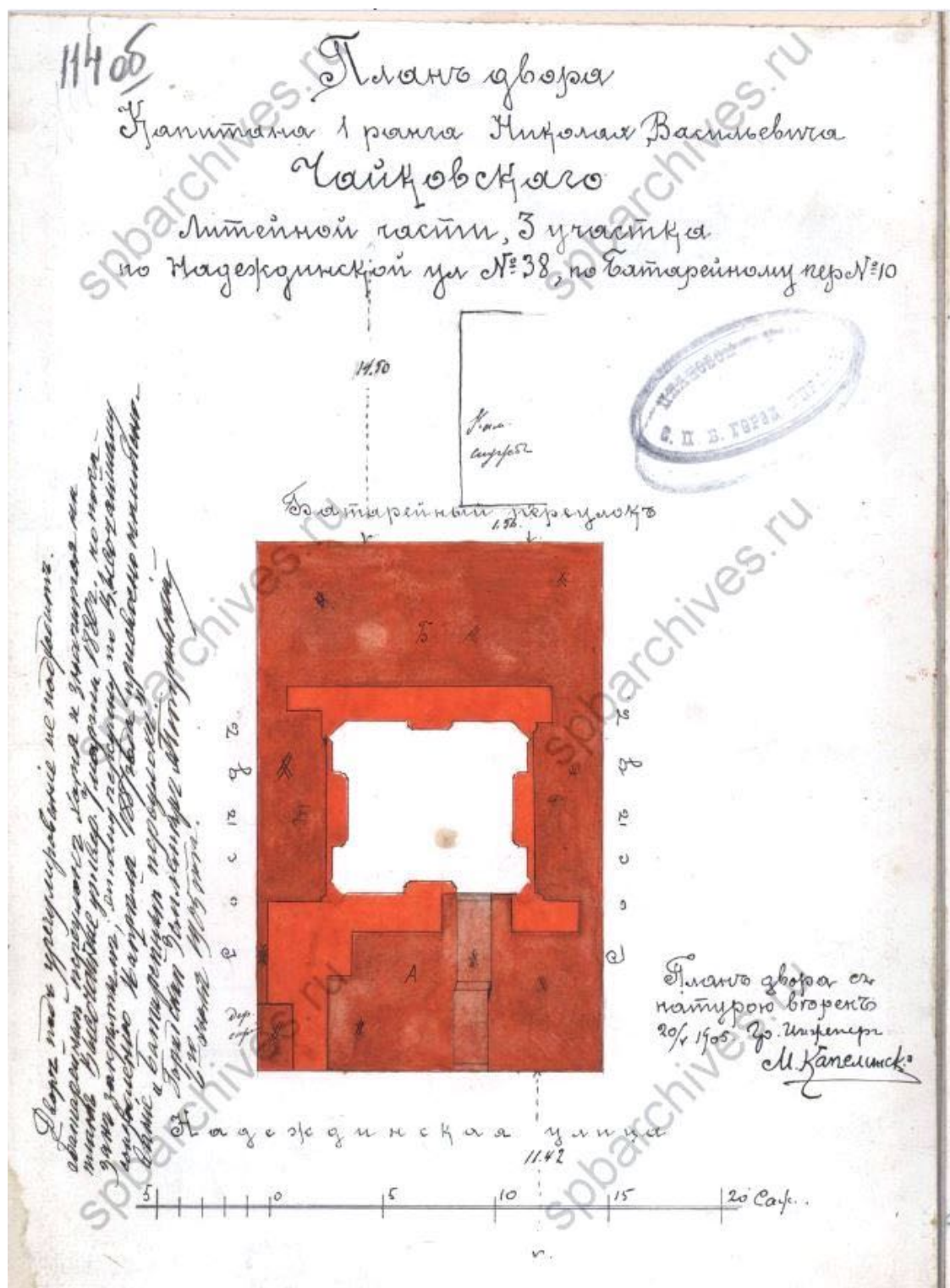
Илл. 26. План двора капитана 1 ранга Николая Васильевича Чайковского Литейной части, 3 участка по Надеждинской ул. № 38, по Батарейному пер. № 10. 1905 г. Гражданский инженер М. Капелинский. ЦГИА СПб. Ф. 513. Оп. 102. Д. 4306. Л. 114 об.
